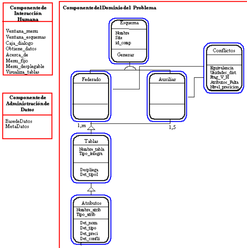
Clases Componentes de la Herramienta de Integración
