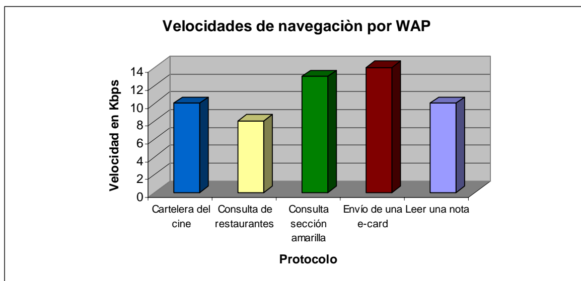
Figura 19: Velocidades de navegación por WAP
