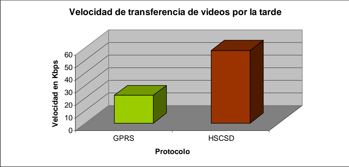
Figura 11: Velocidad de transferencia de videos por la tarde
