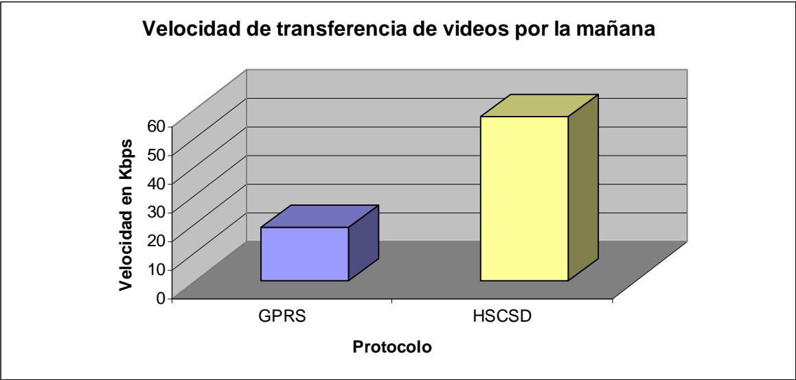
Figura 10: Velocidad de transferencia de videos por la mañana
