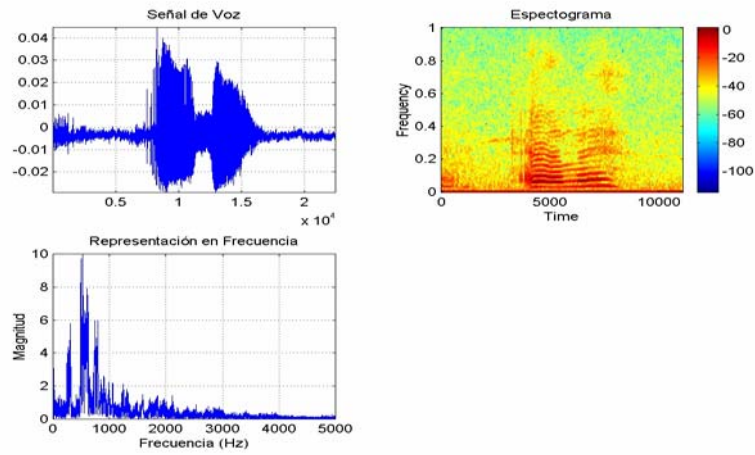
Figura A2.10 Letra M Pronunciación EME
