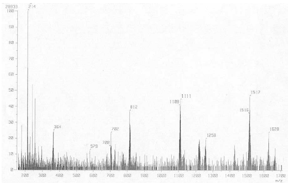
Figura C2. Complejo [Cd(C 14 H 10 NO 2 Cl 2 ) 2 •(MeOH)] 2
