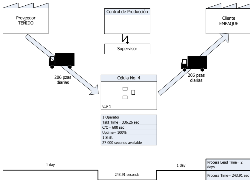
3. Mapa Futuro de la Célula de Manufactura No. 4
