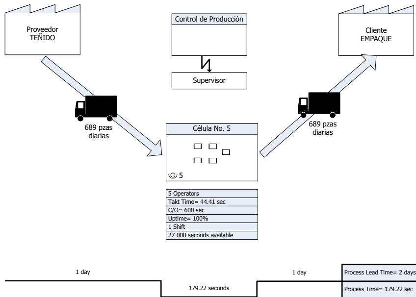
4. Mapa Futuro de la Célula de Manufactura No. 5
