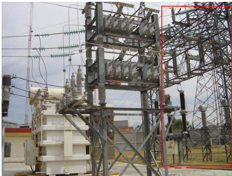
Figura A7 Banco de capacitores Puebla 2000
