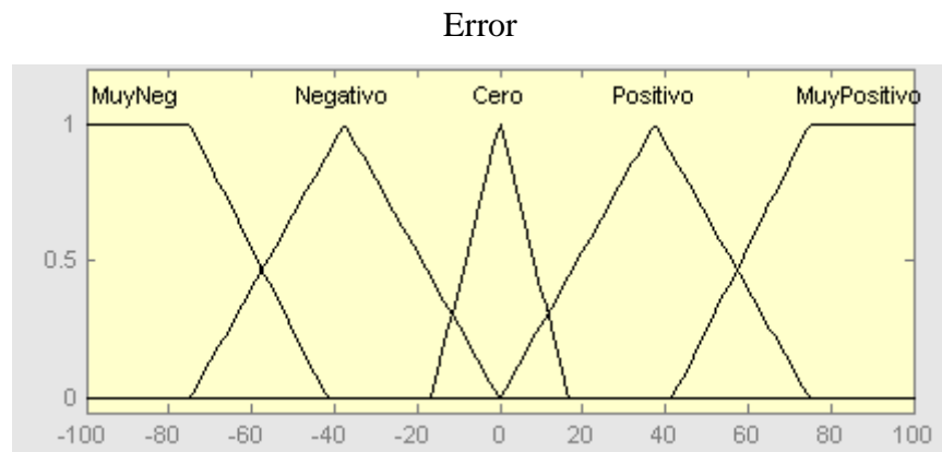
Figura A-1: Conjuntos difusos de la variable Error
