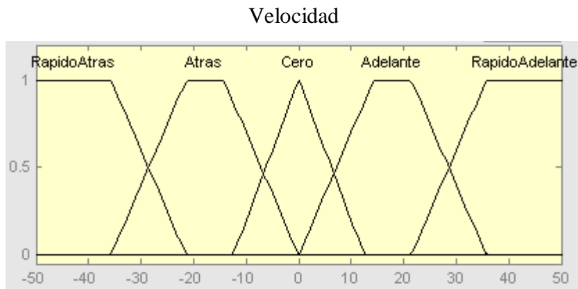
Figura A-8: Conjuntos difusos de la variable Velocidad
