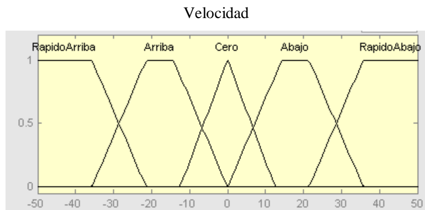
Figura A-2: Conjuntos difusos de la variable Velocidad
