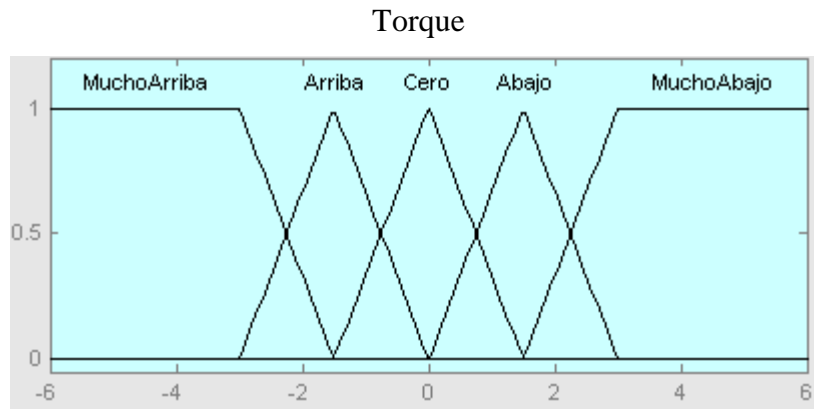
Figura A-3: Conjuntos difusos de la variable Torque
