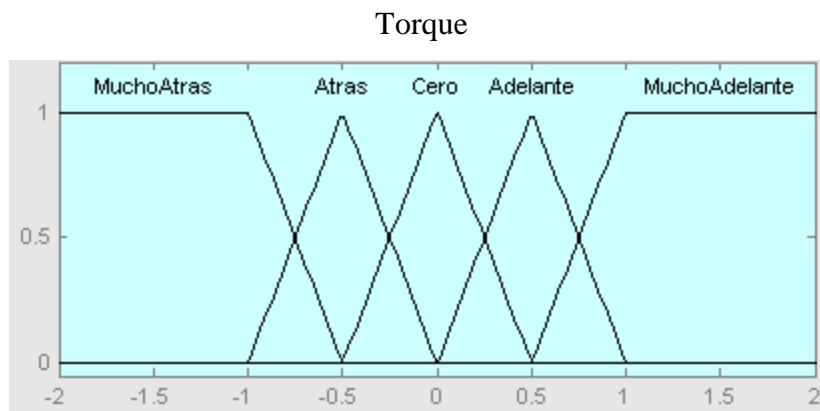
Figura A-6: Conjuntos difusos de la variable Torque
