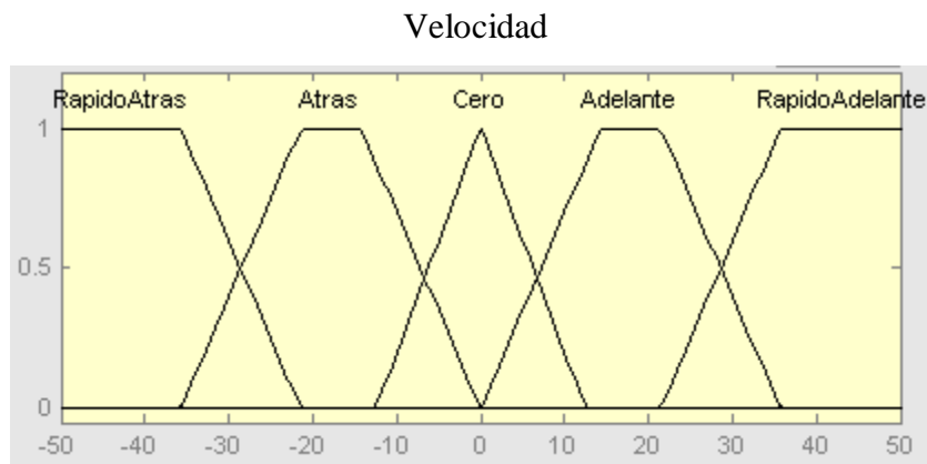
Figura A-5: Conjuntos difusos de la variable Velocidad
