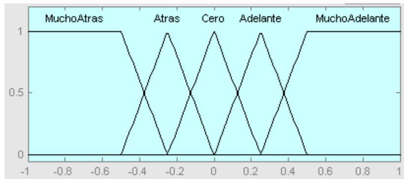
Figura A-9: Conjuntos difusos de la variable Torque
