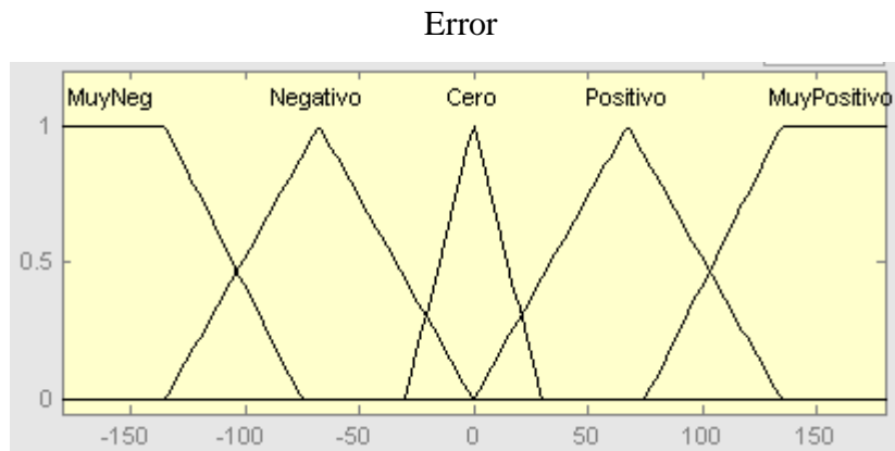
Figura A-7: Conjuntos difusos de la variable Error
