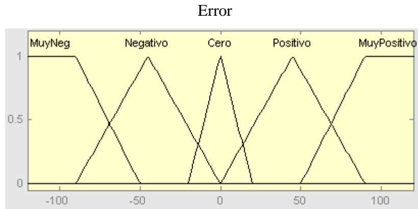
Figura A-4: Conjuntos difusos de la variable Error
