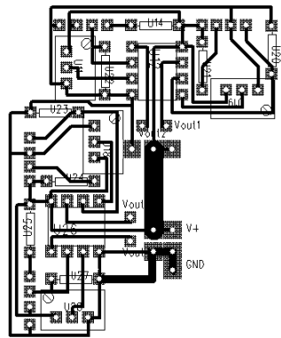
Circuito impreso para sensores de luz
