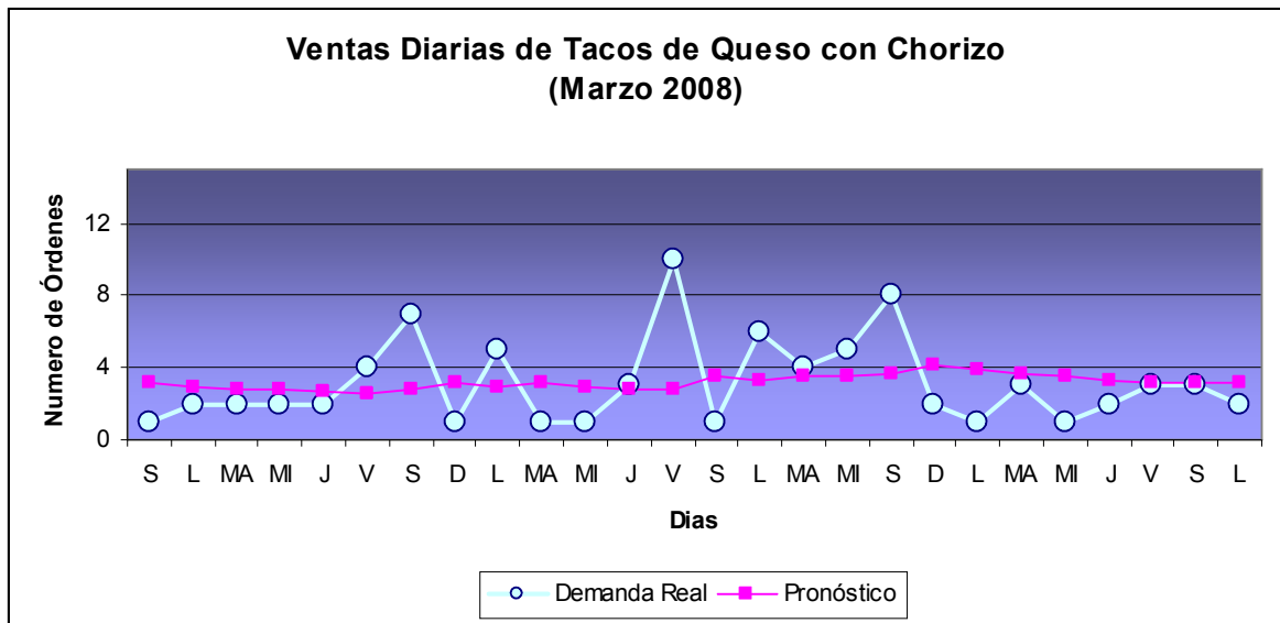
Figura A10.1 Ventas Diarias Reales vs. Pronosticadas de Tacos de Queso con Chorizo
