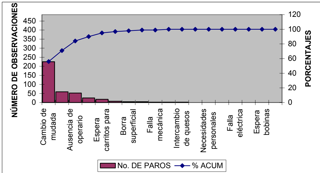
Diagrama de Pareto Continua Macías lado D
