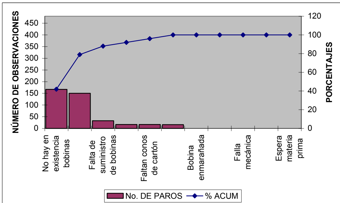
Diagrama de Pareto Conera lado B
