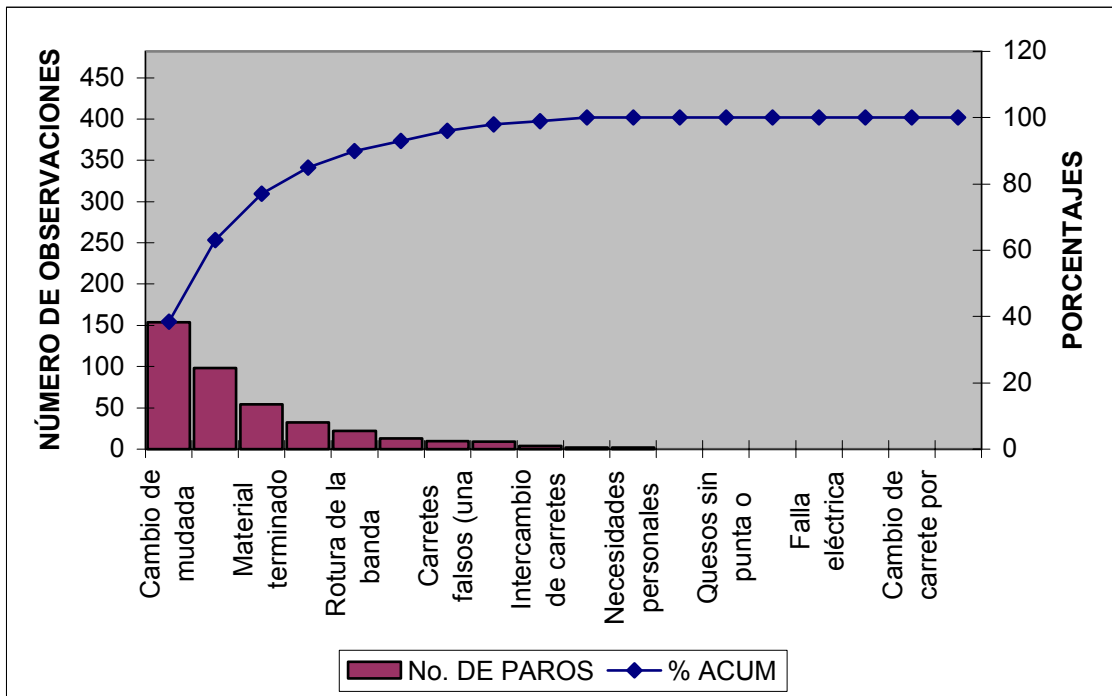
Diagrama de Pareto Continua Befama lado B
