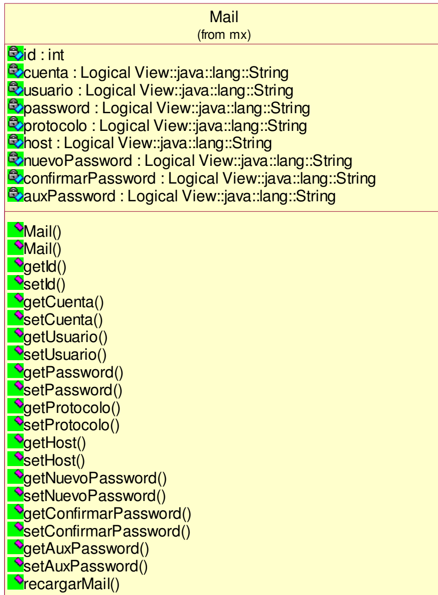
Clase Mail
