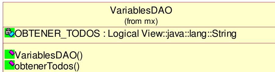
Clase VariablesDAO
