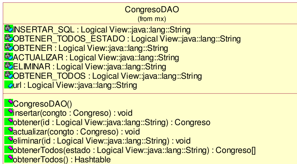
Clase CongresoDAO
