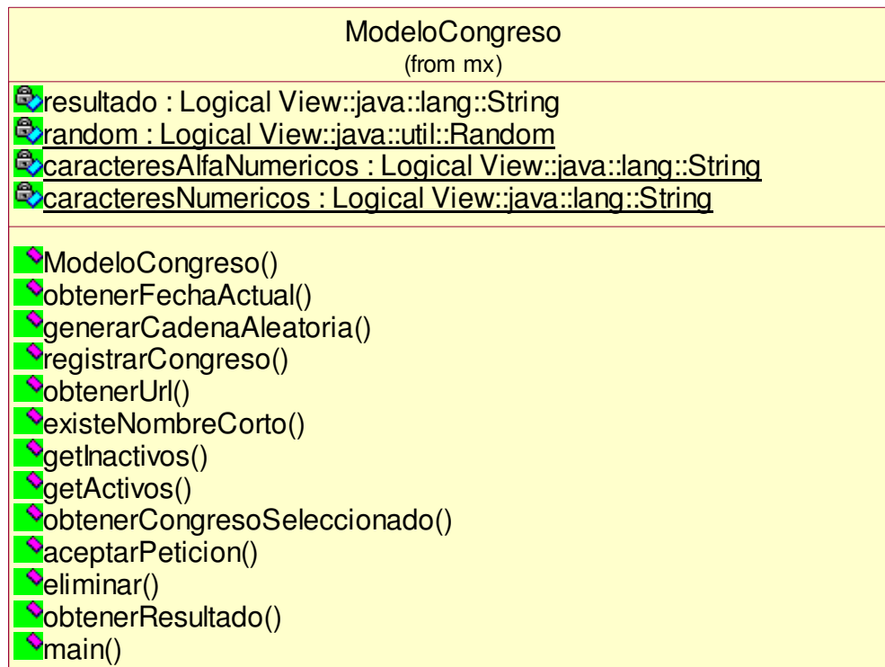
Clase ModeloCongreso
