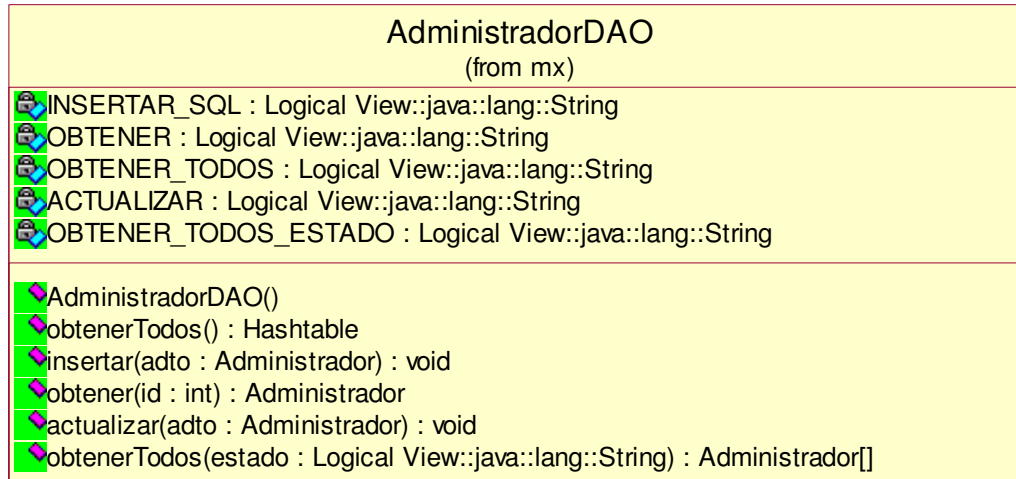
Clase AdministradorDAO
