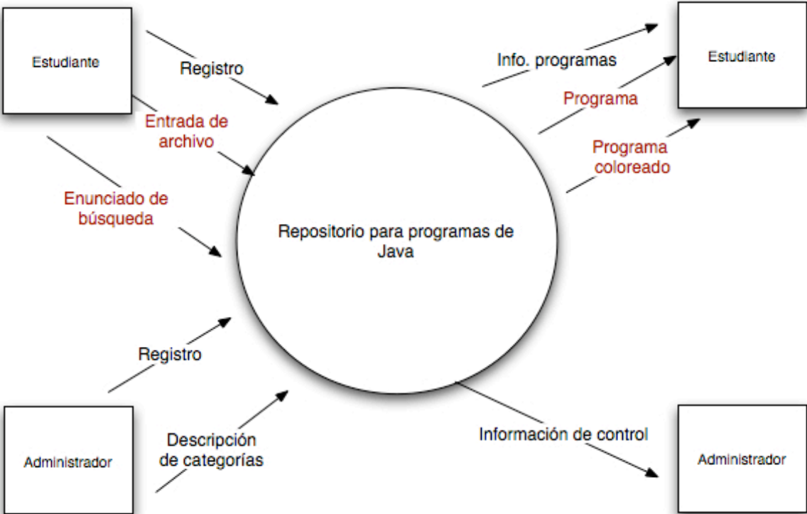
DFD de nivel contextual
