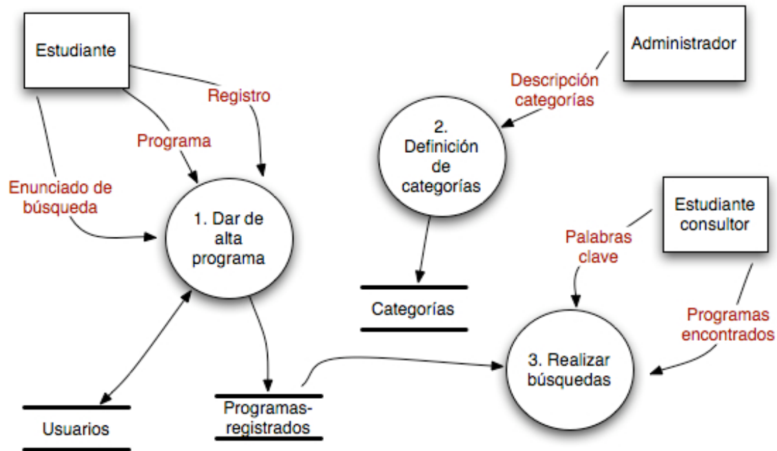
DFD nivel 1
