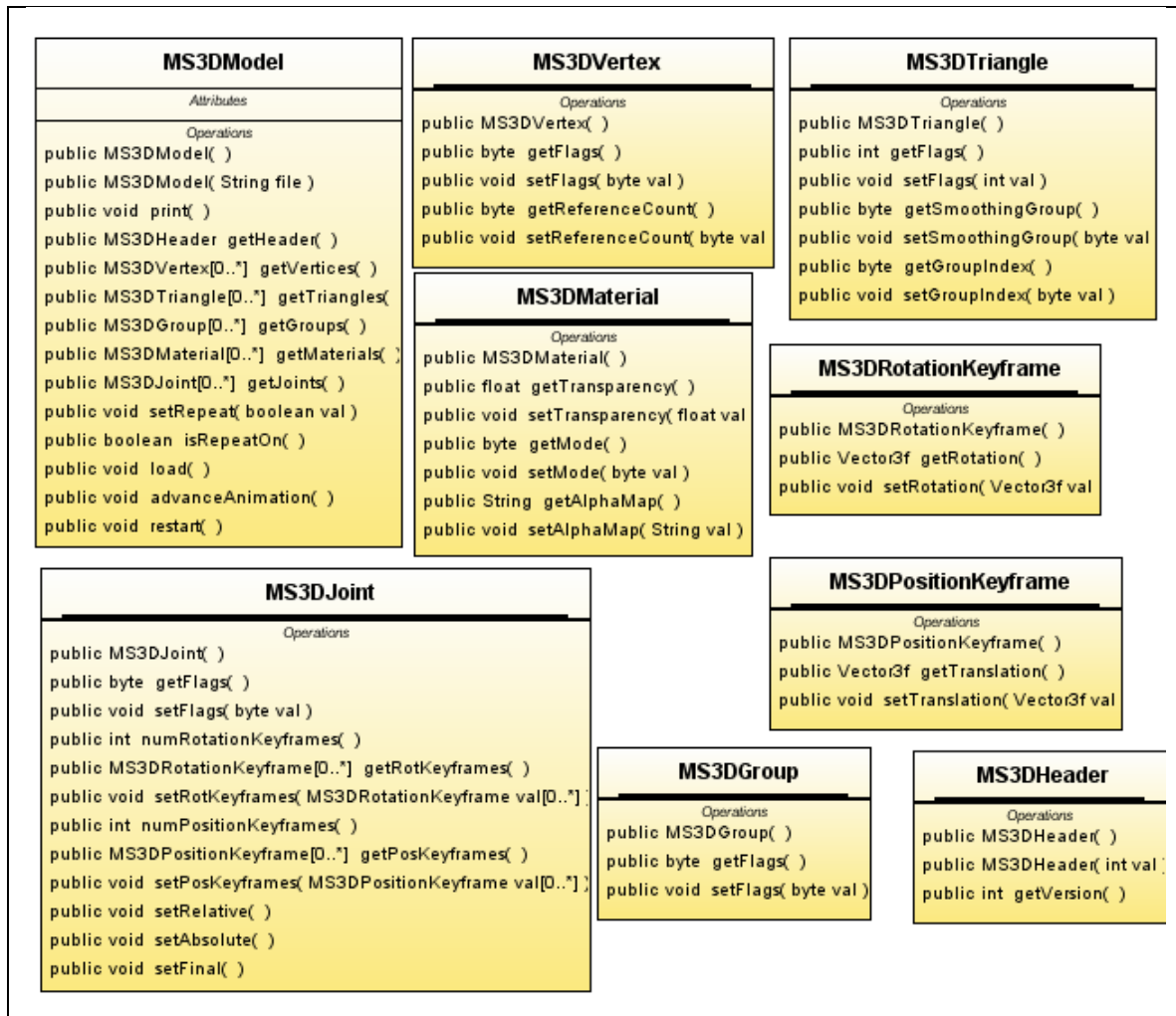
Figura C2: Clases de la especificación Milkshape 3D 1.8.0
