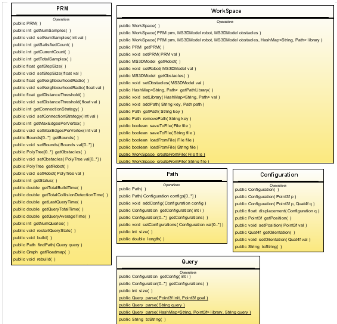
Figura C3: Clases para la planeación de rutas.
