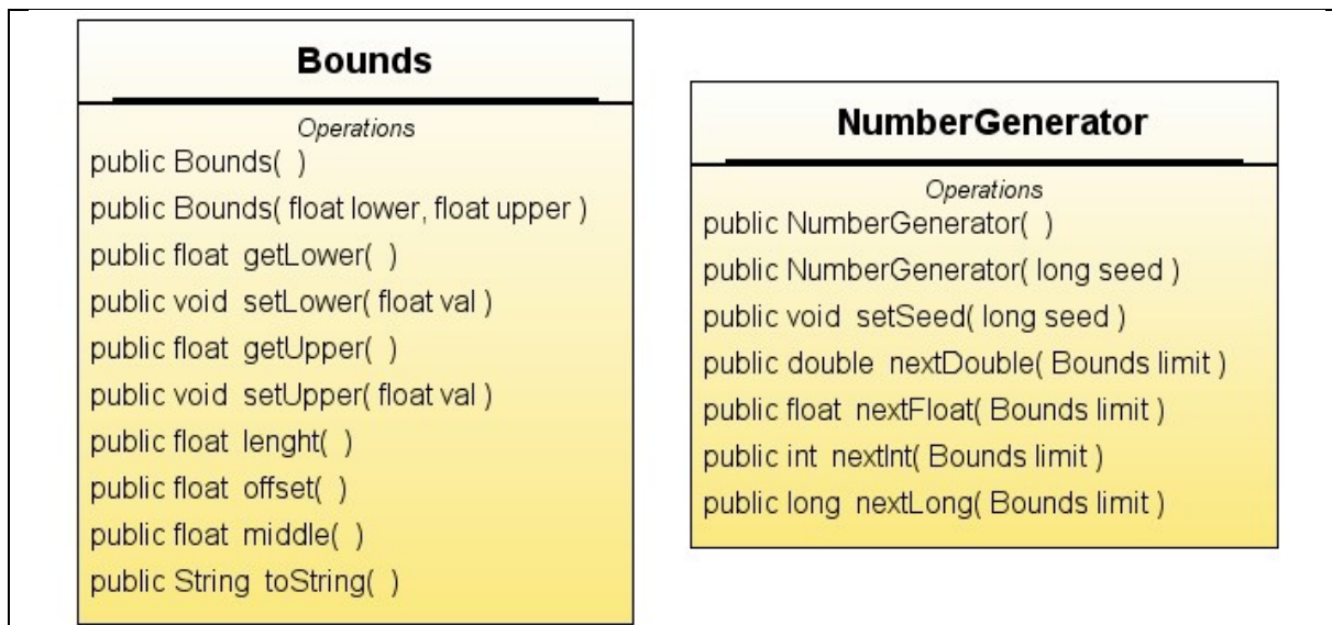
Figura C5: Clases auxiliares.
