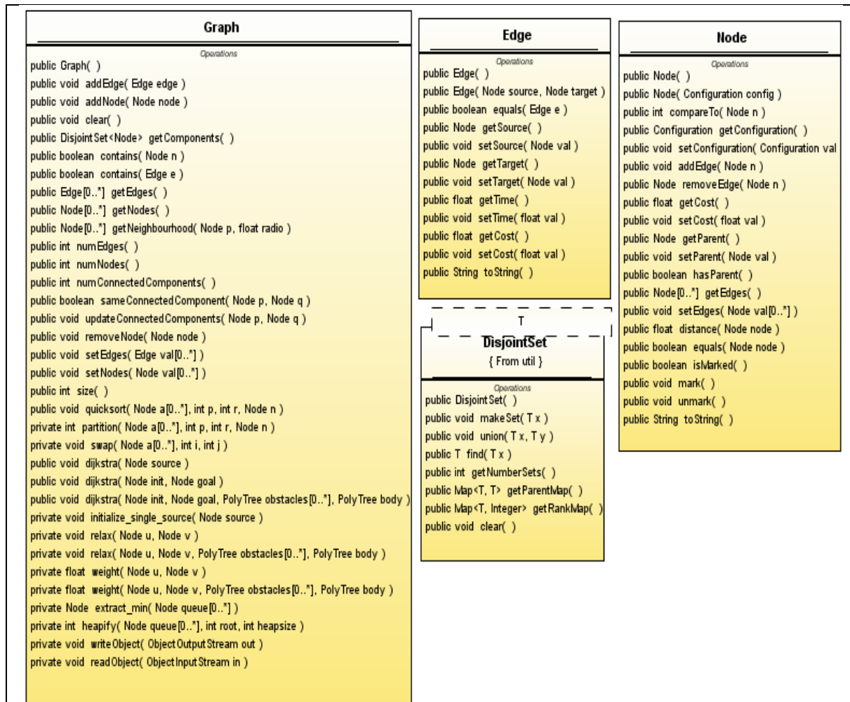
Figura C4: Clases para la representación del grafo.
