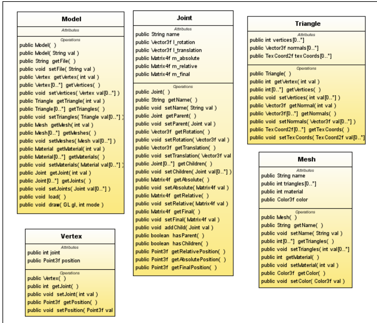
Figura C1: Clases para la representación de un modelo 3D.
