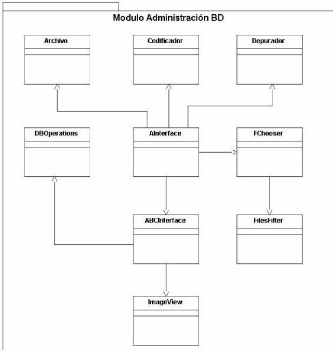
Figura A.1 Diagrama UML de clase del módulo de administración de la base de datos
