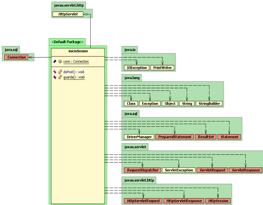
F.1 Diagrama clase inicioSesion.
