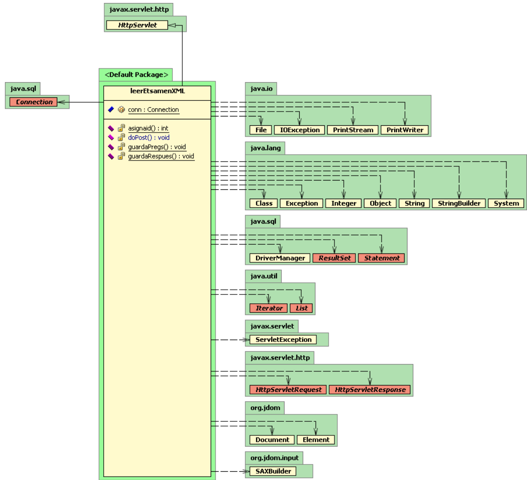
D.4 Diagrama de clase leerEtsamenXML.
