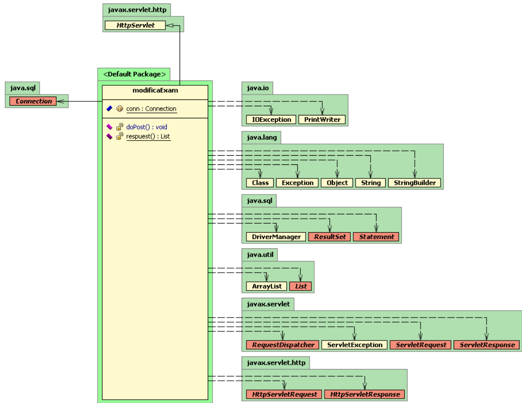
F.2 Diagrama de clase modificaExam.
