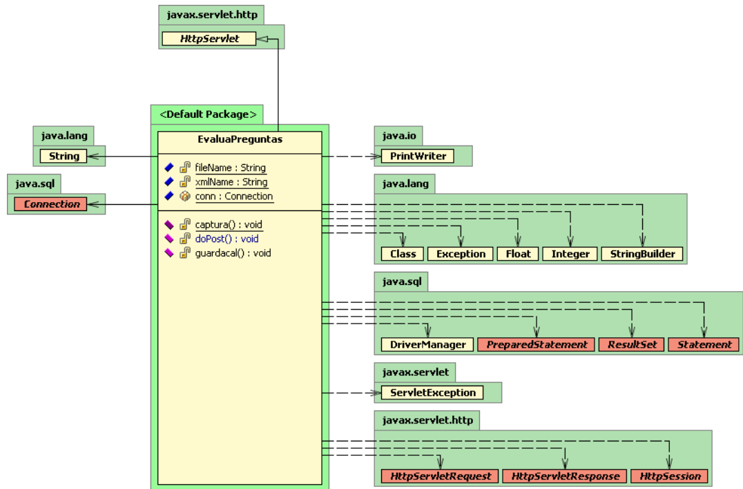
F.3 Diagrama de clase EvaluaPreguntas.
