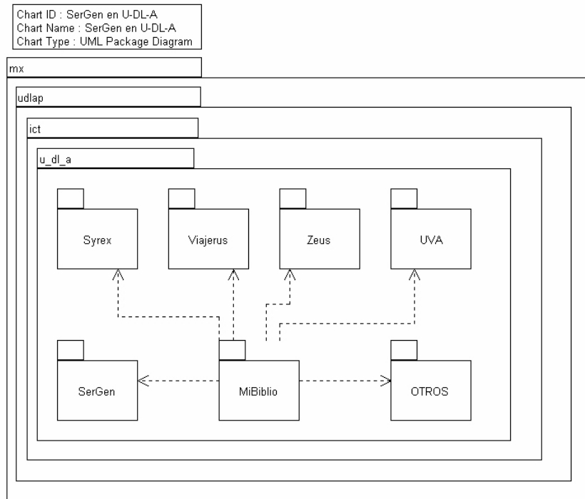
Figura A.1 SerGen en U-DL-A
