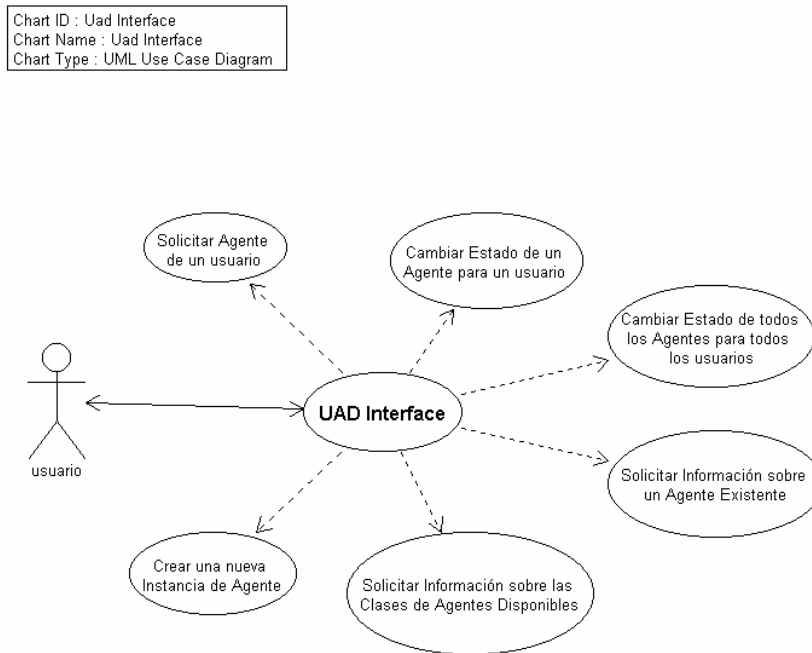
Figura A.4 Diagrama de casos de uso del UAD
