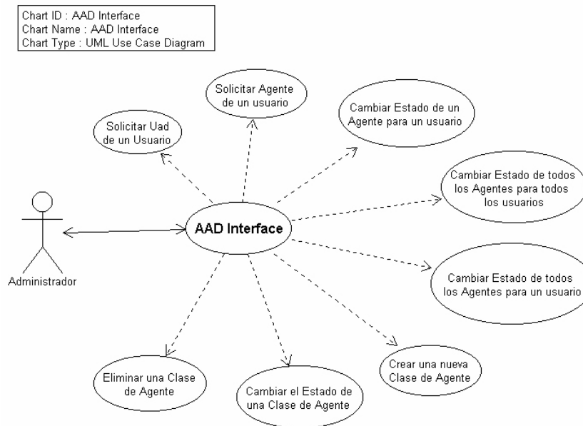
Figura A.5 Diagrama de casos de uso del AAD
