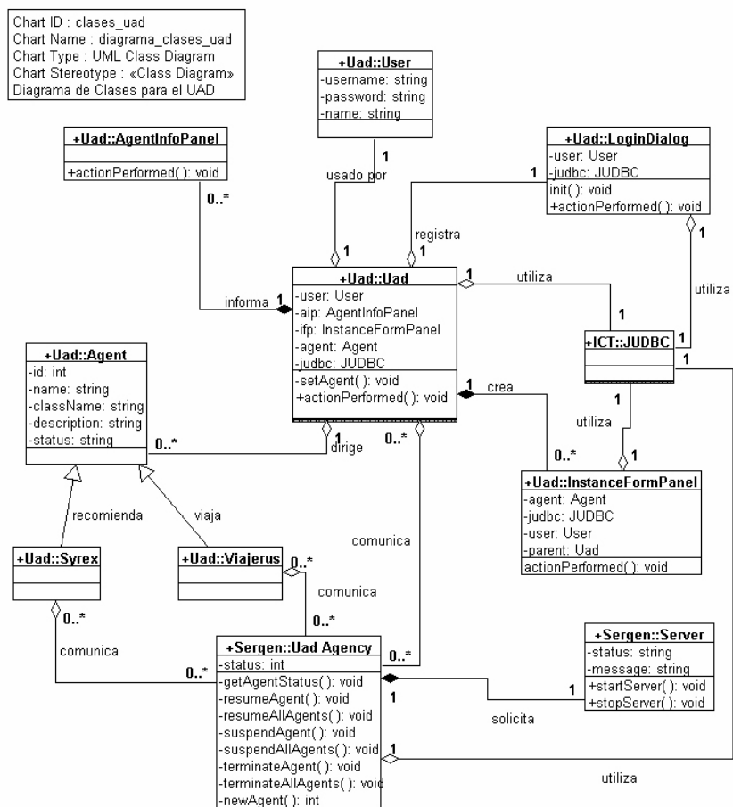
Figura A.3 Diagrama de Clases del UAD
