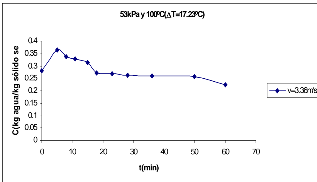
Figura E.10 Curva de secado de arroz.
