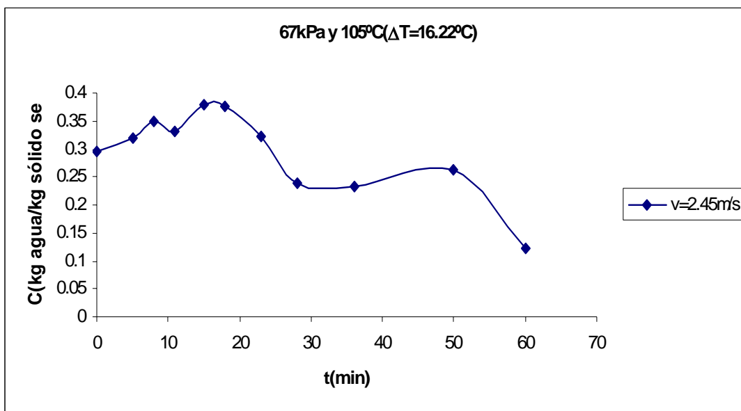
Figura E.25 Curva de secado de arroz.
