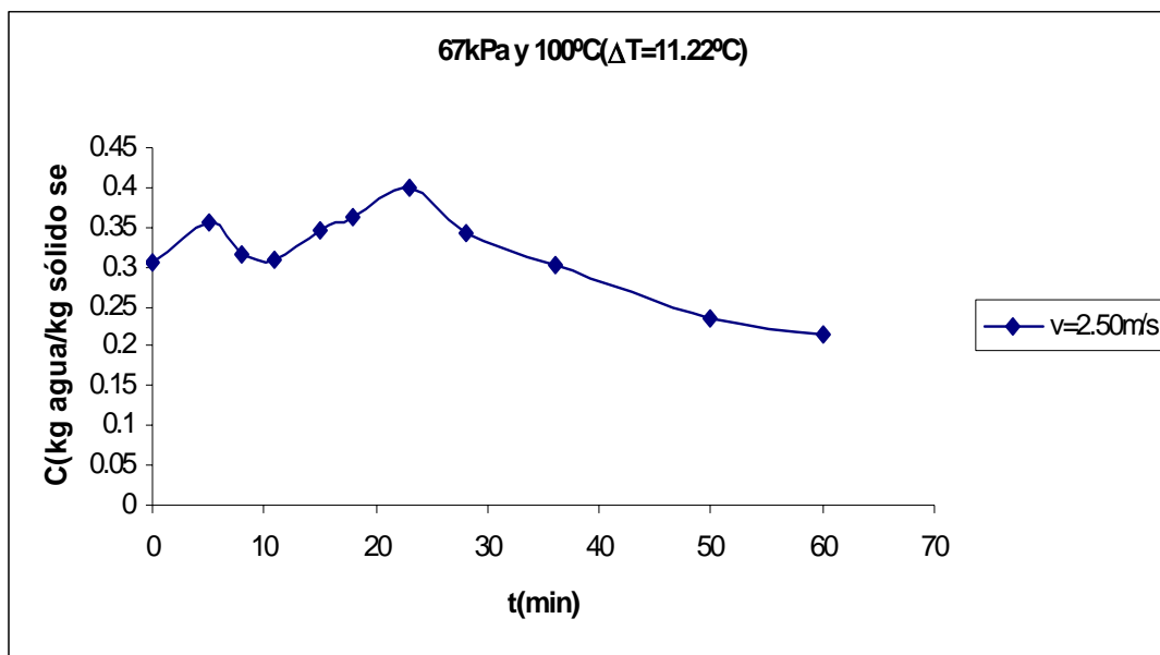
Figura E.19 Curva de secado de arroz.
