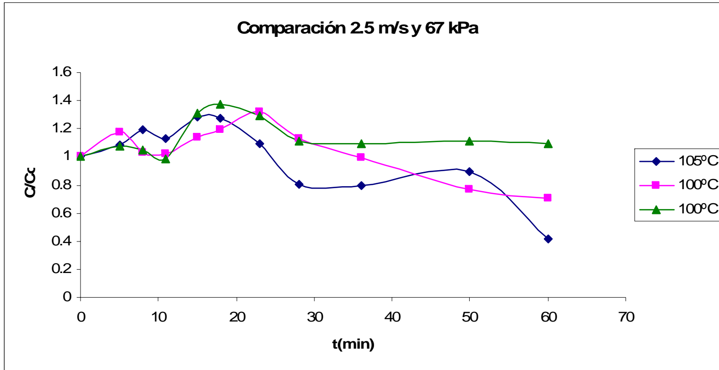
Figura E.26 Comparación de curvas normalizadas de secado.
