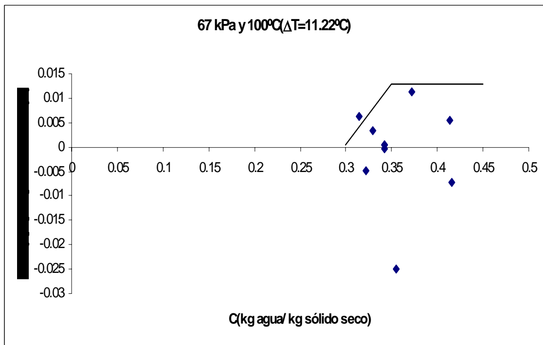
Figura E.24 Velocidad de secado de arroz v=2.51\text{ m/s} .
