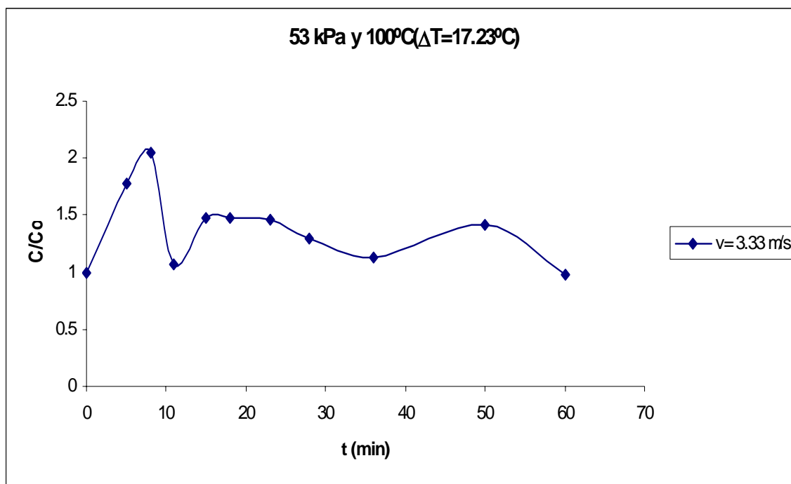
Figura E.5 Curva de secado de arroz.
