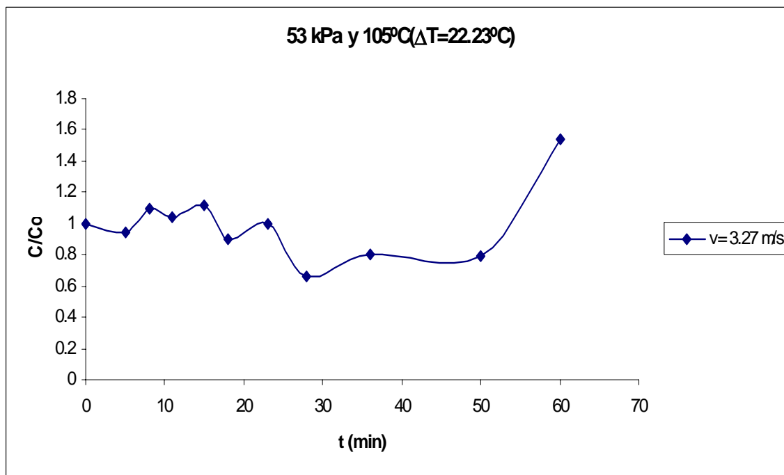
Figura E.14 Curva de secado de arroz.
