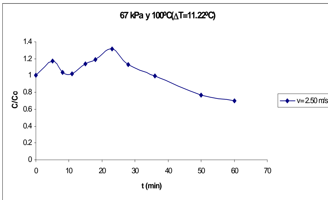
Figura E.20 Curva de secado de arroz.
