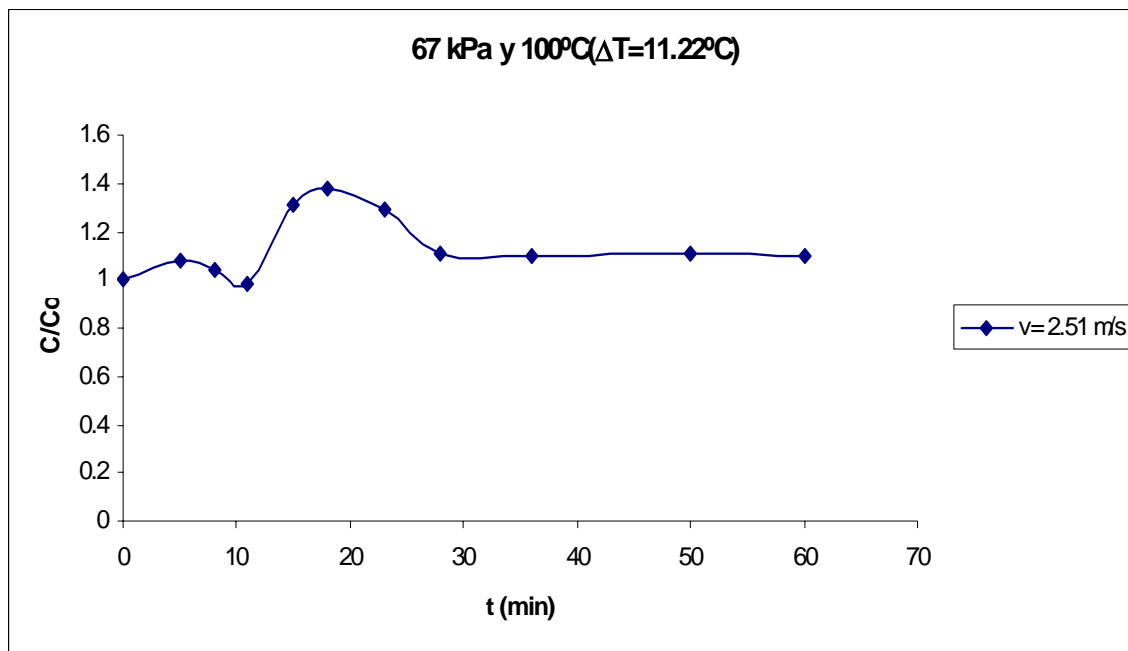
Figura E.23 Curva de secado de arroz.
