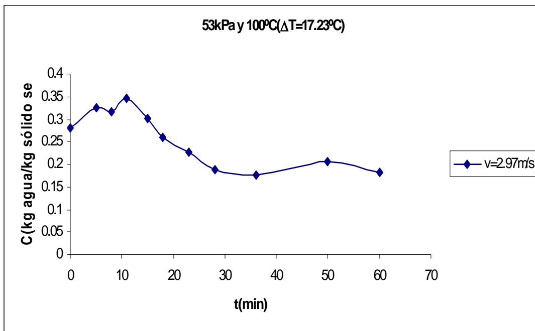
Figura E.1 Curva de secado de arroz.
