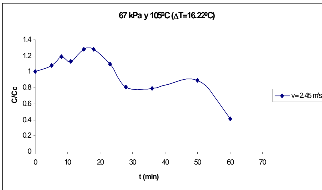
Figura E.26 Curva de secado de arroz.
