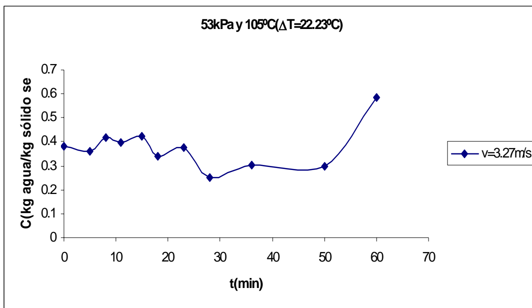
Figura E.13 Curva de secado de arroz.
