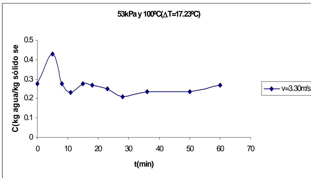
Figura E.7 Curva de secado de arroz.
