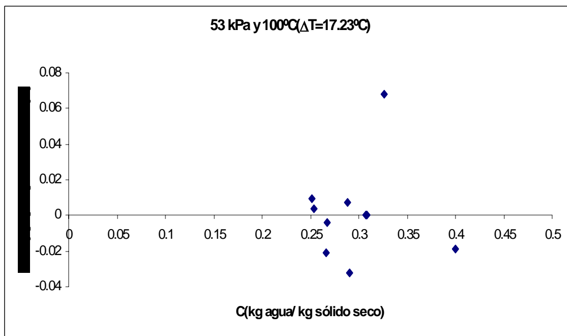
Figura E.6 Velocidad de secado de arroz v=2.97 m/s.
