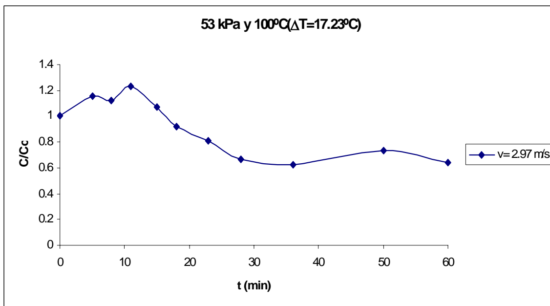
Figura E.2 Curva de secado de arroz.
