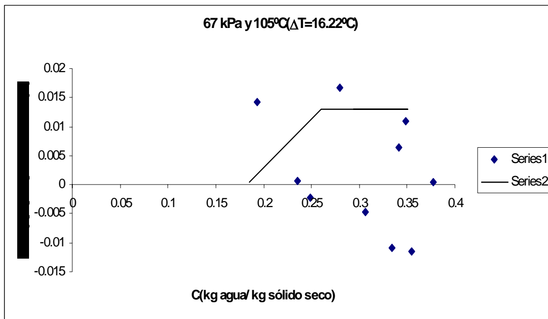
Figura E.24 Velocidad de secado de arroz v=2.45 m/s.
