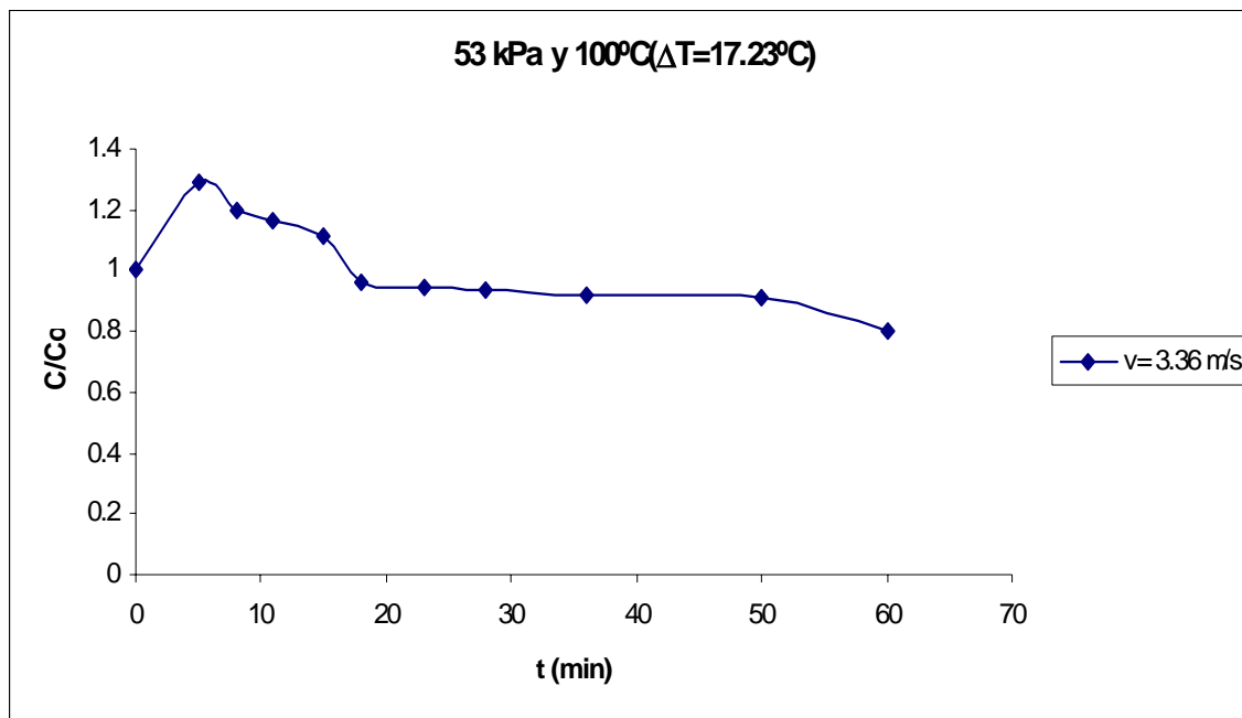
Figura E.11 Curva de secado de arroz.
