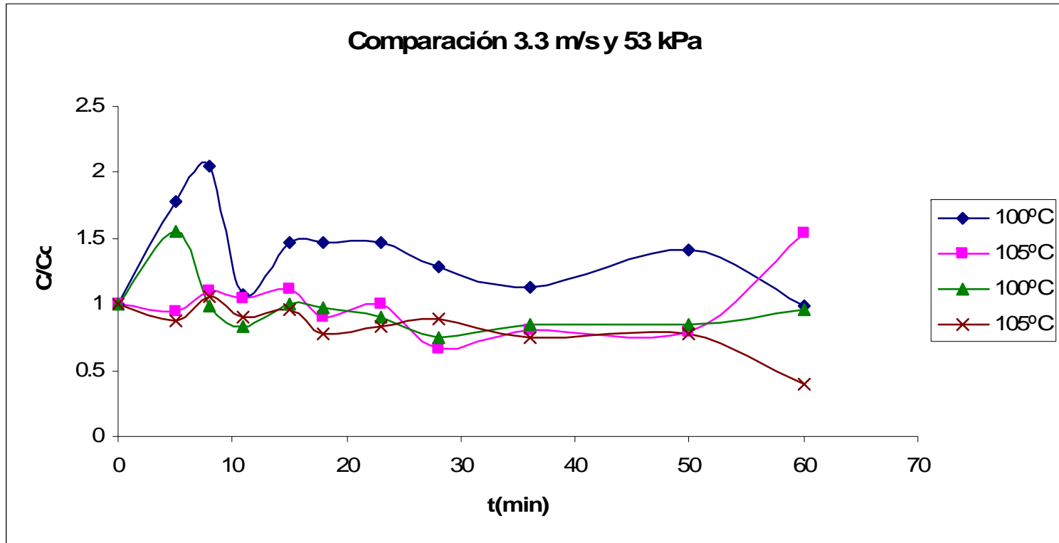
Figura E.25 Comparación de curvas normalizadas de secado.
