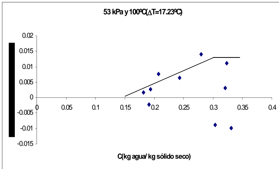
Figura E.3 Velocidad de secado de arroz v=2.97 m/s.
