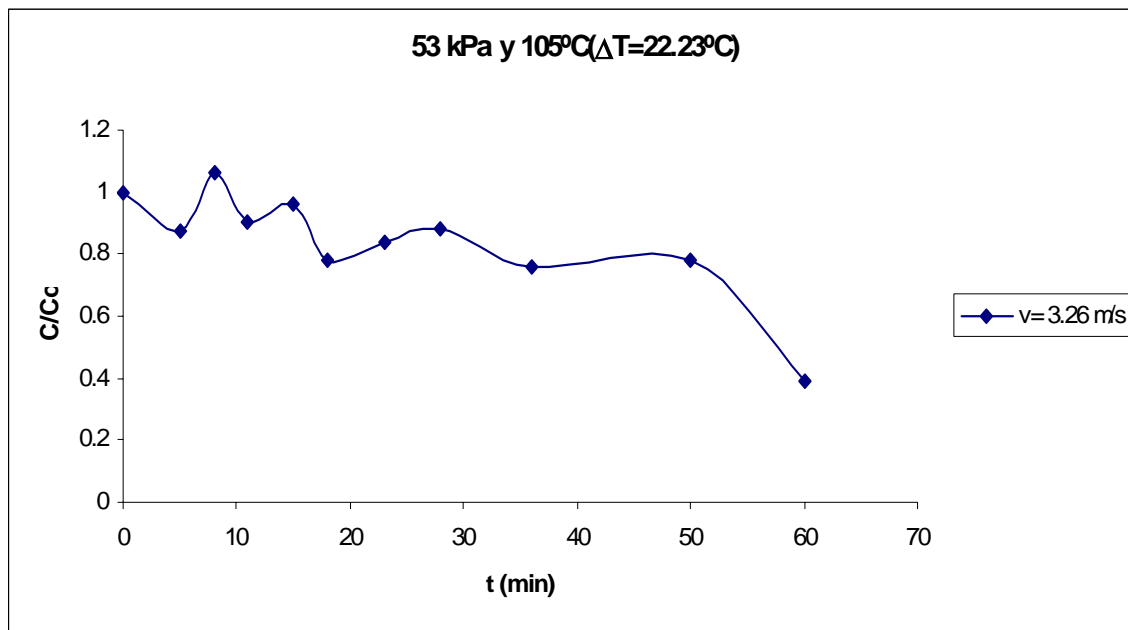
Figura E.17 Curva de secado de arroz.
