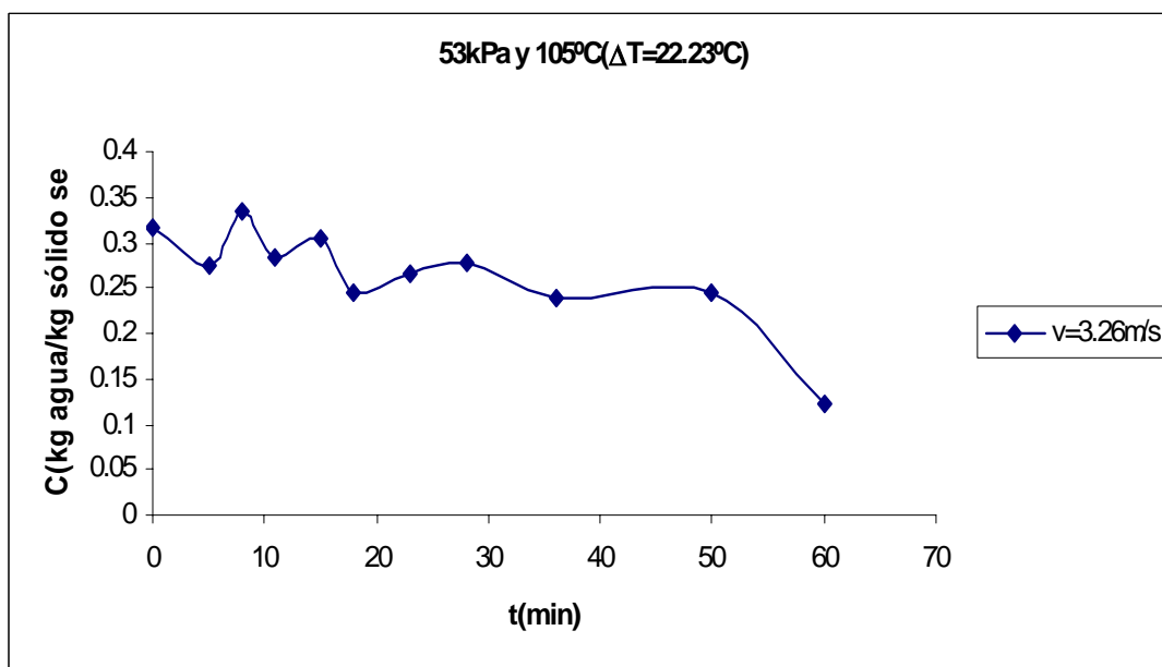
Figura E.16 Curva de secado de arroz.
