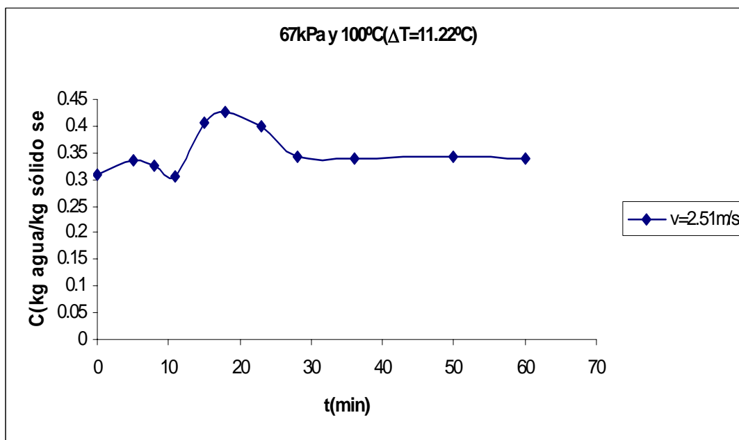
Figura E.22 Curva de secado de arroz.
