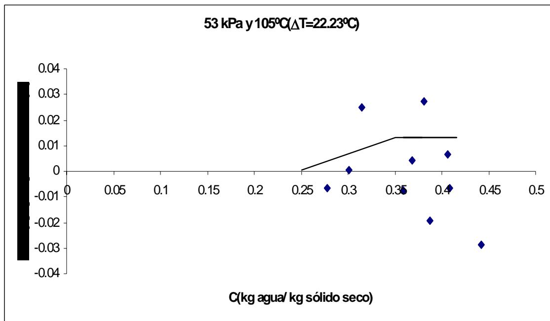
Figura E.15 Velocidad de secado de arroz v=3.27 m/s.
