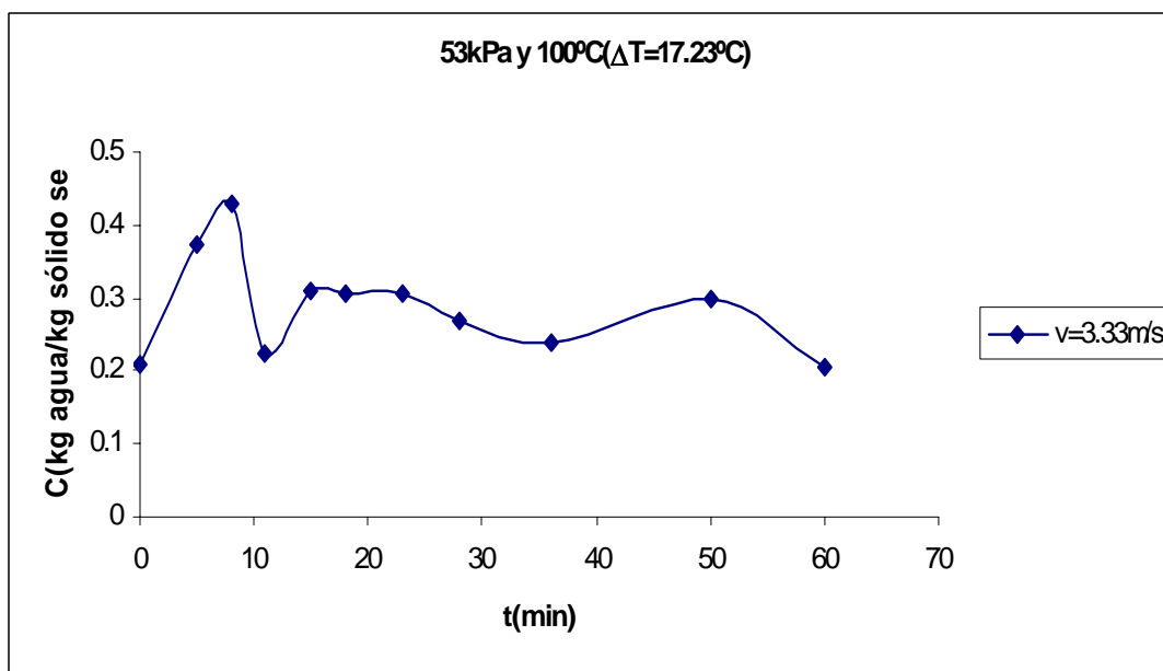
Figura E.4 Curva de secado de arroz.
