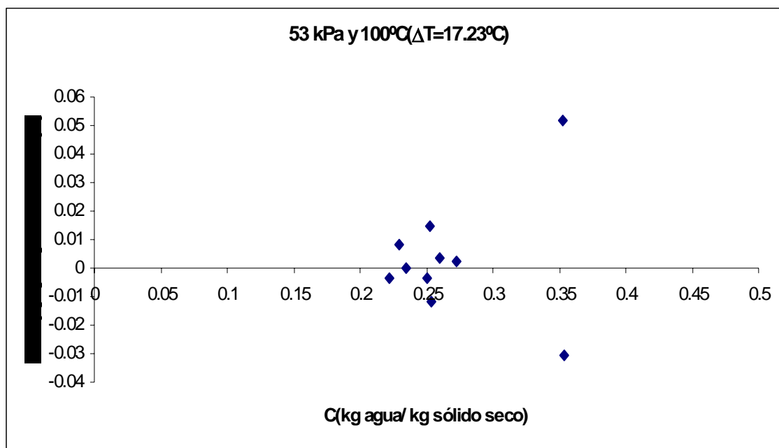
Figura E.9 Velocidad de secado de arroz v = 3.30 m/s.
