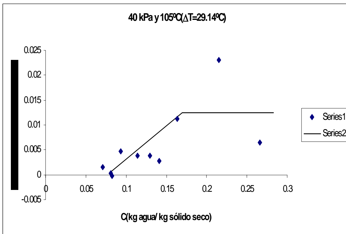
Figura C.6 Velocidad de secado de arroz con cáscara v=2.90 m/s.
