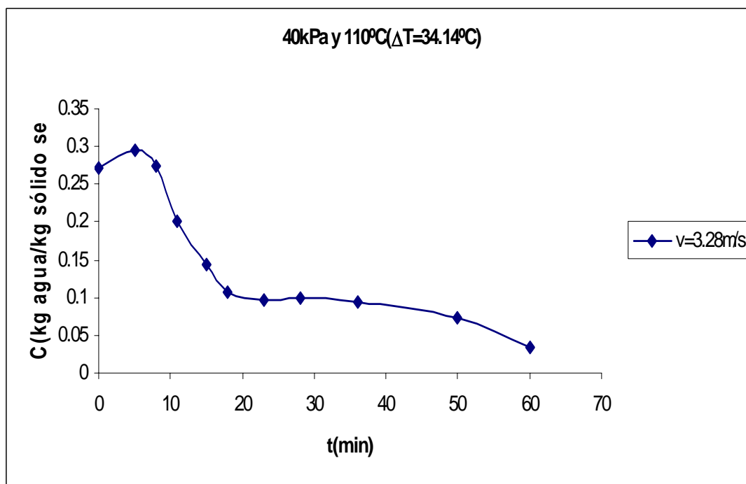
Figura C.16 Curva de secado de arroz con cáscara.
