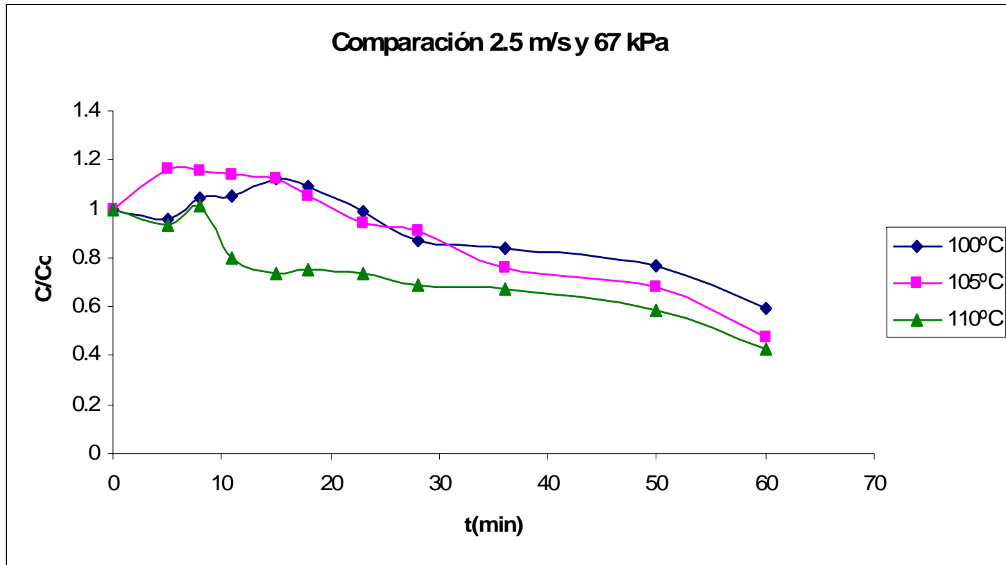
Figura C.79 Comparación de curvas normalizadas de secado.
