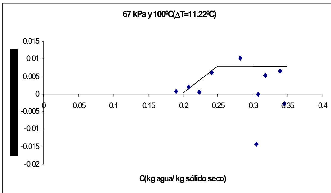
Figura C.51 Velocidad de secado de arroz con cáscara v=2.32 m/s.
