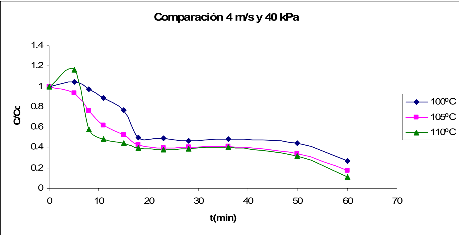
Figura C.75 Comparación de curvas normalizadas de secado.
