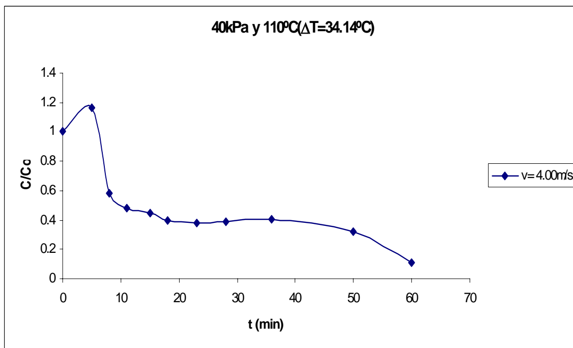
Figura C.26 Curva de secado de arroz con cáscara.
