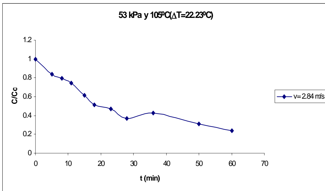
Figura C.32 Curva de secado de arroz con cáscara.
