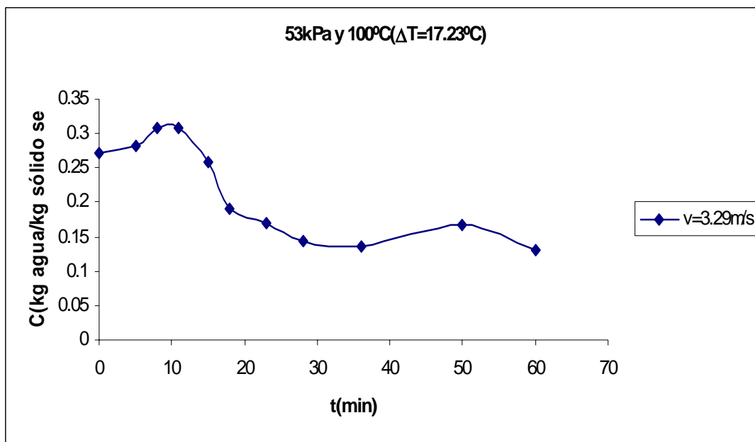
Figura C.37 Curva de secado de arroz con cáscara.
