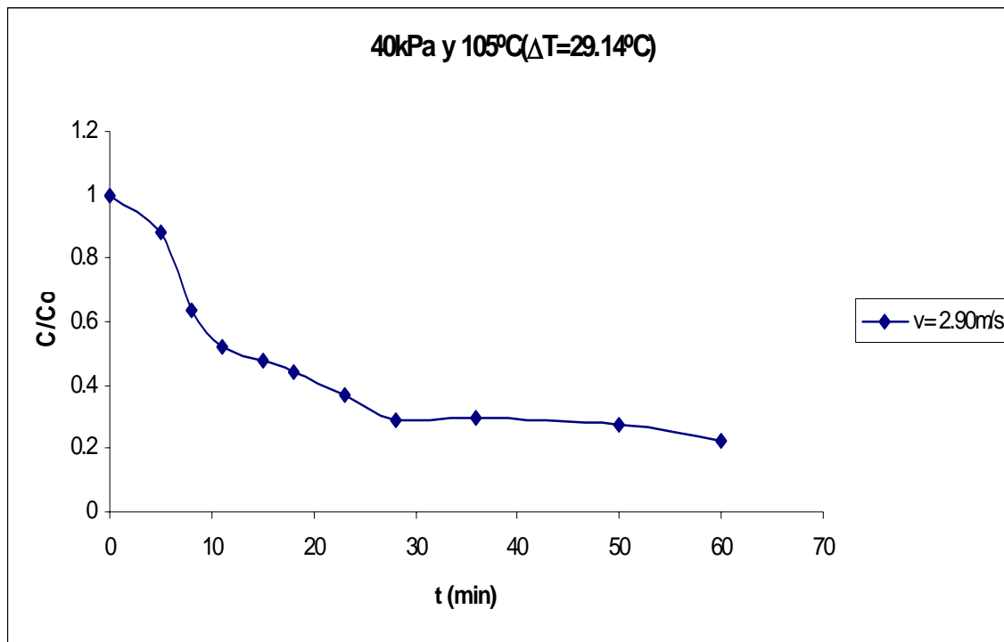
Figura C.5 Curva de secado de arroz con cáscara.
