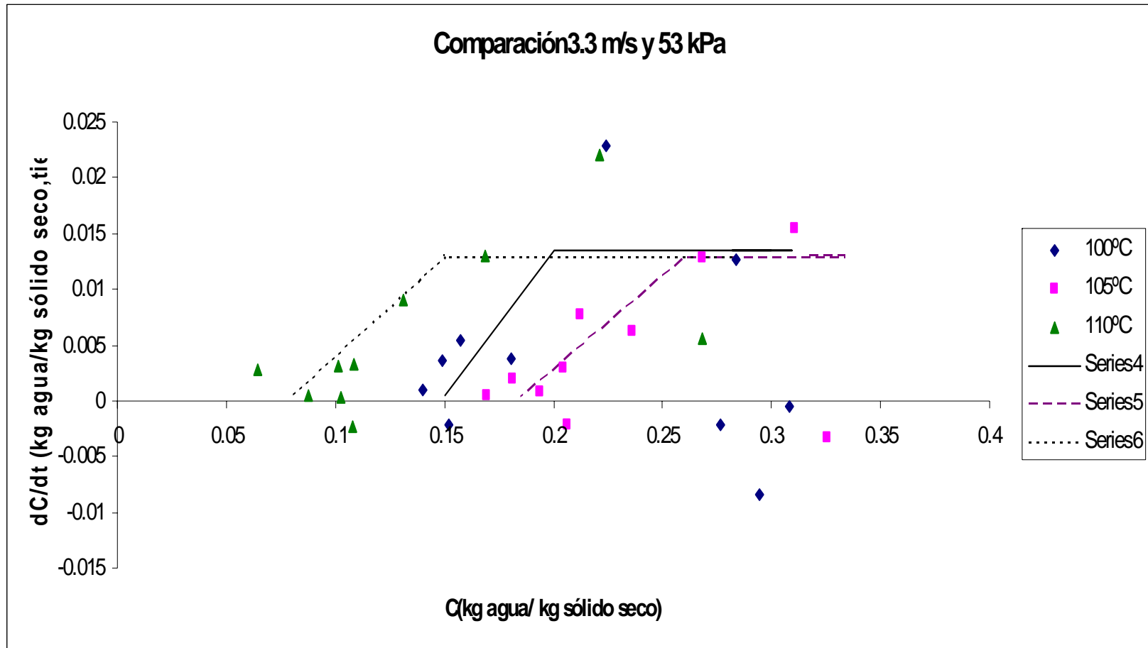
Figura C.90 Comparación de velocidades de secado.
