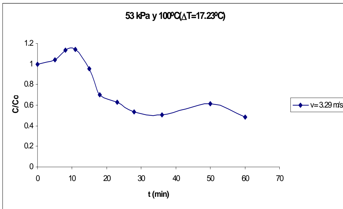
Figura C.38 Curva de secado de arroz con cáscara.
