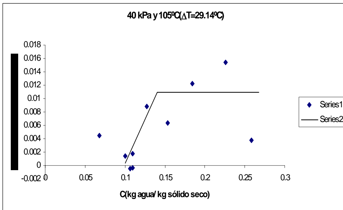
Figura C.24 Velocidad de secado de arroz con cáscara v=4.07 m/s.
