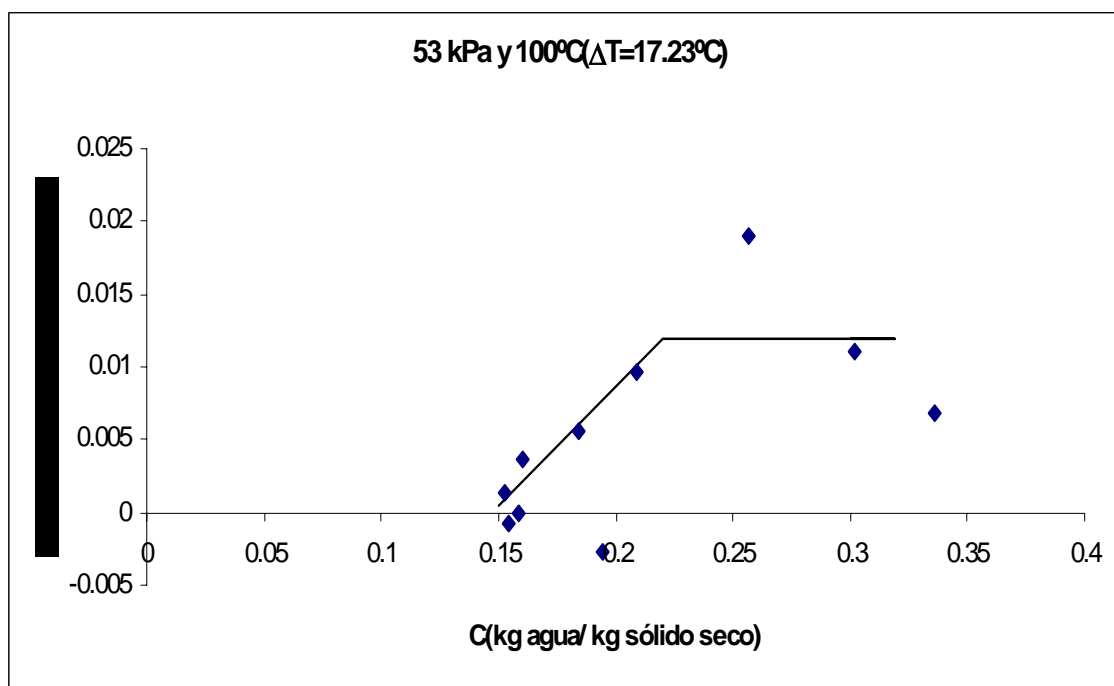
Figura C.30 Velocidad de secado de arroz con cáscara v=2.98\text{ m/s} .
