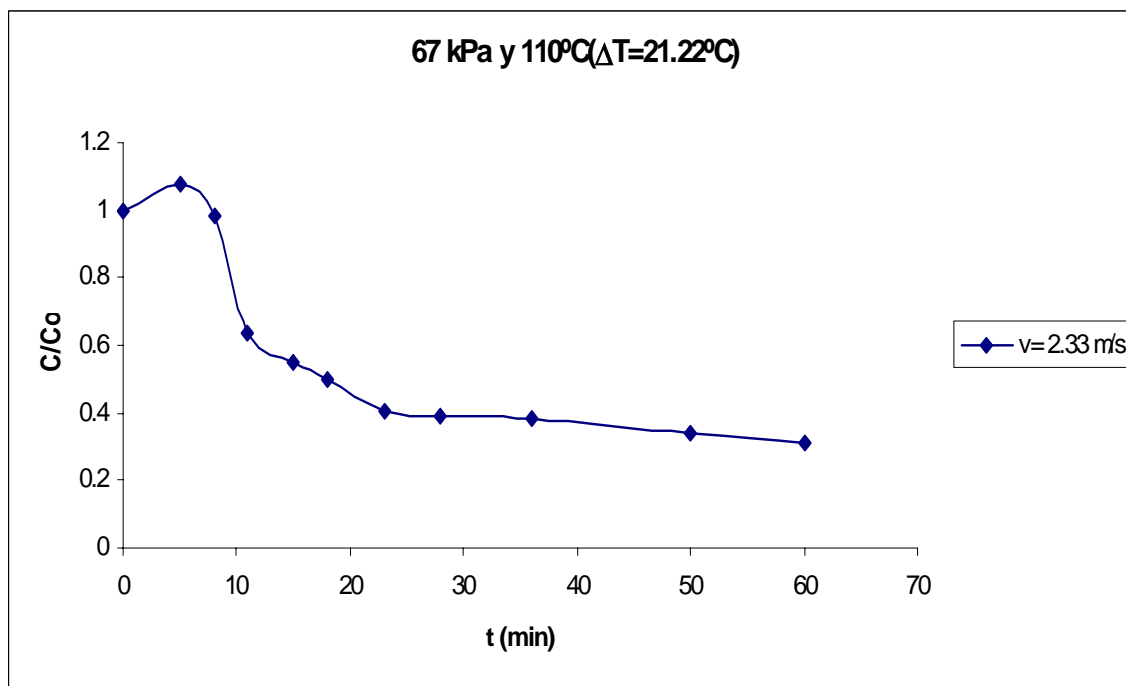
Figura C.56 Curva de secado de arroz con cáscara.
