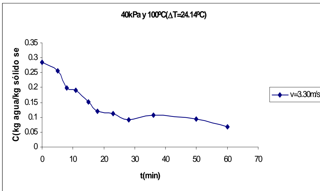
Figura C.10 Curva de secado de arroz con cáscara.
