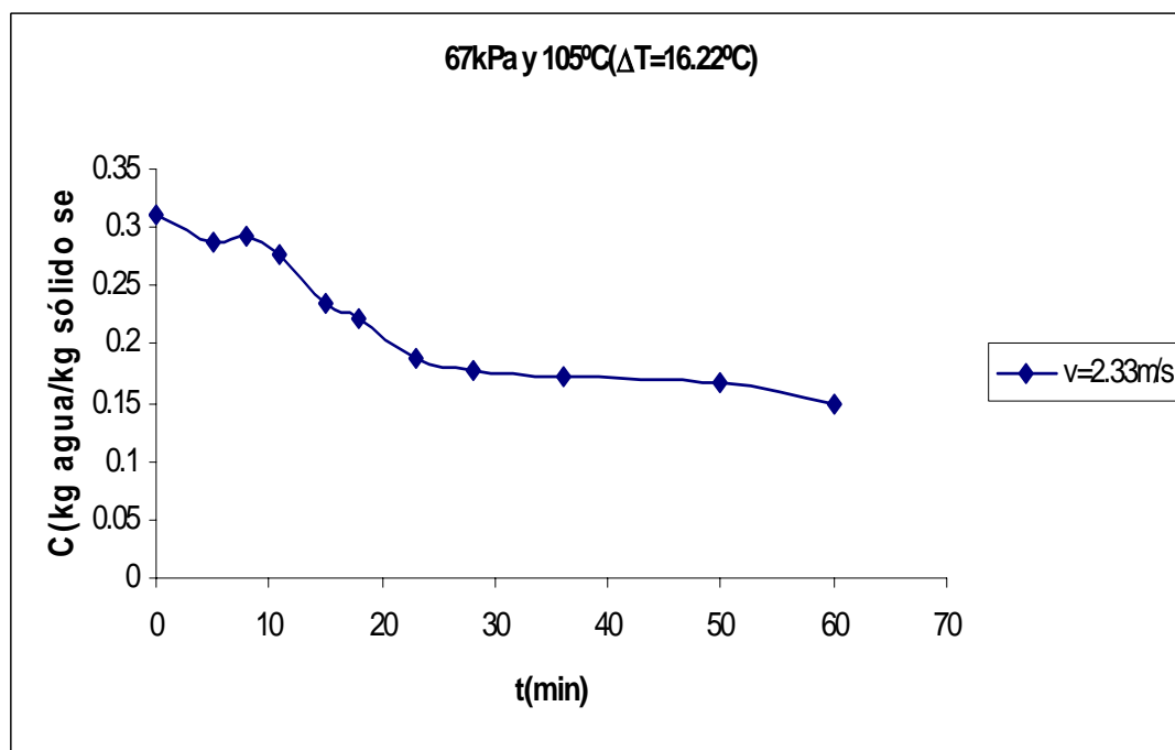
Figura C.52 Curva de secado de arroz con cáscara.
