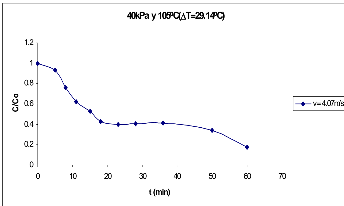
Figura C.23 Curva de secado de arroz con cáscara.
