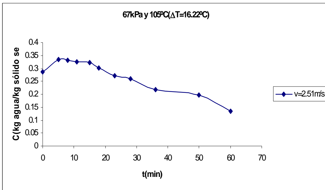
Figura C.61 Curva de secado de arroz con cáscara.
