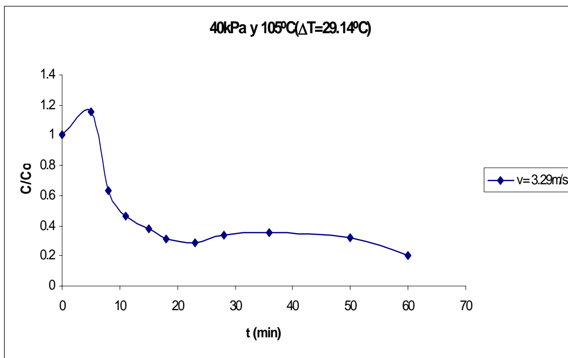
Figura C.14 Curva de secado de arroz con cáscara.
