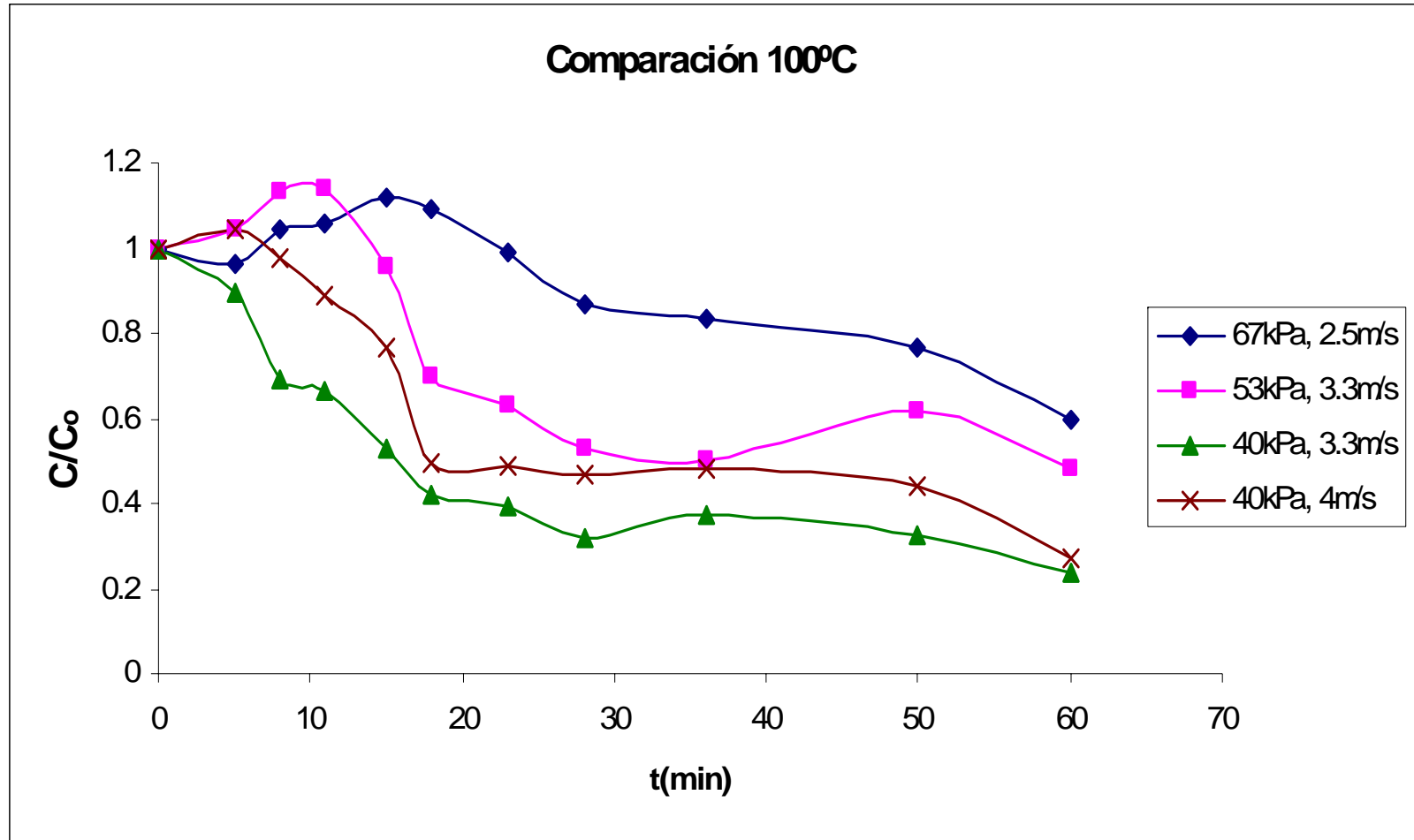
Figura C.67 Comparación de curvas normalizadas de secado.
