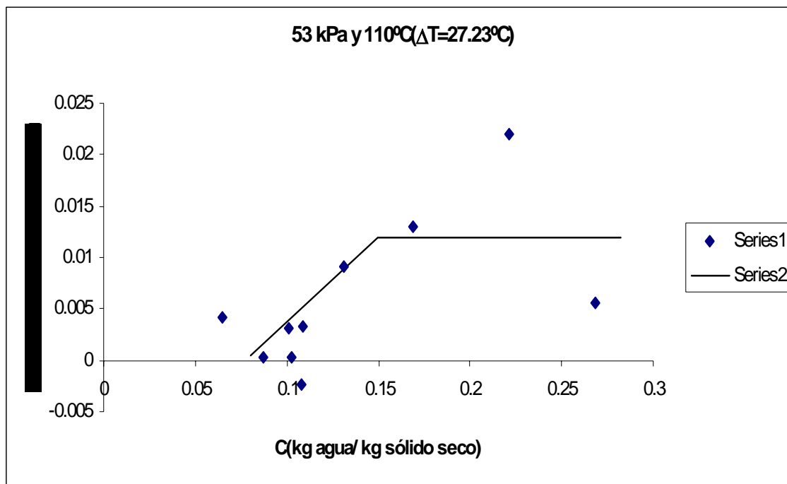
Figura C.45 Velocidad de secado de arroz con cáscara v=3.38 m/s.
