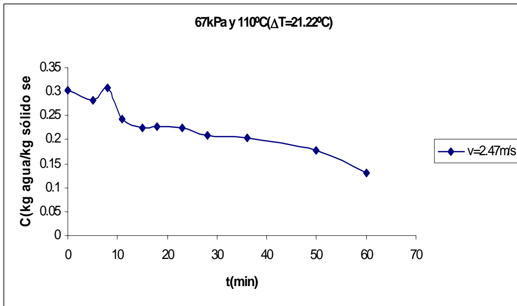
Figura C.64 Curva de secado de arroz con cáscara.
