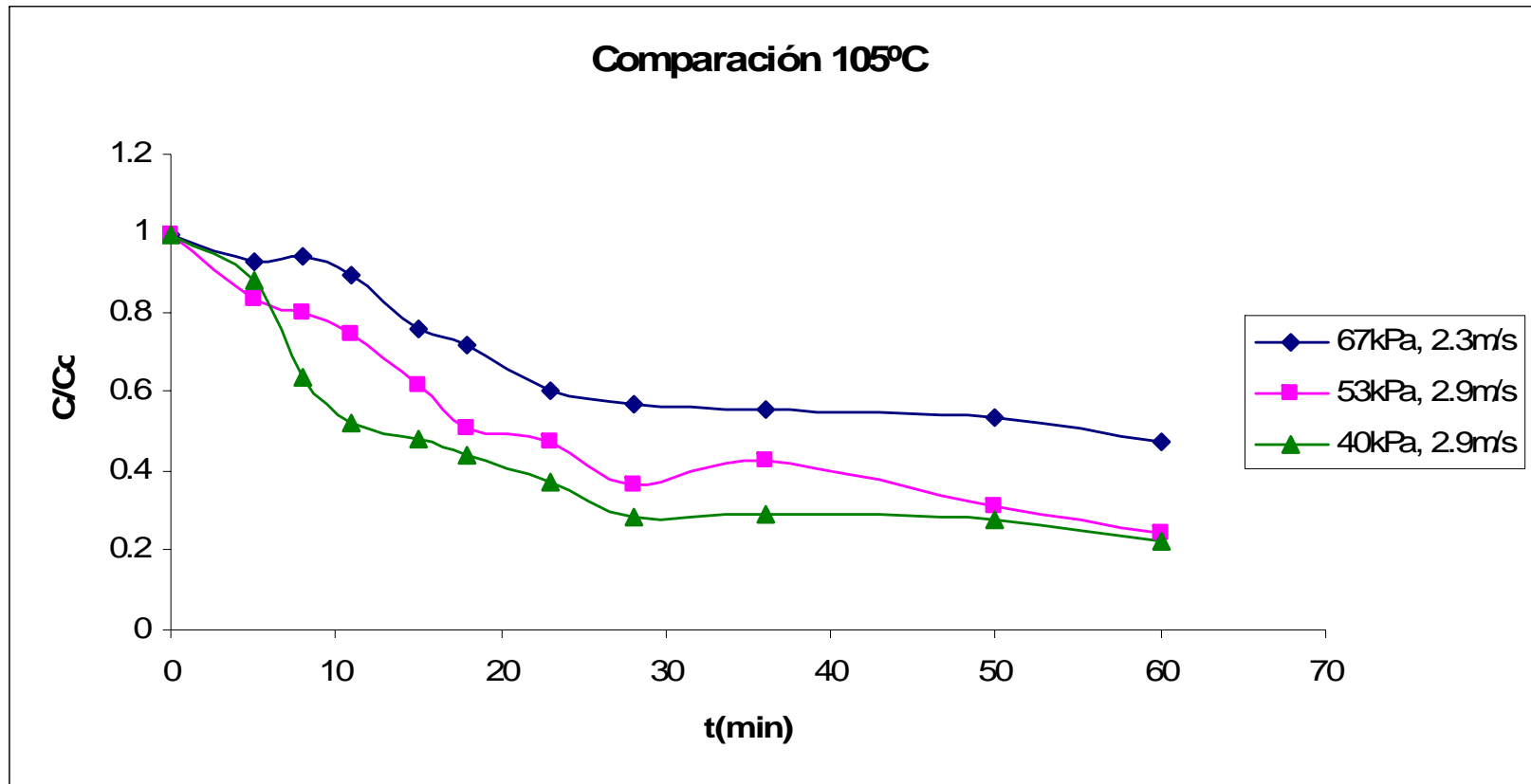
Figura C.70 Comparación de curvas normalizadas de secado.
