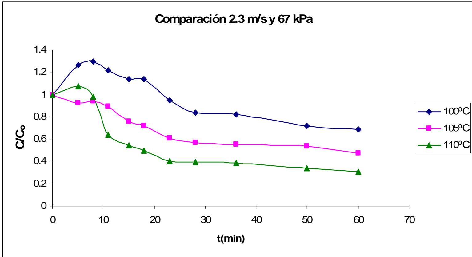
Figura C.78 Comparación de curvas normalizadas de secado.
