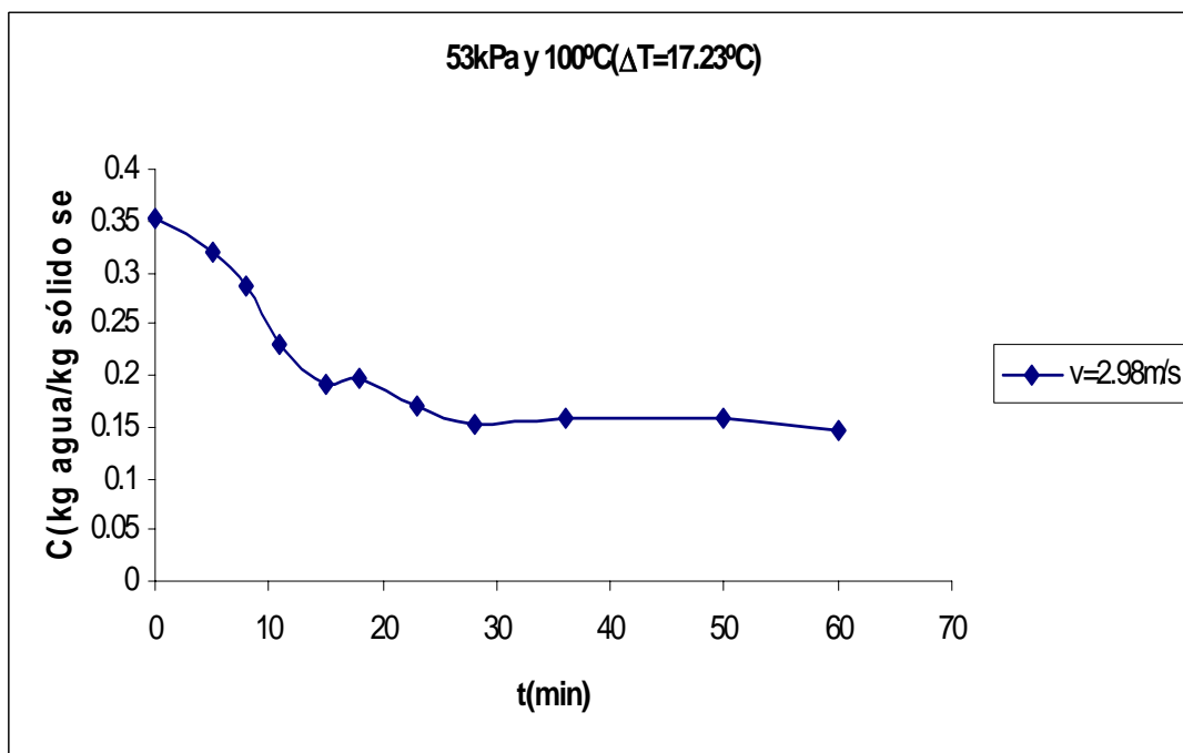
Figura C.28 Curva de secado de arroz con cáscara.
