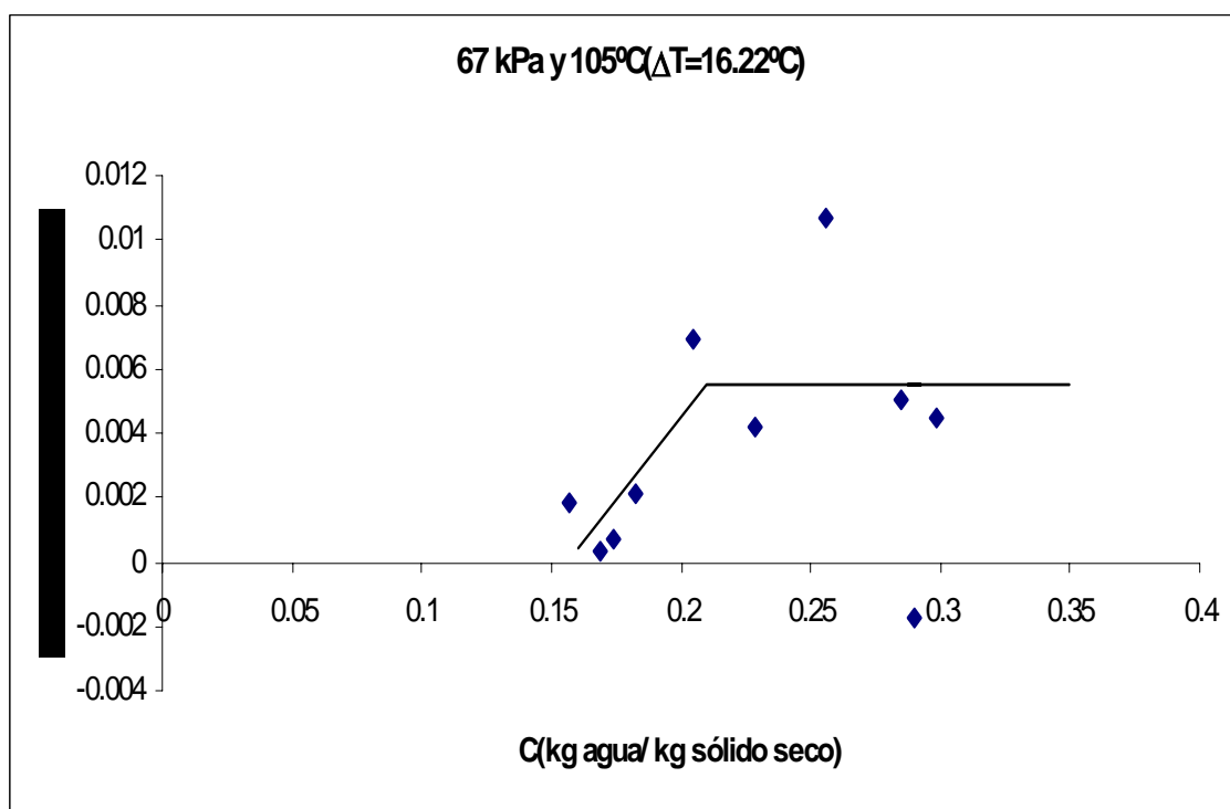
Figura C.54 Velocidad de secado de arroz con cáscara v=2.33 m/s.
