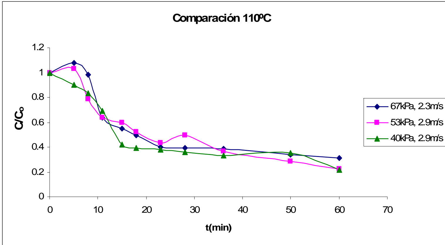
Figura C.72 Comparación de curvas normalizadas de secado.
