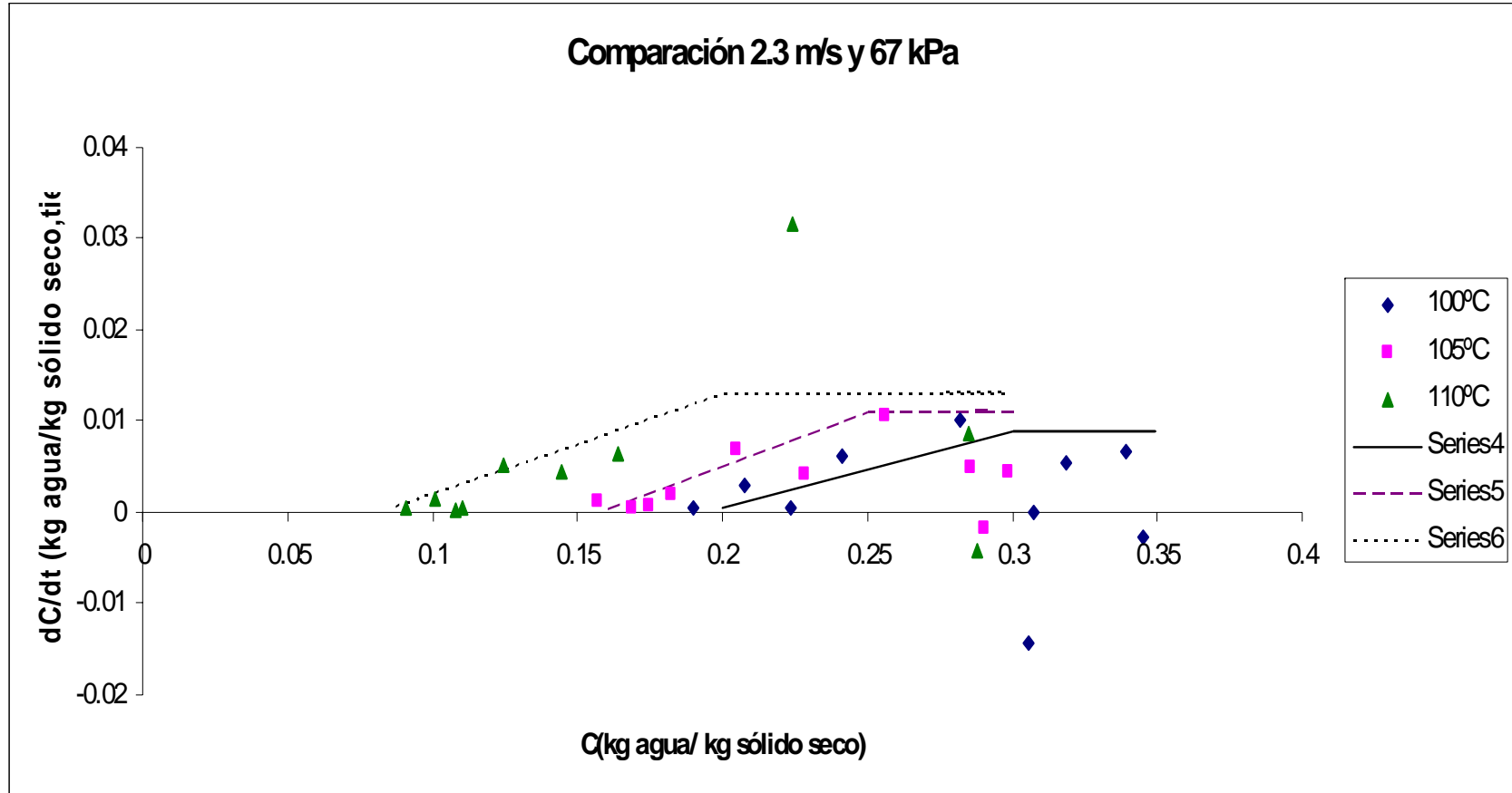
Figura C.93 Comparación de velocidades de secado.
