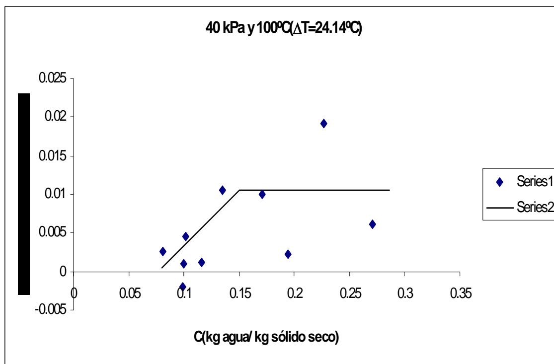
Figura C.12 Velocidad de secado de arroz con cáscara v=3.30 m/s.
