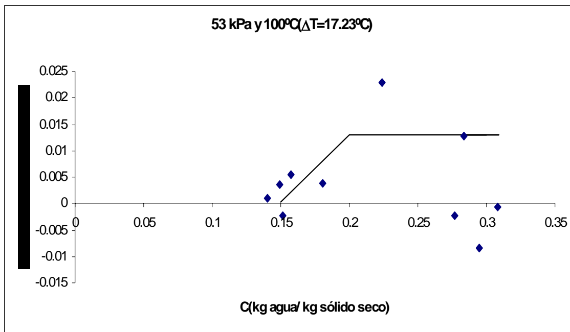
Figura C.39 Velocidad de secado de arroz con cáscara v=3.29 m/s.
