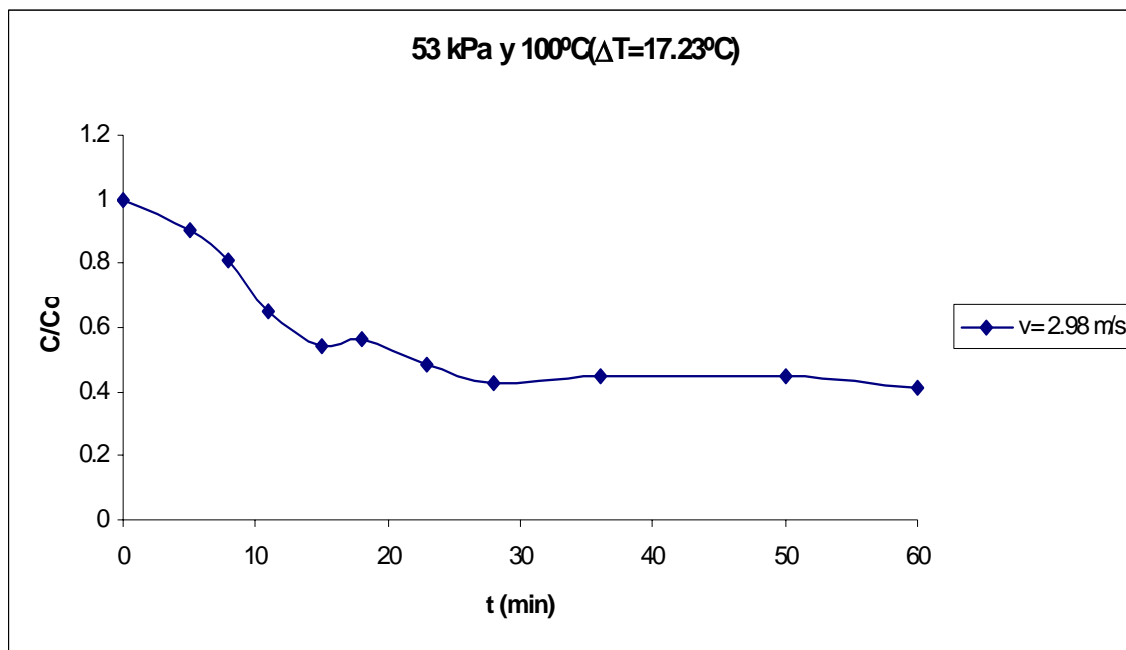
Figura C.29 Curva de secado de arroz con cáscara.
