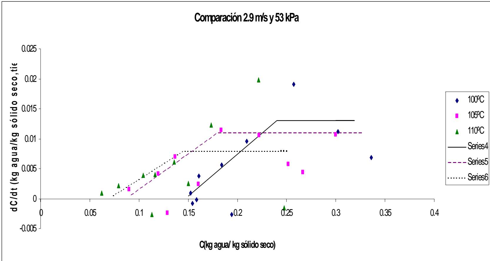
Figura C.89 Comparación de velocidades de secado.
