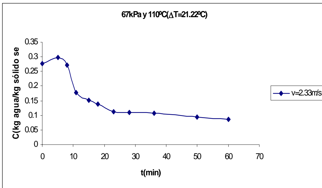
Figura C.55 Curva de secado de arroz con cáscara.
