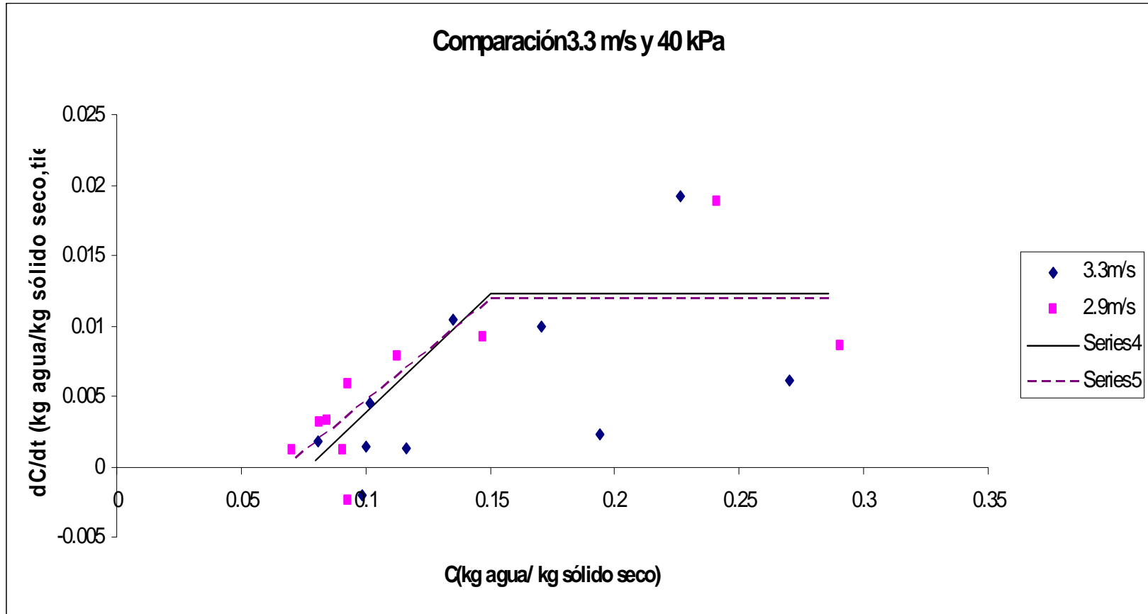
Figura C.97 Comparación de velocidades de secado.
