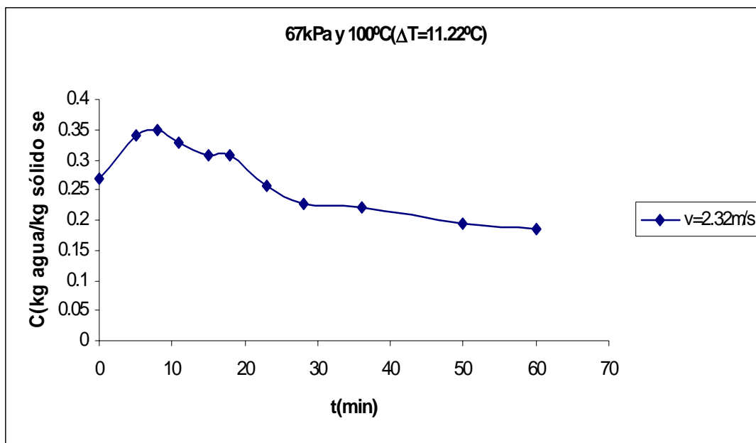
Figura C.49 Curva de secado de arroz con cáscara.
