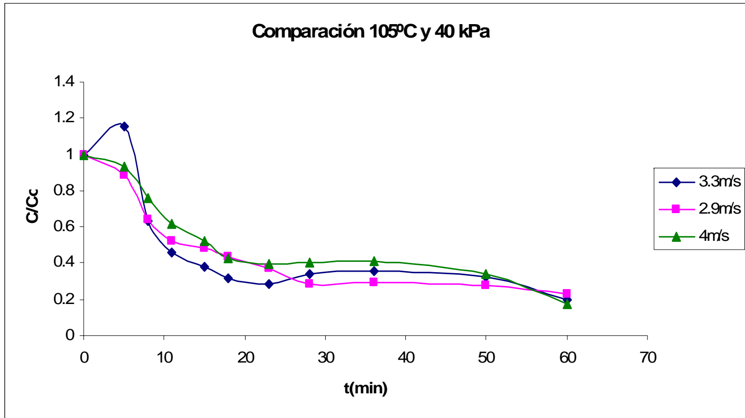
Figura C.81 Comparación de curvas normalizadas de secado.
