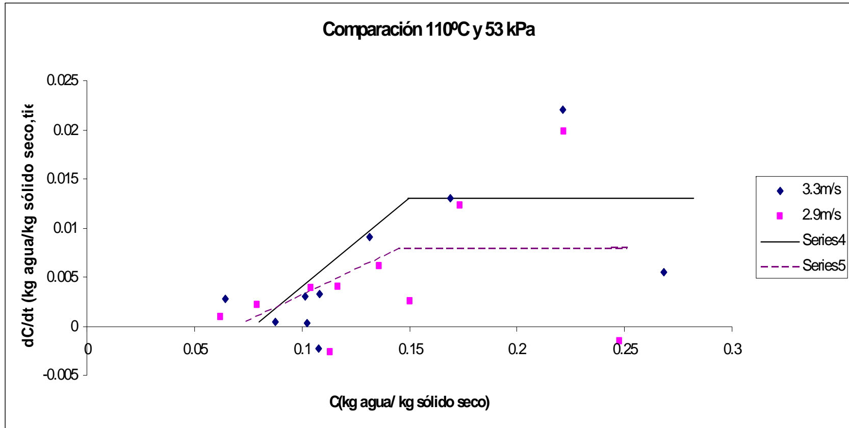
Figura C.92 Comparación de velocidades de secado.
