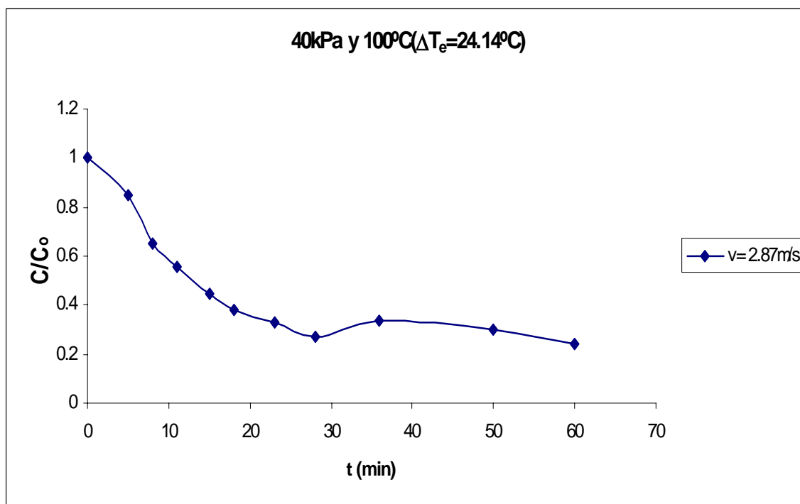
Figura C.2 Curva de secado de arroz con cáscara.
