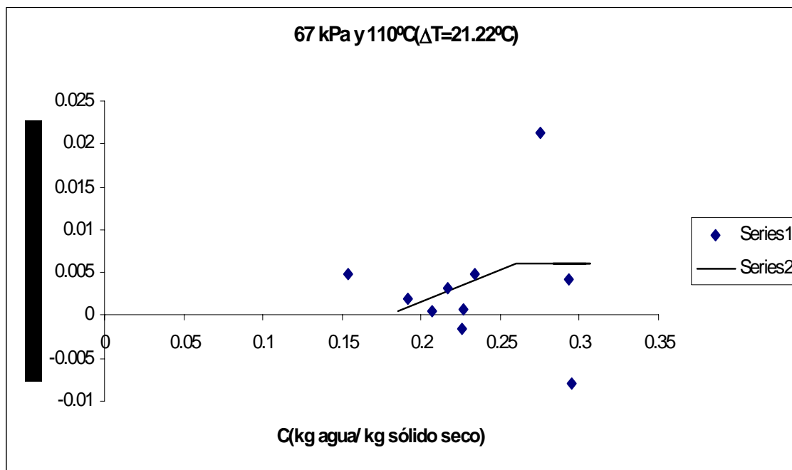
Figura C.66 Velocidad de secado de arroz con cáscara v=2.47 m/s.
