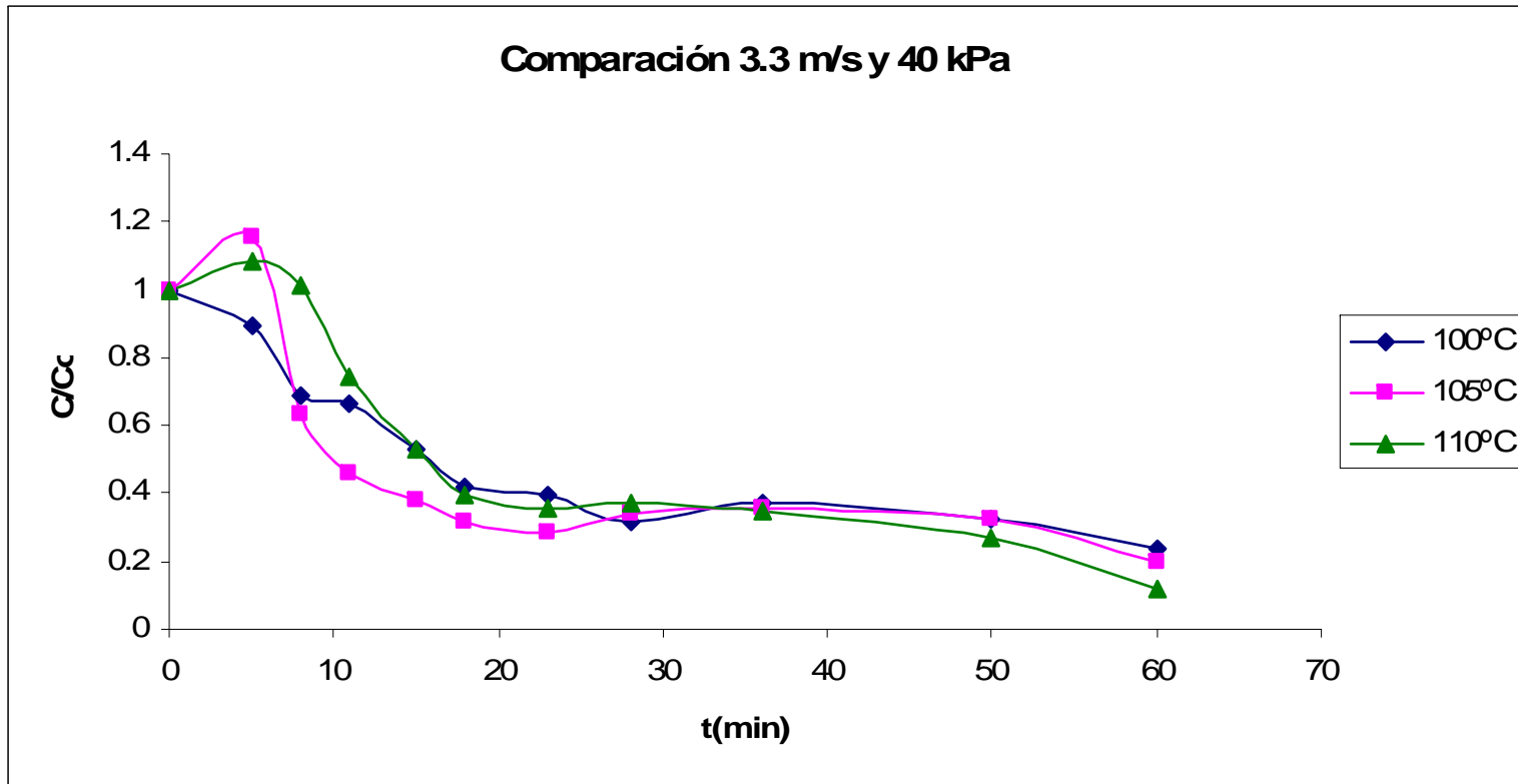
Figura C.74 Comparación de curvas normalizadas de secado.
