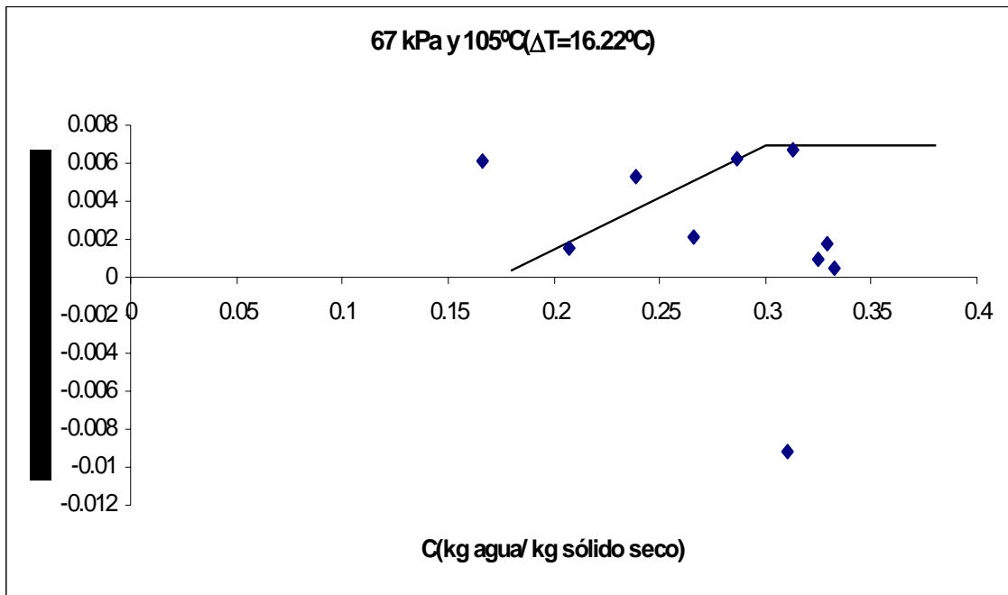
Figura C.63 Velocidad de secado de arroz con cáscara v=2.51 m/s.
