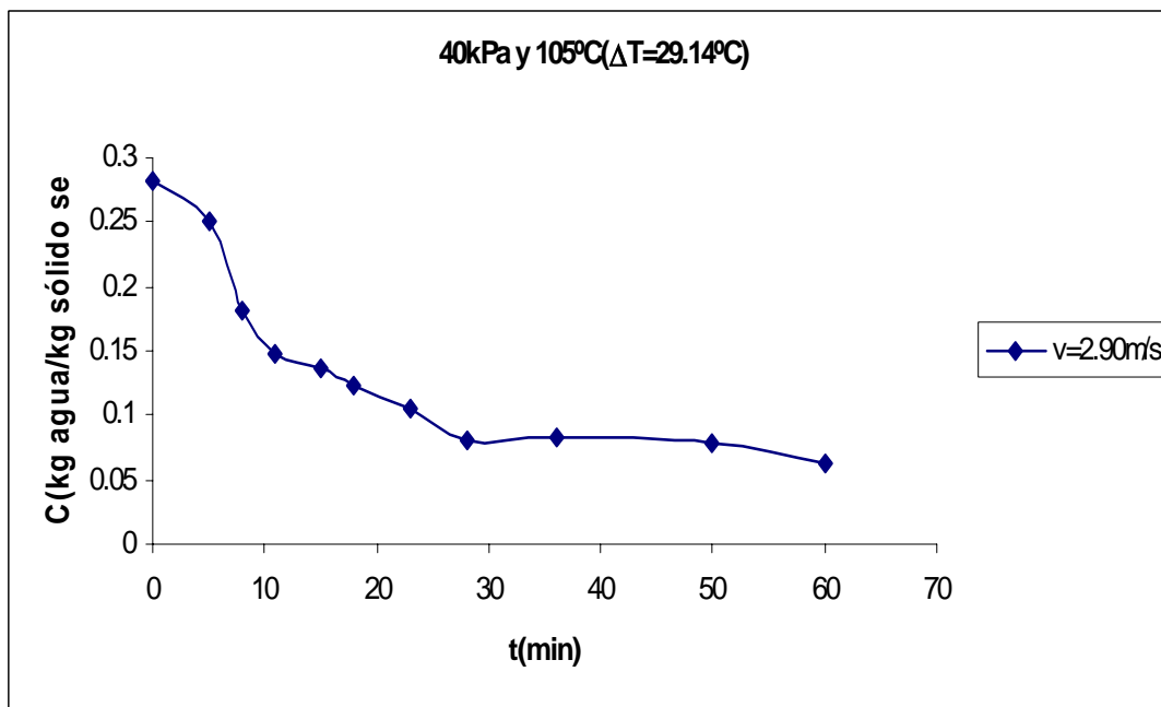
Figura C.4 Curva de secado de arroz con cáscara.
