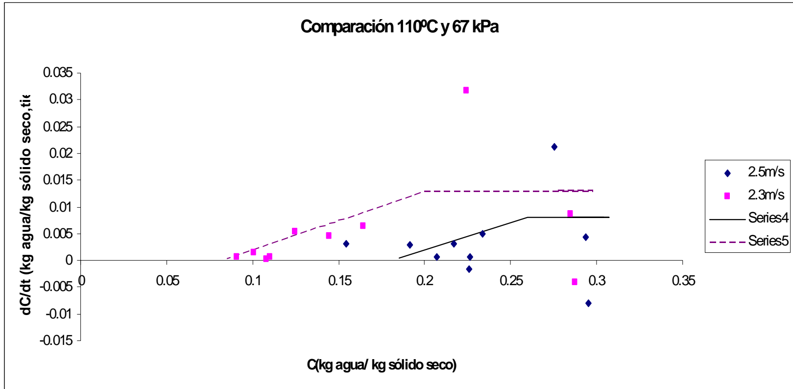
Figura C.95 Comparación de velocidades de secado.
