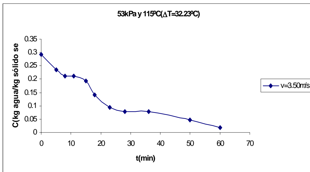
Figura C.46 Curva de secado de arroz con cáscara.
