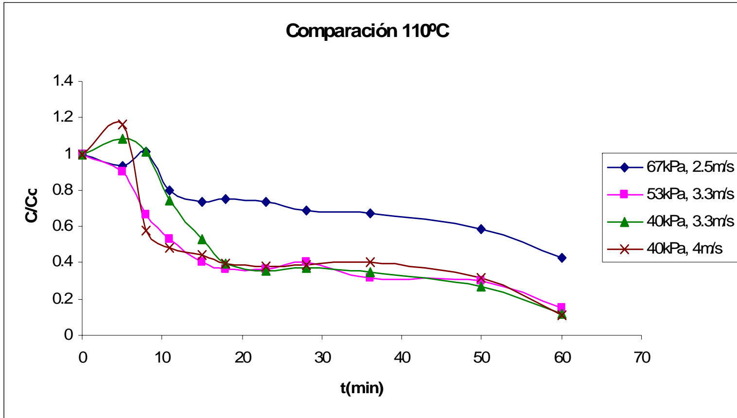
Figura C.71 Comparación de curvas normalizadas de secado.
