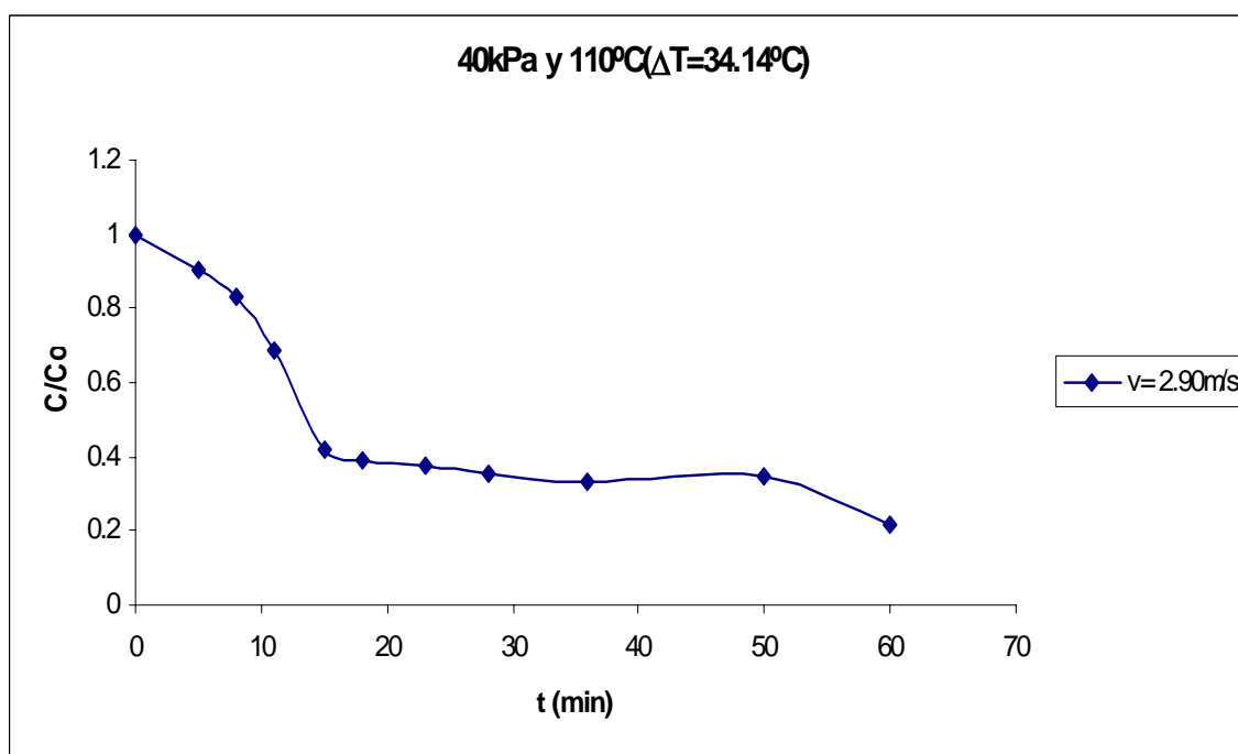
Figura C.8 Curva de secado de arroz con cáscara.
