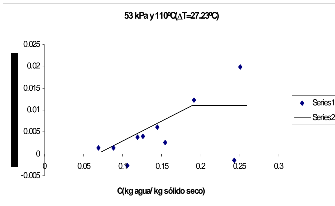
Figura C.36 Velocidad de secado de arroz con cáscara v=2.91 m/s.
