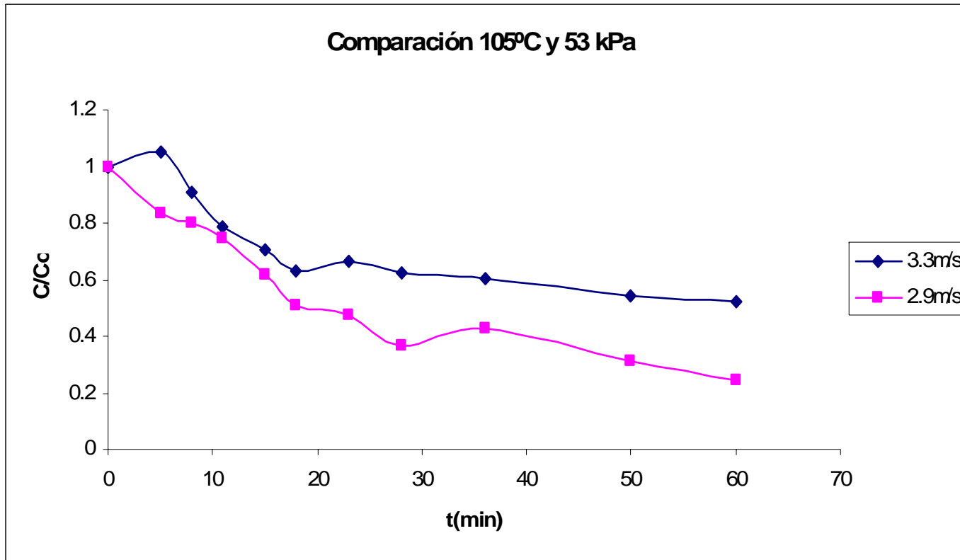
Figura C.84 Comparación de curvas normalizadas de secado.
