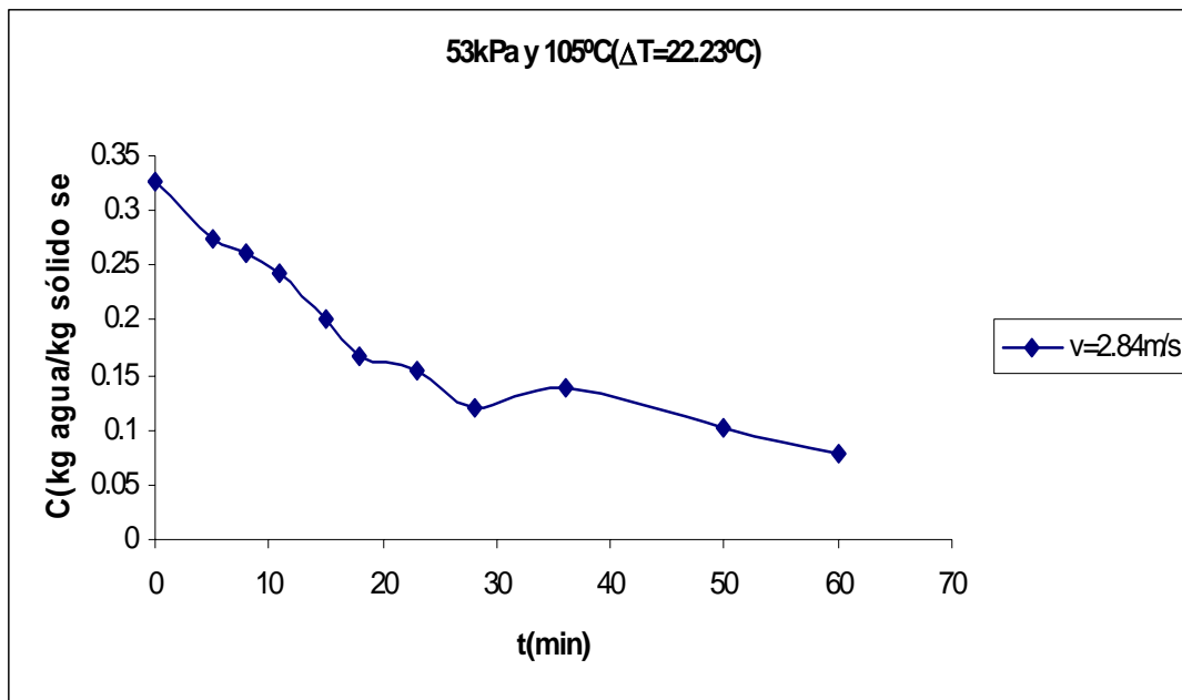
Figura C.31 Curva de secado de arroz con cáscara.
