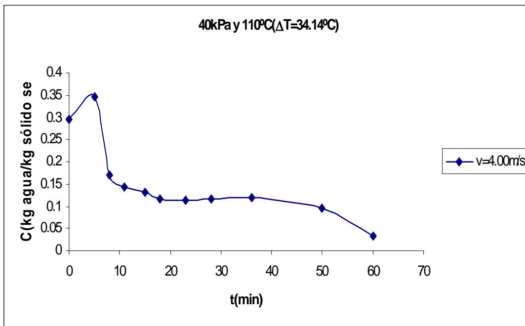
Figura C.25 Curva de secado de arroz con cáscara.
