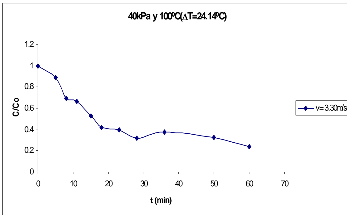
Figura C.11 Curva de secado de arroz con cáscara.
