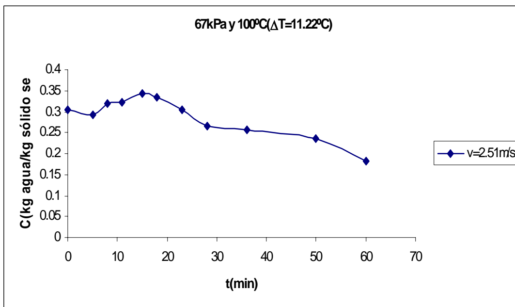
Figura C.58 Curva de secado de arroz con cáscara.
