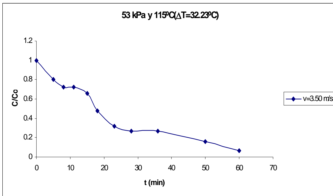
Figura C.47 Curva de secado de arroz con cáscara.
