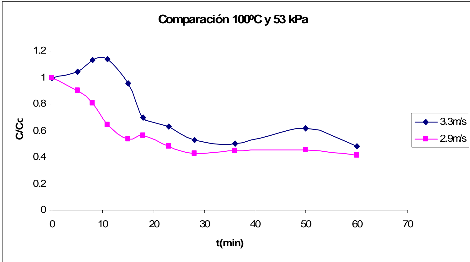
Figura C.83 Comparación de curvas normalizadas de secado.
