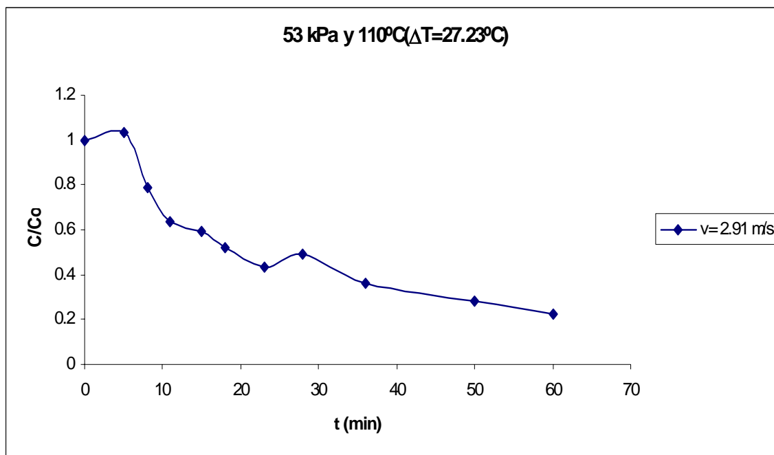
Figura C.35 Curva de secado de arroz con cáscara.
