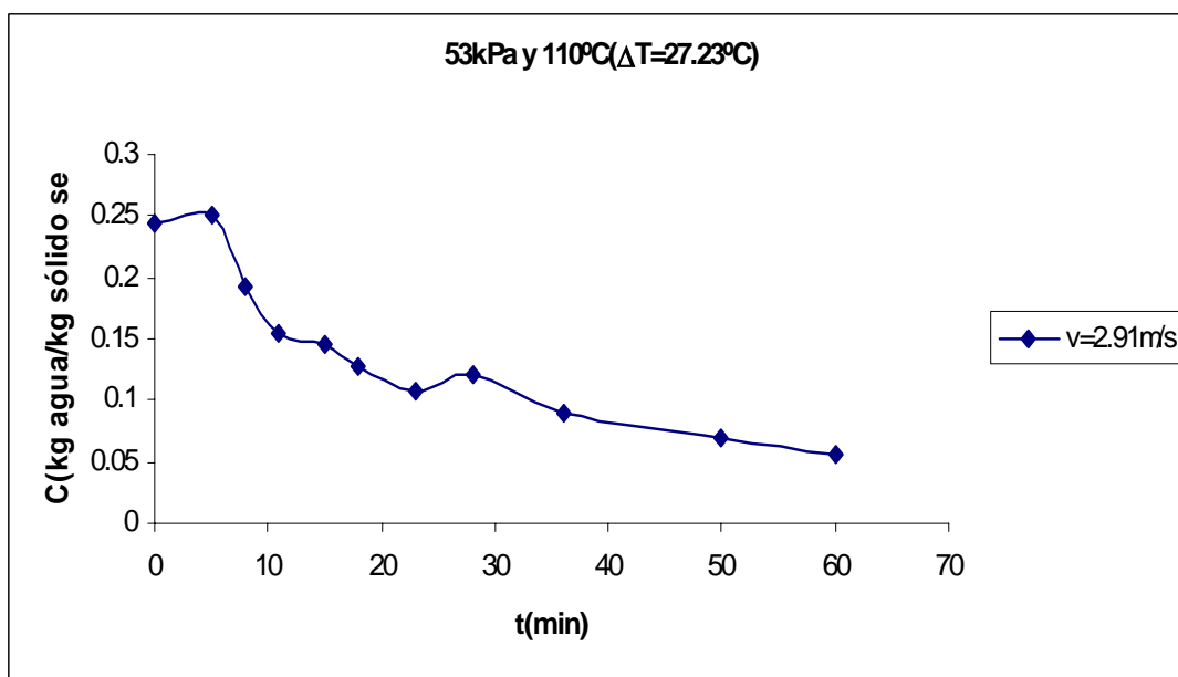
Figura C.34 Curva de secado de arroz con cáscara.
