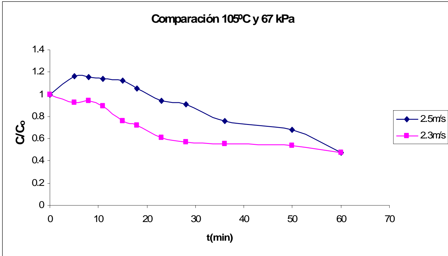
Figura C.87 Comparación de curvas normalizadas de secado.
