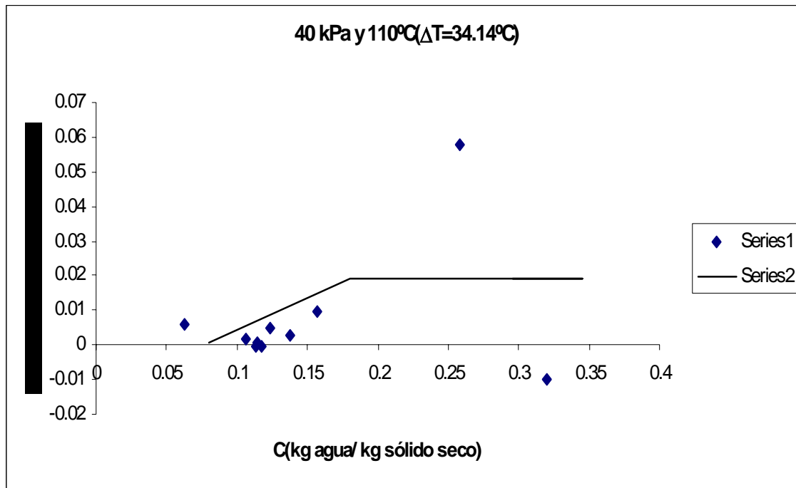
Figura C.27 Velocidad de secado de arroz con cáscara v=4.0 m/s.
