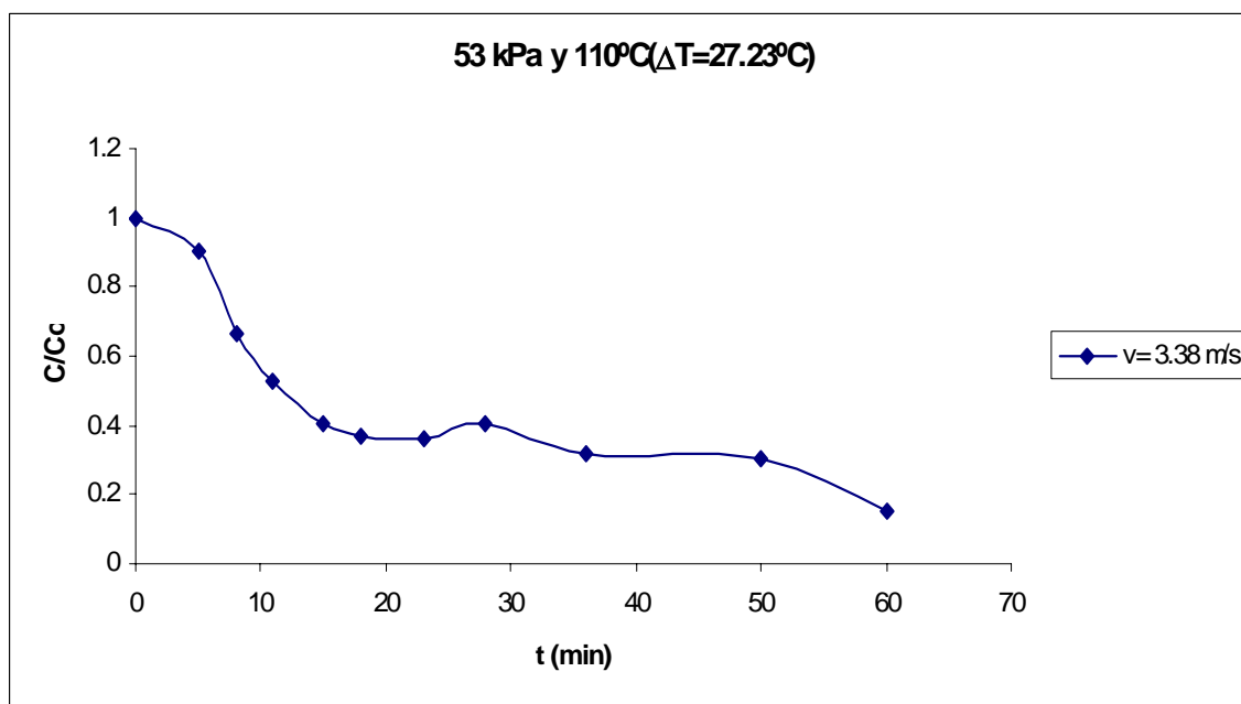
Figura C.44 Curva de secado de arroz con cáscara.
