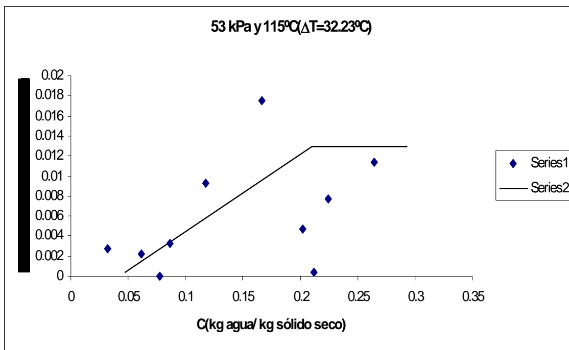
Figura C.48 Velocidad de secado de arroz con cáscara v=3.50 m/s.
