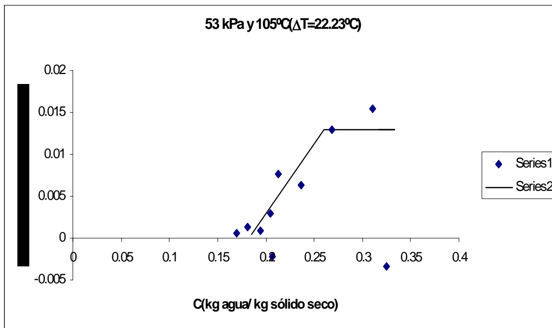
Figura C.42 Velocidad de secado de arroz con cáscara v=3.34 \text{ m/s} .
