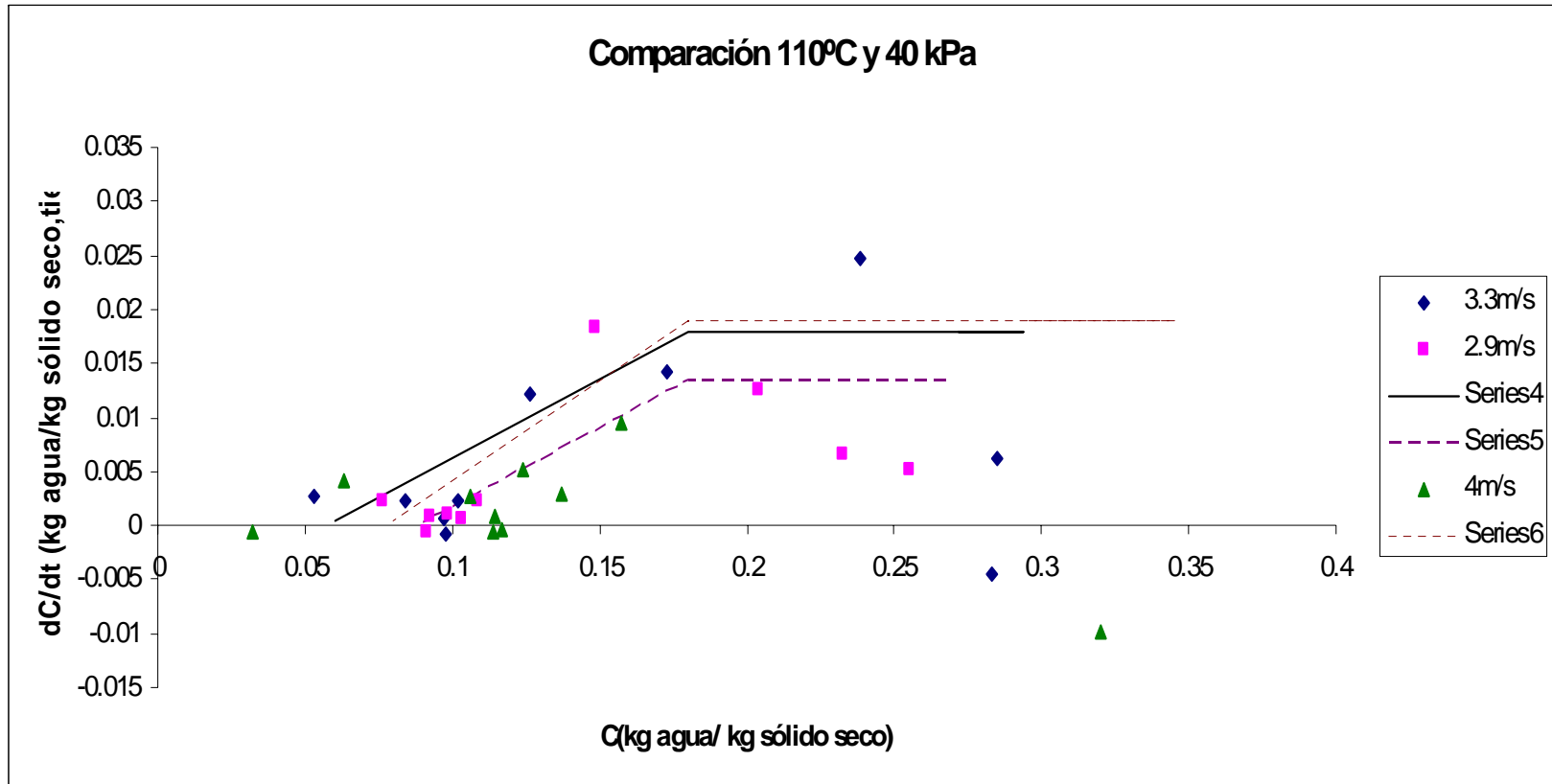
Figura C.96 Comparación de velocidades de secado.
