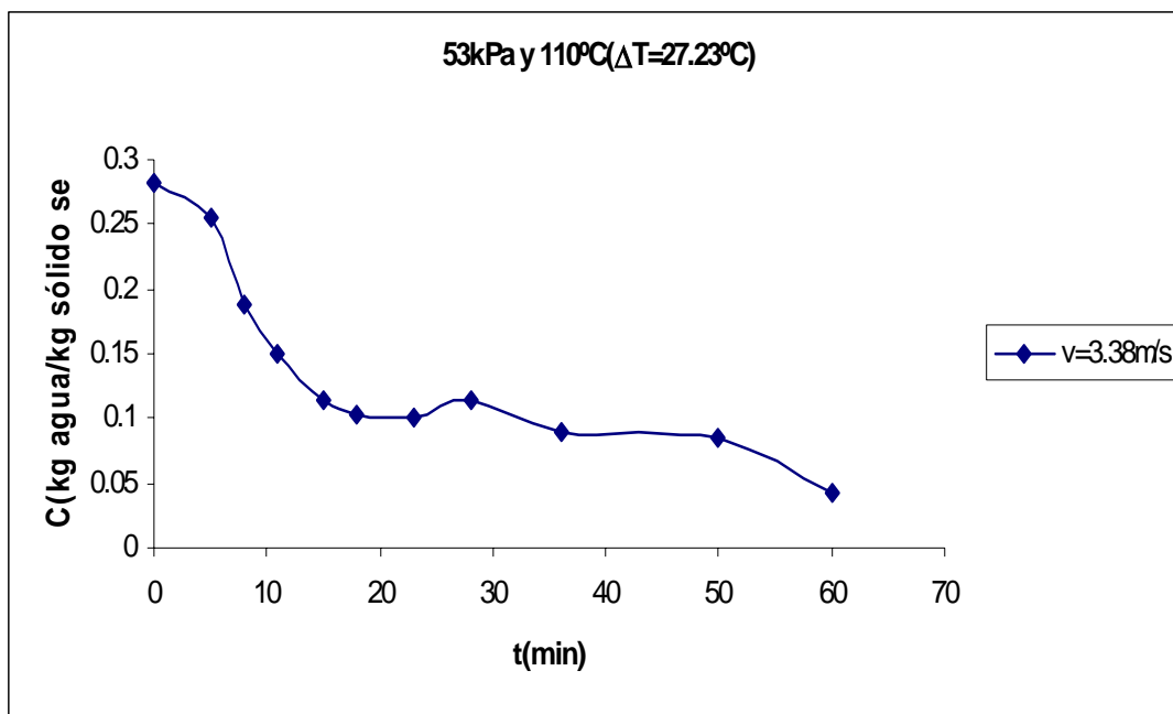
Figura C.43 Curva de secado de arroz con cáscara.
