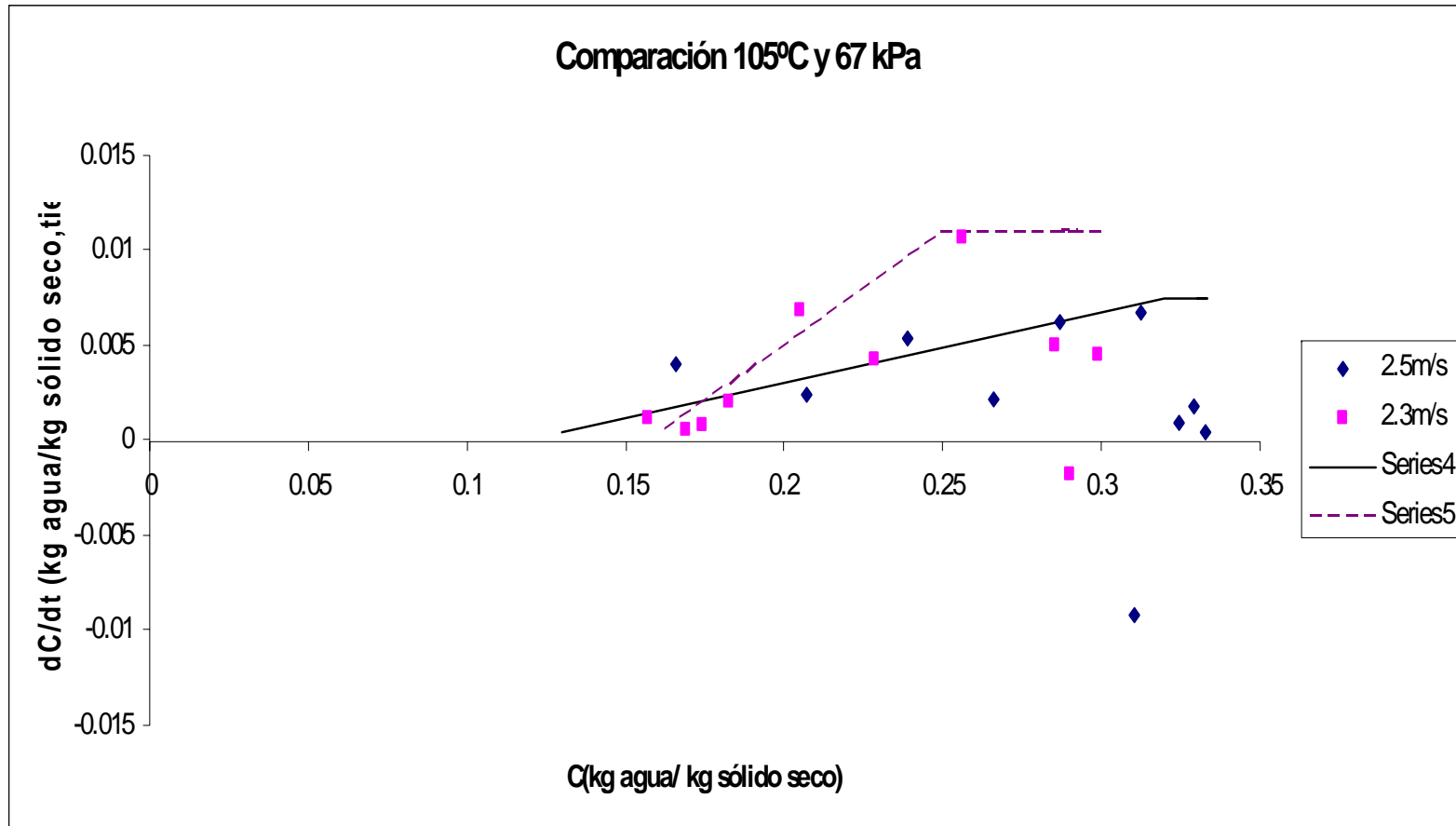
Figura C.94 Comparación de velocidades de secado.
