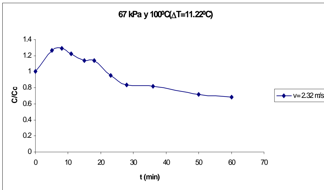
Figura C.50 Curva de secado de arroz con cáscara.
