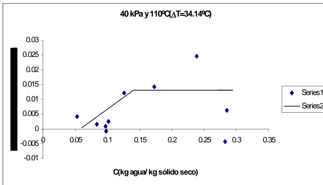
Figura C.18 Velocidad de secado de arroz con cáscara v=3.28 m/s.
