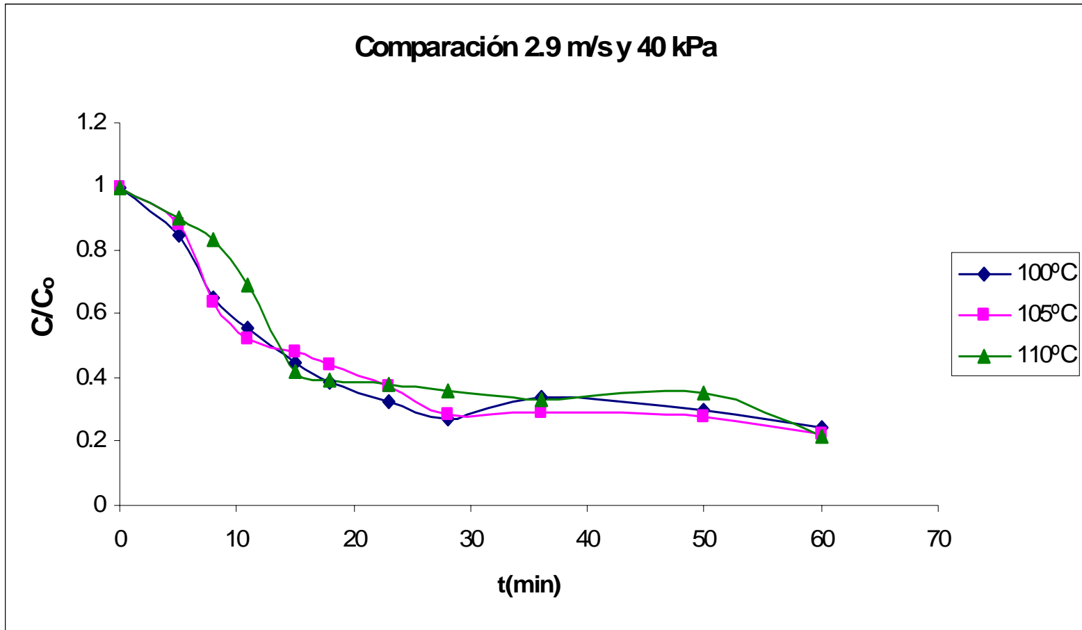
Figura C.73 Comparación de curvas normalizadas de secado.
