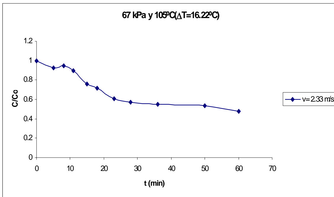
Figura C.53 Curva de secado de arroz con cáscara.
