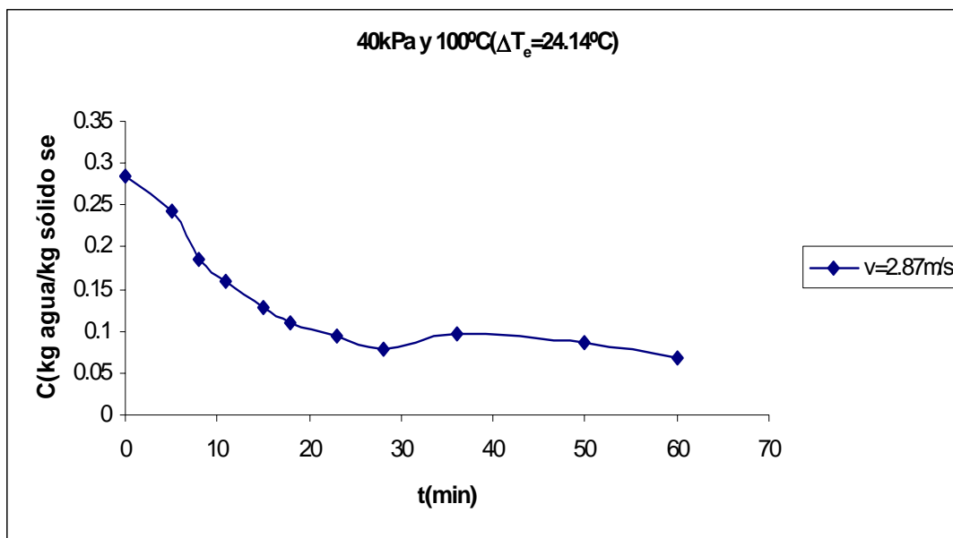
Figura C.1 Curva de secado de arroz con cáscara.
