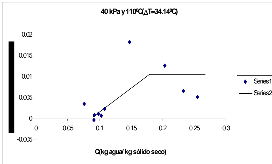
Figura C.9 Velocidad de secado de arroz con cáscara v=2.90 m/s.
