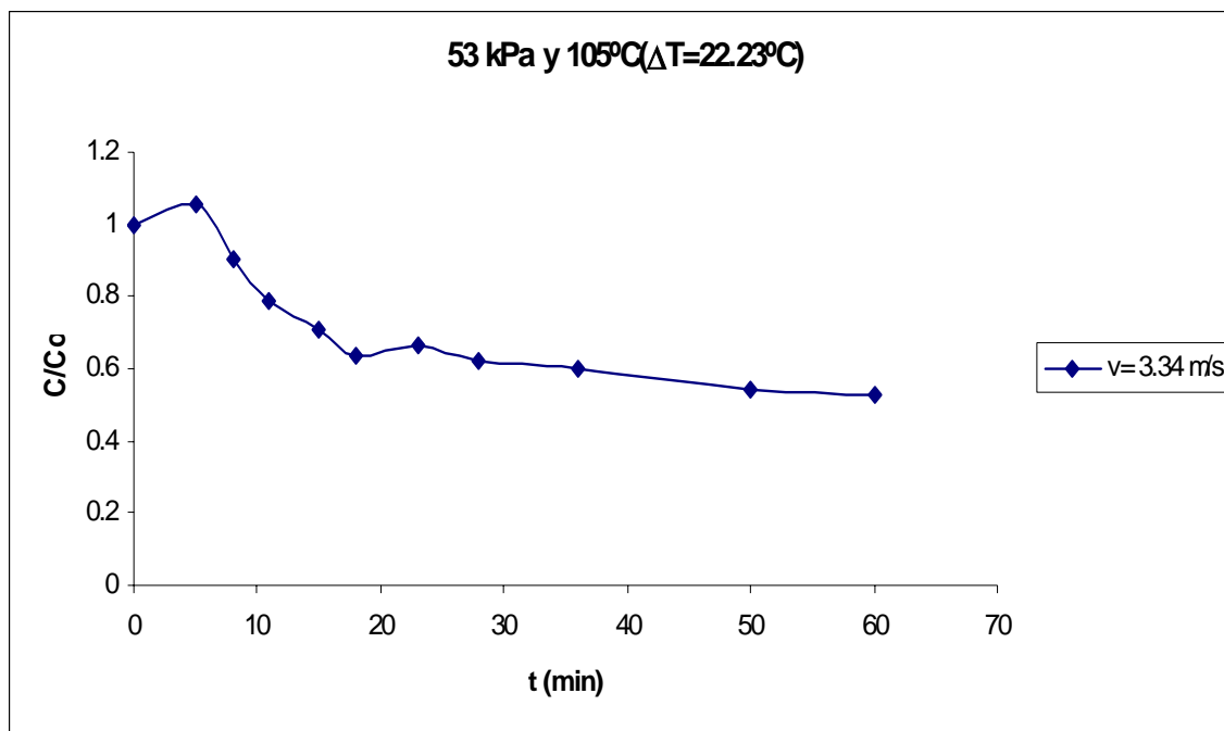
Figura C.41 Curva de secado de arroz con cáscara.
