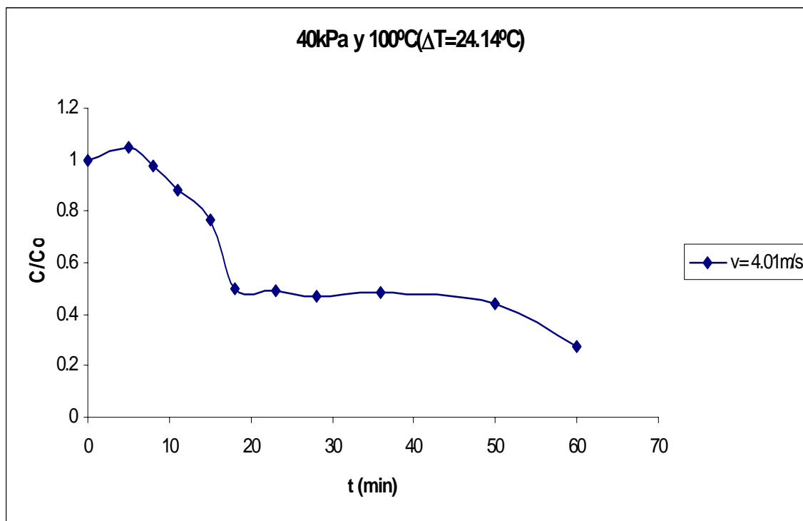
Figura C.20 Curva de secado de arroz con cáscara.
