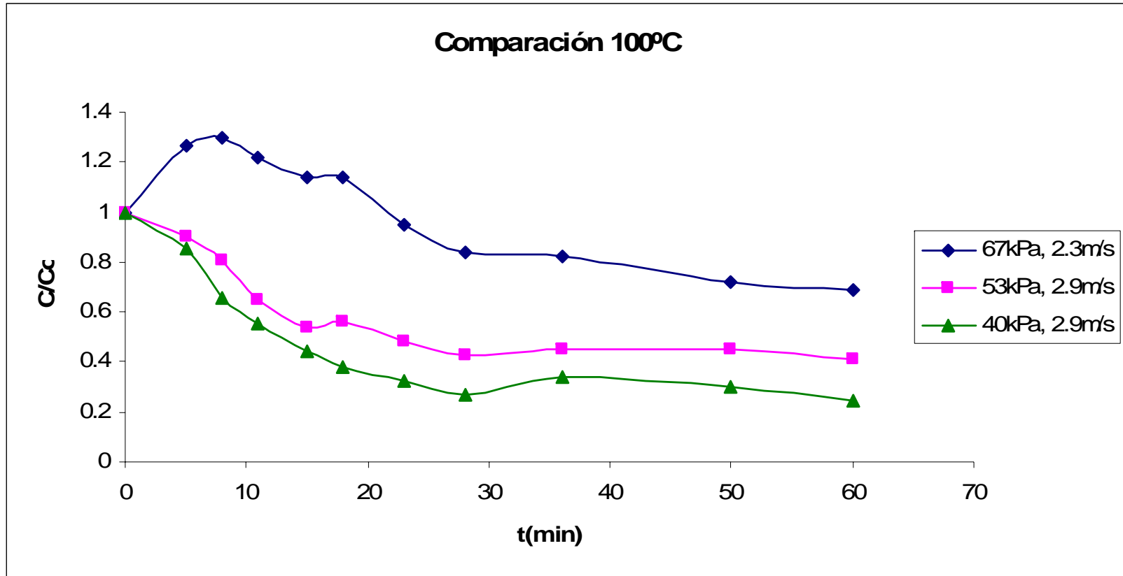
Figura C.68 Comparación de curvas normalizadas de secado.
