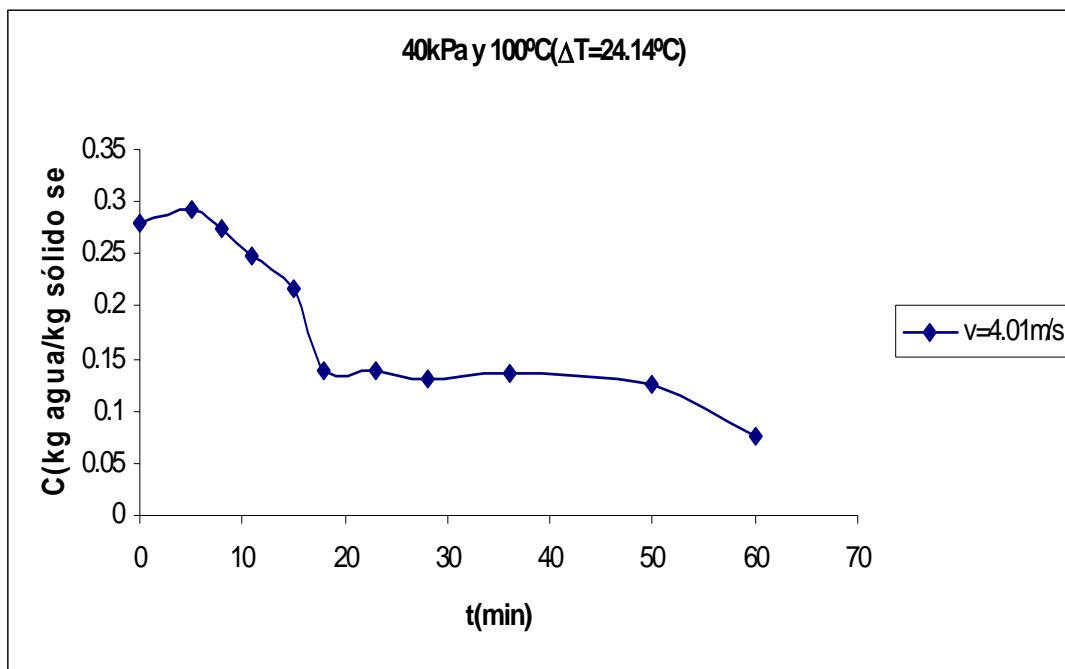
Figura C.19 Curva de secado de arroz con cáscara.
