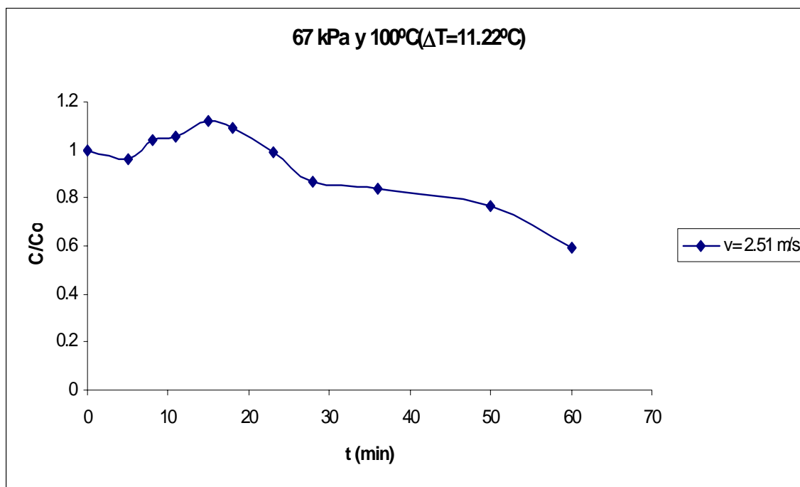
Figura C.59 Curva de secado de arroz con cáscara.
