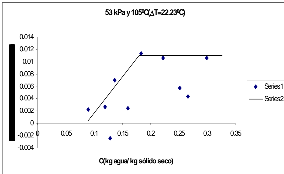
Figura C.33 Velocidad de secado de arroz con cáscara v=2.84 m/s.
