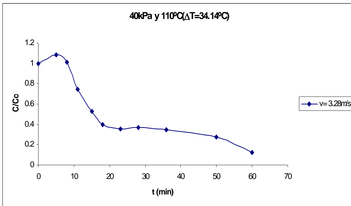
Figura C.17 Curva de secado de arroz con cáscara.
