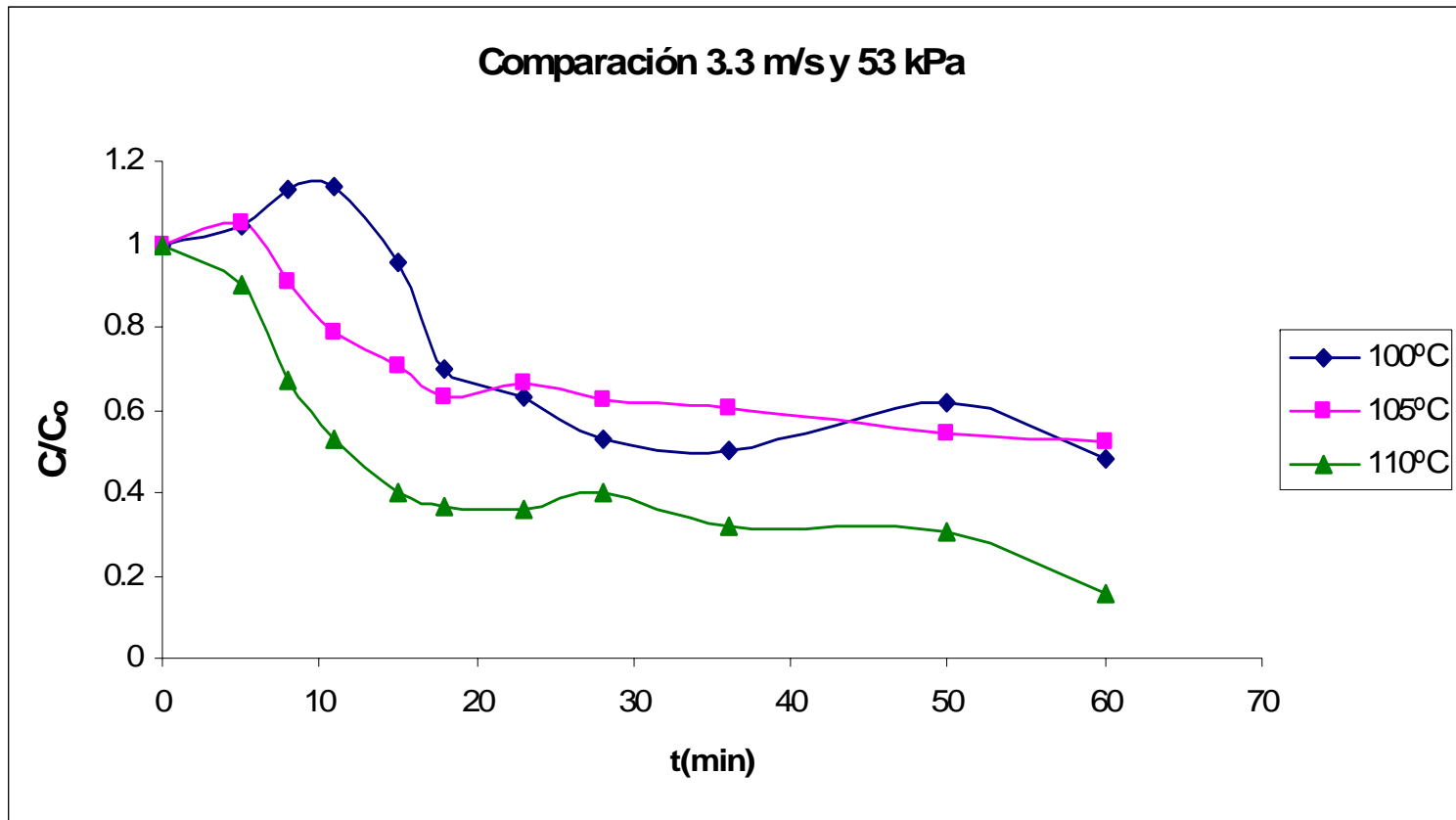
Figura C.77 Comparación de curvas normalizadas de secado.
