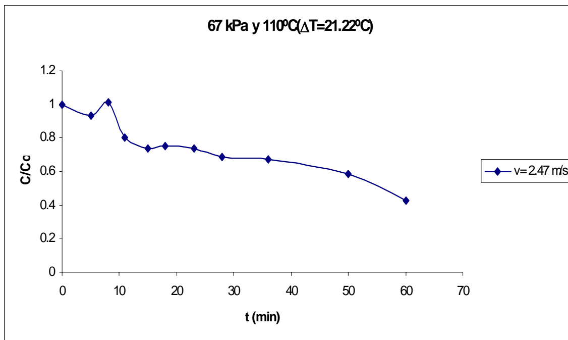
Figura C.65 Curva de secado de arroz con cáscara.
