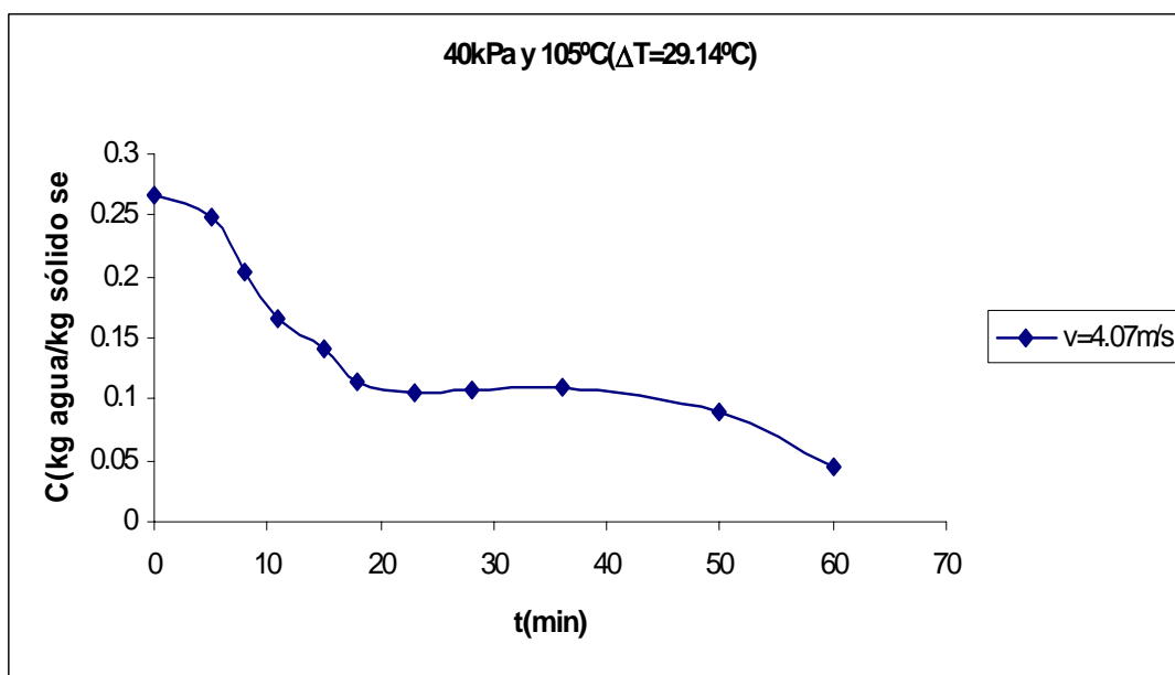
Figura C.22 Curva de secado de arroz con cáscara.
