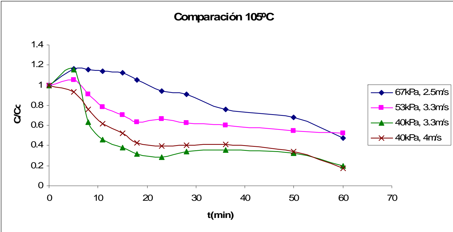
Figura C.69 Comparación de curvas normalizadas de secado.
