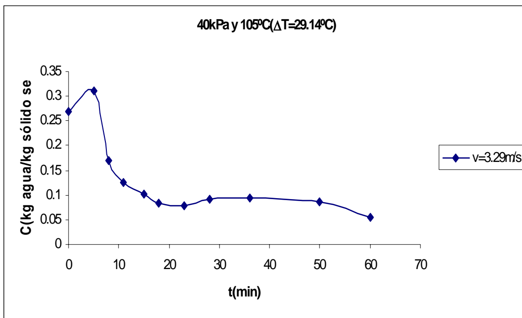
Figura C.13 Curva de secado de arroz con cáscara.
