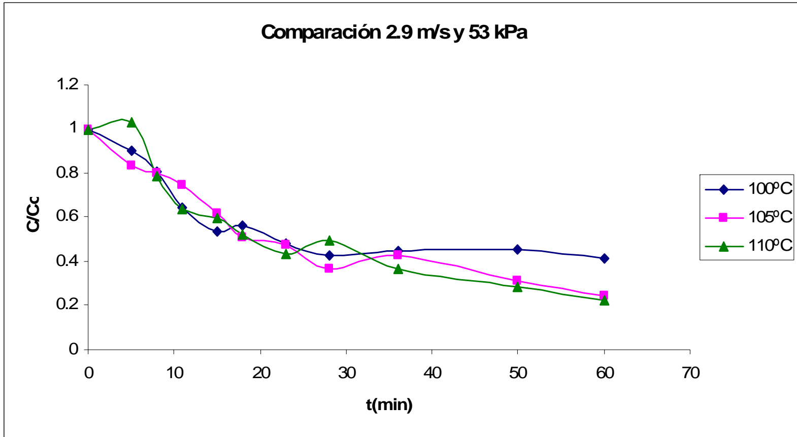
Figura C.76 Comparación de curvas normalizadas de secado.
