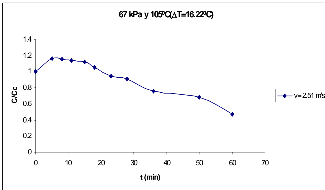
Figura C.62 Curva de secado de arroz con cáscara.
