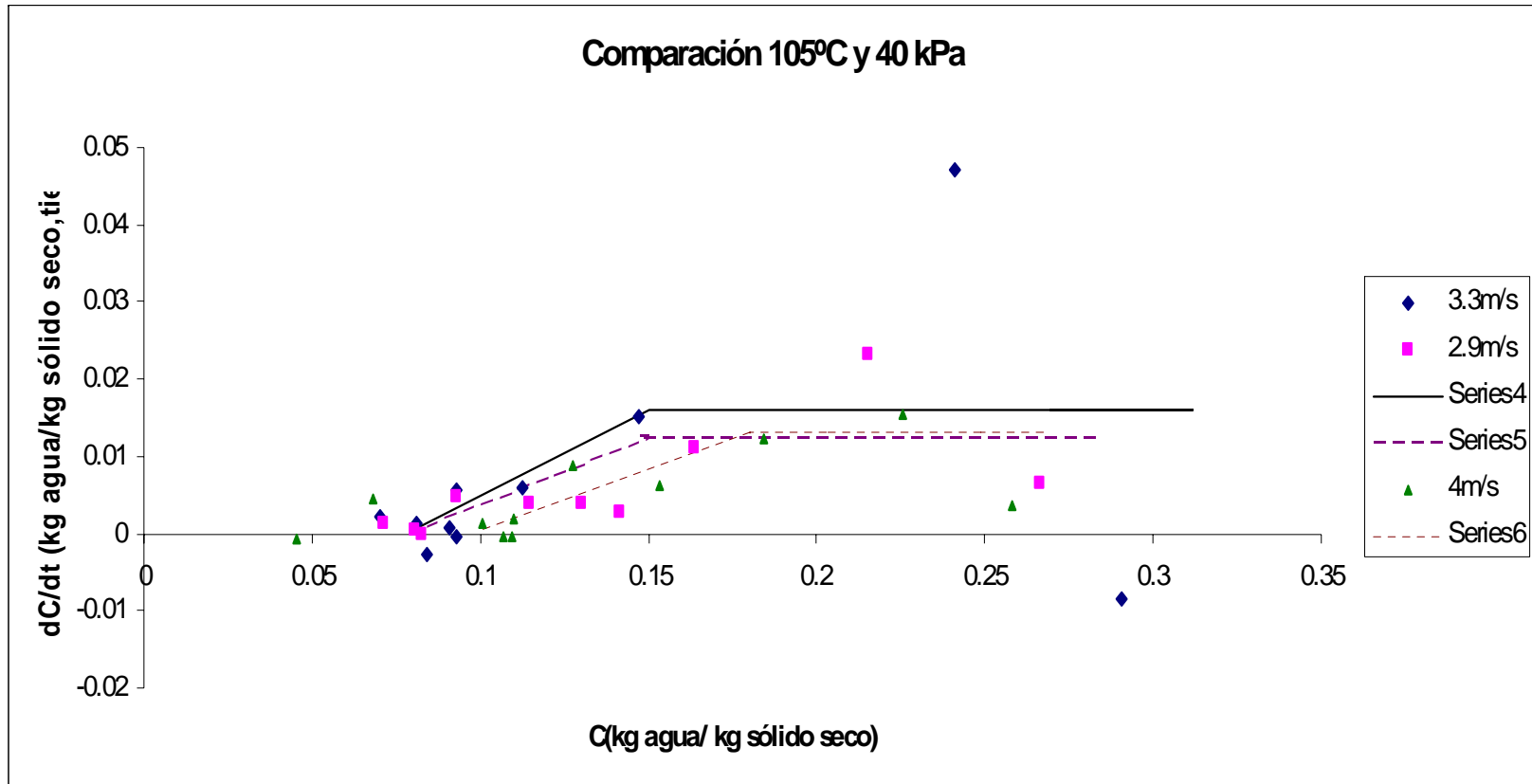
Figura C.98 Comparación de velocidades de secado.
