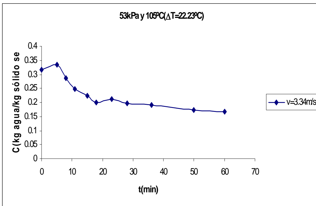
Figura C.40 Curva de secado de arroz con cáscara.
