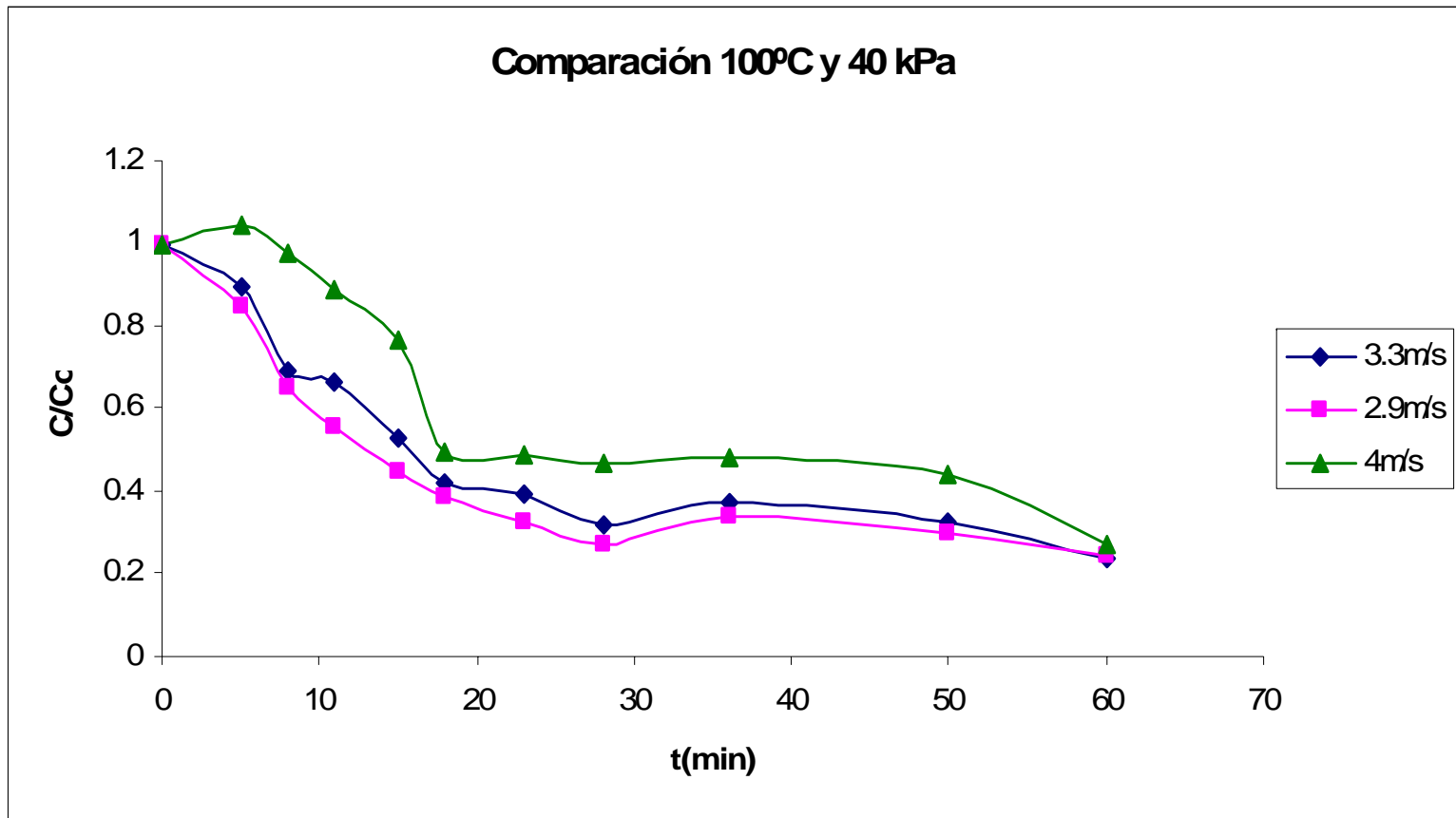
Figura C.80 Comparación de curvas normalizadas de secado.
