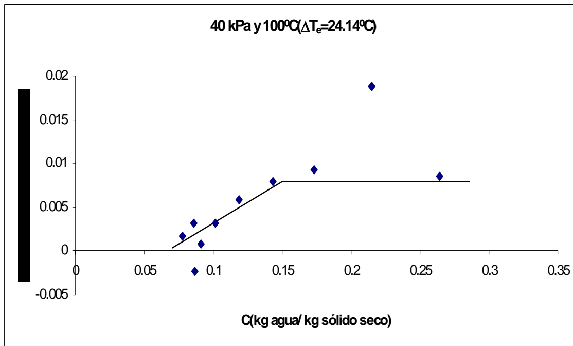
Figura C.3 Velocidad de secado de arroz con cáscara v=2.87 m/s.
