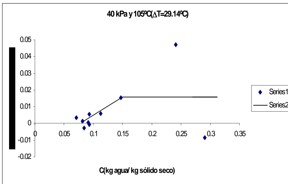
Figura C.15 Velocidad de secado de arroz con cáscara v=3.29 m/s.
