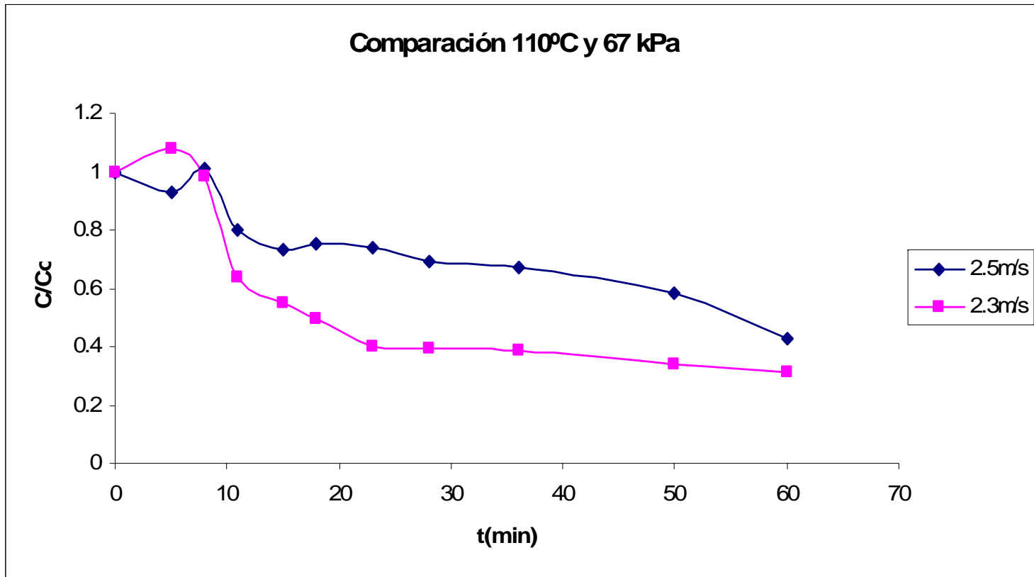
Figura C.88 Comparación de curvas normalizadas de secado.
