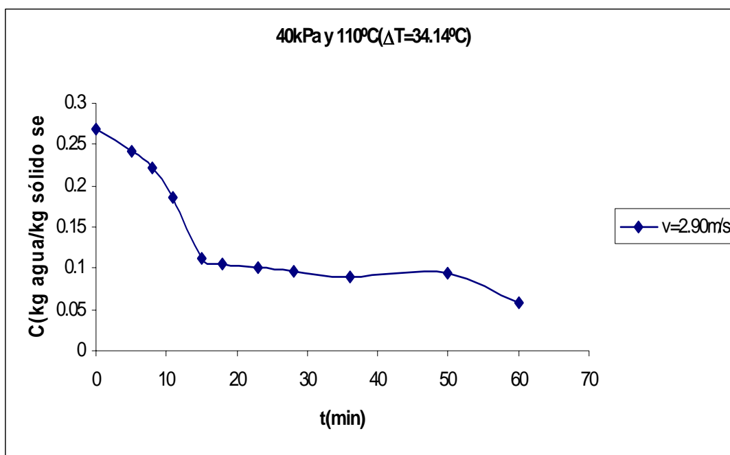
Figura C.7 Curva de secado de arroz con cáscara.
