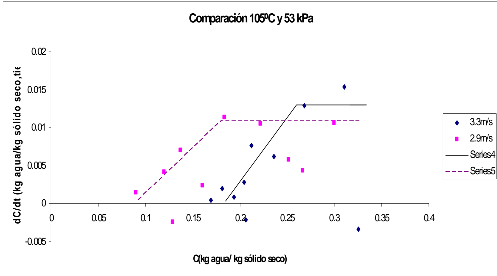
Figura C.91 Comparación de velocidades de secado.
