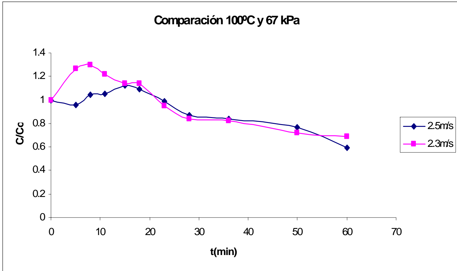
Figura C.86 Comparación de curvas normalizadas de secado.
