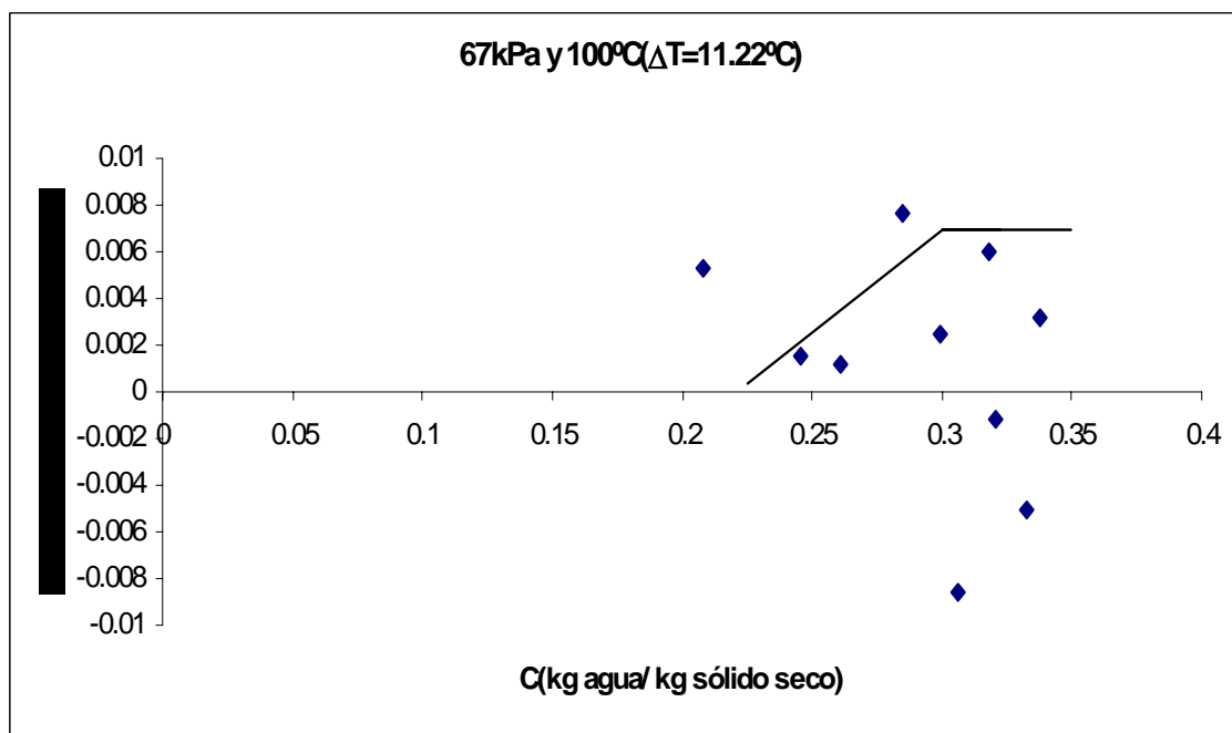
Figura C.60 Velocidad de secado de arroz con cáscara v=2.51 m/s.
