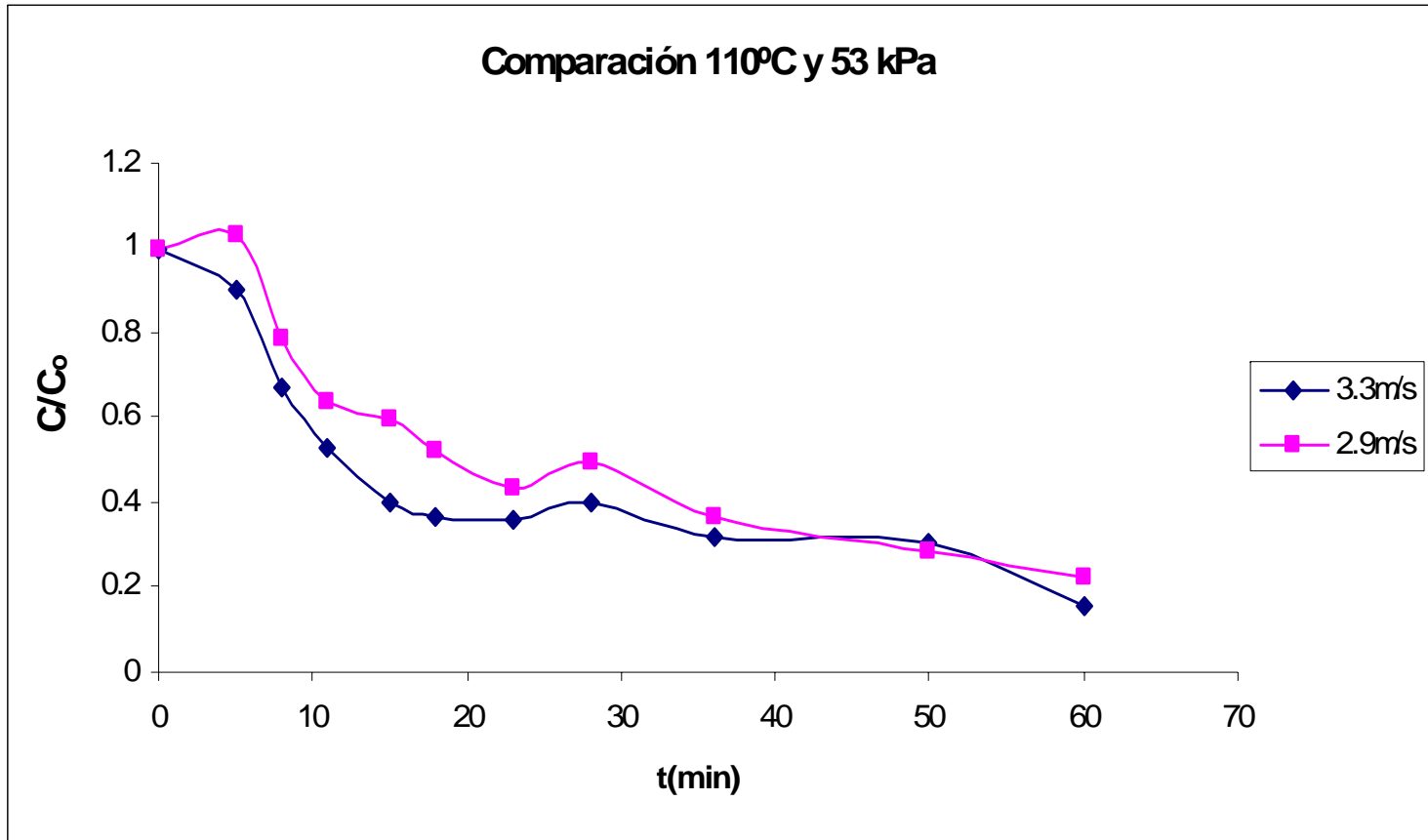
Figura C.85 Comparación de curvas normalizadas de secado.
