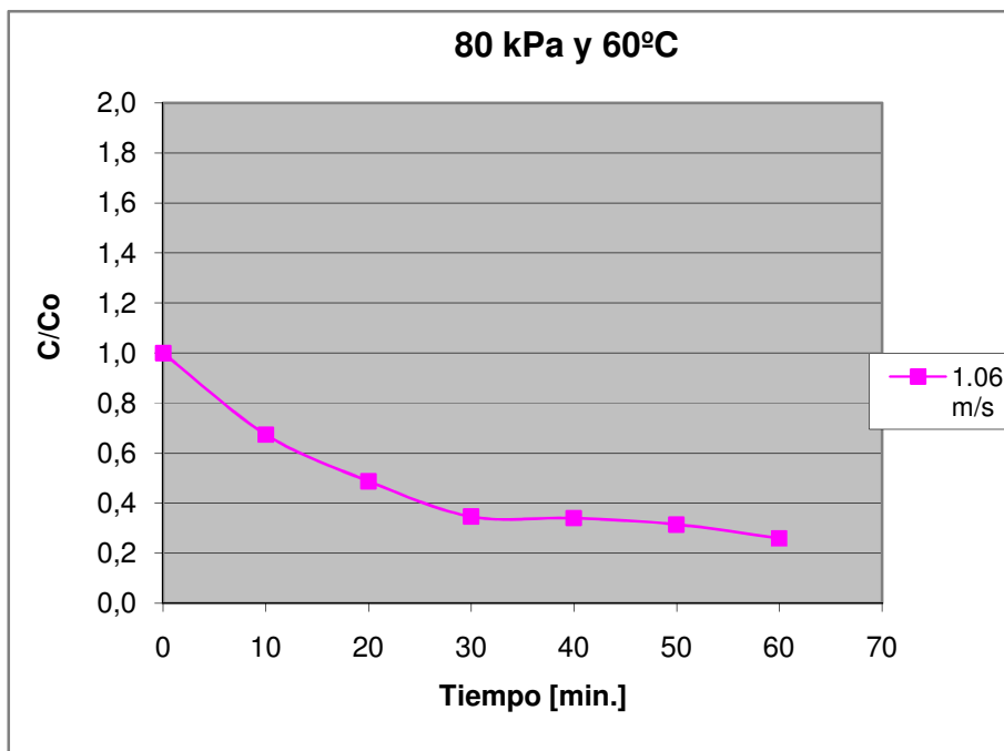
Figura D.24 Curva de secado de maíz crudo a 80 kPa y 60°C, 1.06 m/s
