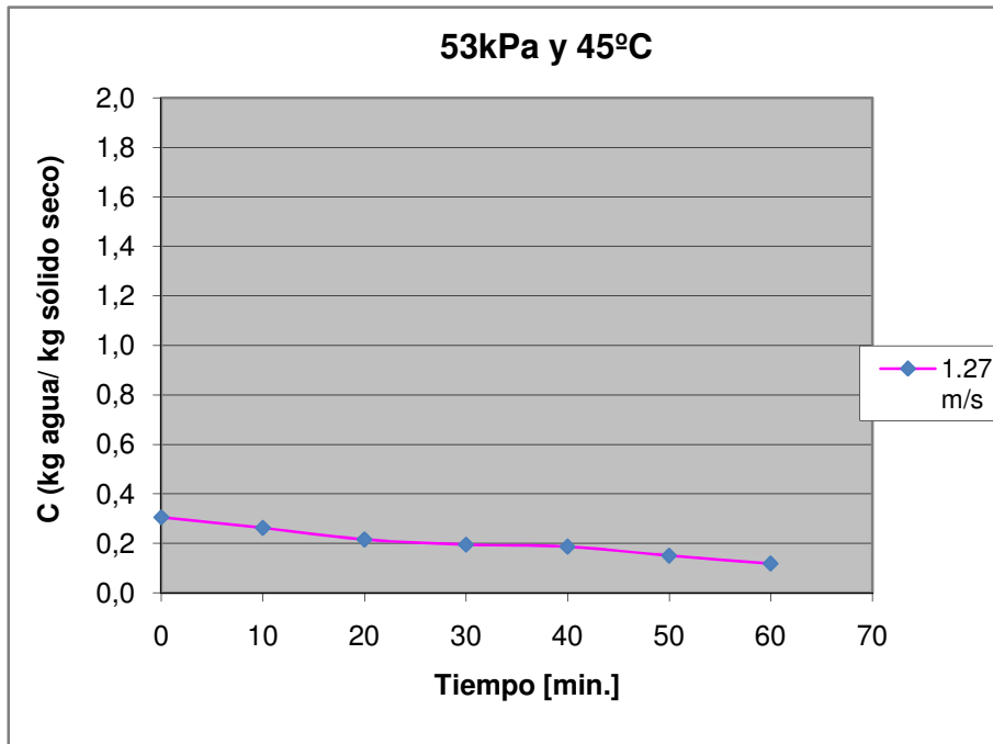
Figura D.15 Curva de secado de maíz crudo a 53 kPa y 45°C, 1.27 m/s
