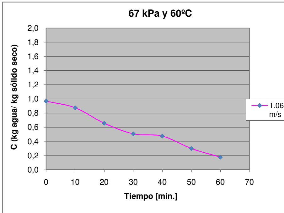
Figura D.29 Curva de secado de maíz crudo a 67 kPa y 60°C, 1.06 m/s
