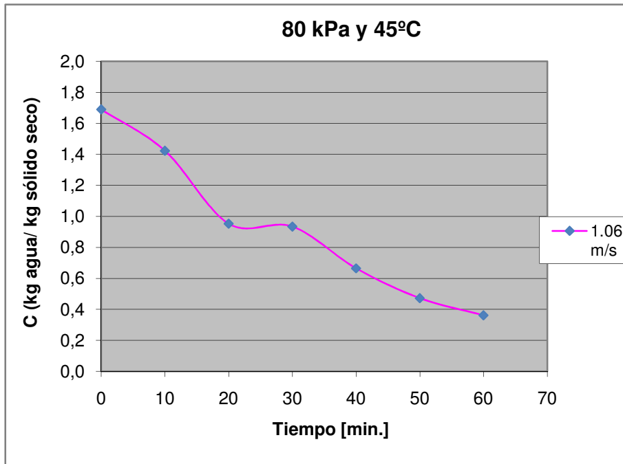
Figura D.21 Curva de secado de maíz crudo a 80 kPa y 45°C, 1.06 m/s
