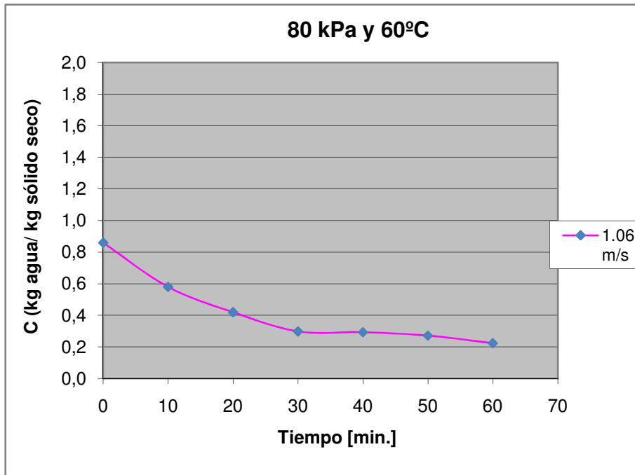
Figura D.23 Curva de secado de maíz crudo a 80 kPa y 60°C, 1.06 m/s
