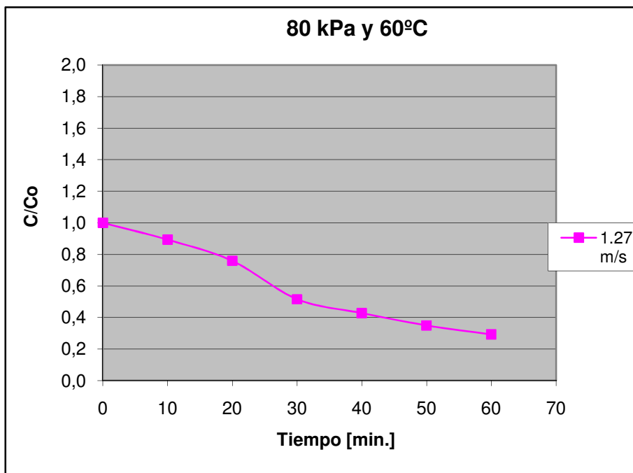
Figura D.6 Curva de secado de maíz crudo a 80 kPa y 60°C, 1.27 m/s
