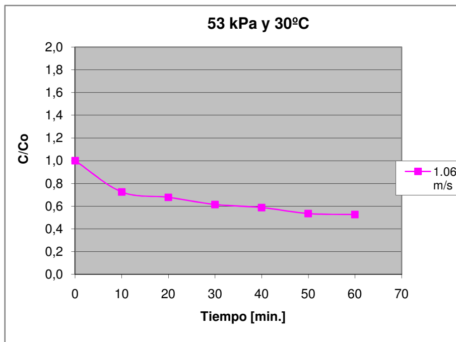
Figura D.32 Curva de secado de maíz crudo a 53 kPa y 30°C, 1.06 m/s
