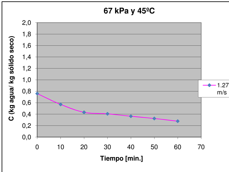
Figura D.9 Curva de secado de maíz crudo a 67kPa y 45°C, 1.27 m/s
