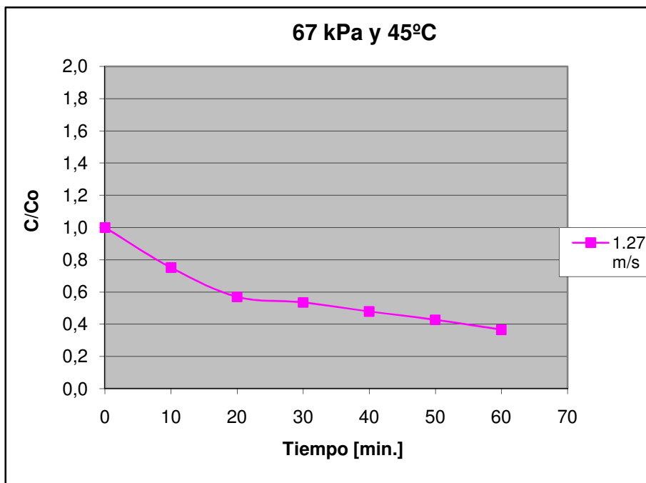
Figura D.10 Curva de secado de maíz crudo a 67 kPa y 45°C, 1.27 m/s
