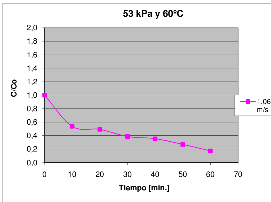
Figura D.36 Curva de secado de maíz crudo a 53 kPa y 60°C, 1.06 m/s
