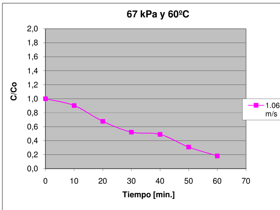
Figura D.30 Curva de secado de maíz crudo a 67 kPa y 60°C, 1.06 m/s
