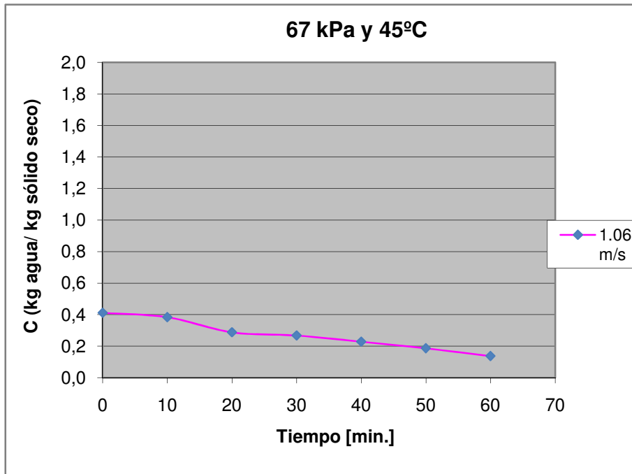
Figura D.27 Curva de secado de maíz crudo a 67 kPa y 45°C, 1.06 m/s
