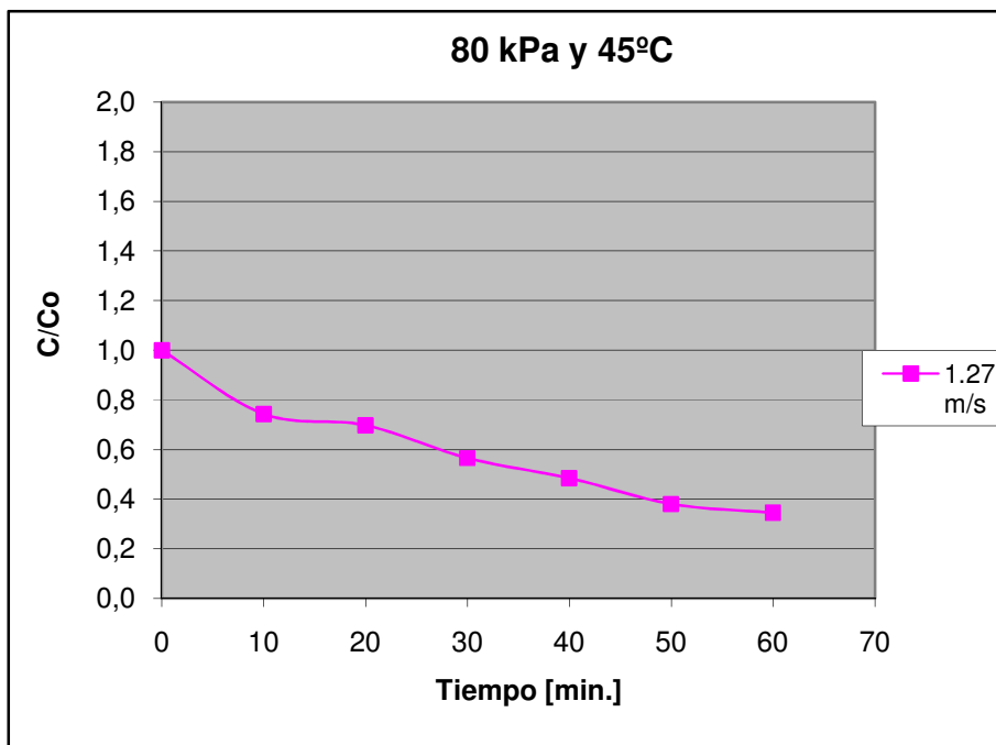
Figura D.4 Curva de secado de maíz crudo a 80 kPa y 45°C, 1.27 m/s
