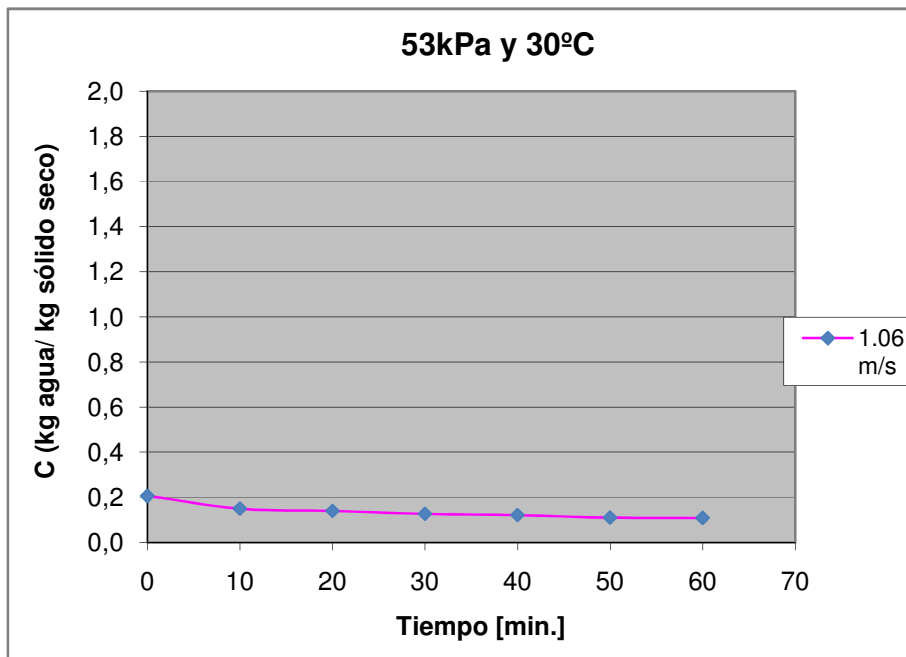
Figura D.31 Curva de secado de maíz crudo a 53 kPa y 30°C, 1.06 m/s
