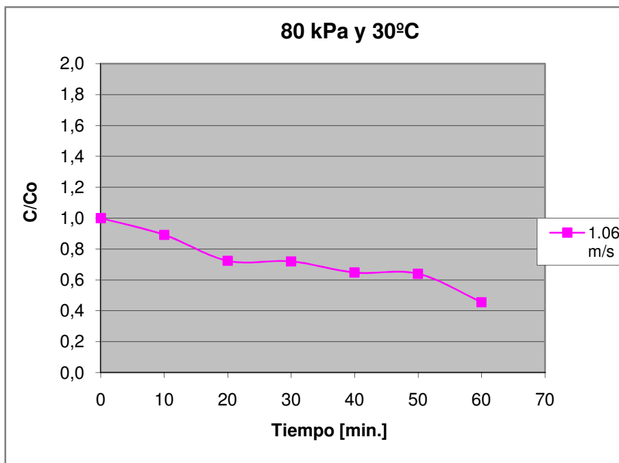
Figura D.20 Curva de secado de maíz crudo a 80 kPa y 30°C, 1.06 m/s
