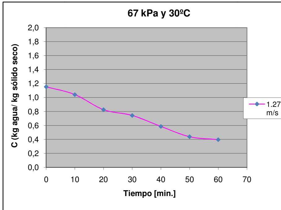
Figura D.7 Curva de secado de maíz crudo a 67kPa y 30°C, 1.27 m/s
