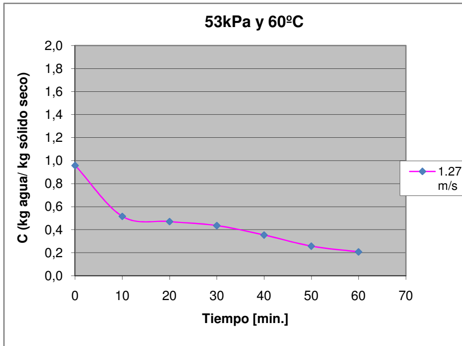
Figura D.17 Curva de secado de maíz crudo a 53 kPa y 60°C, 1.27 m/s
