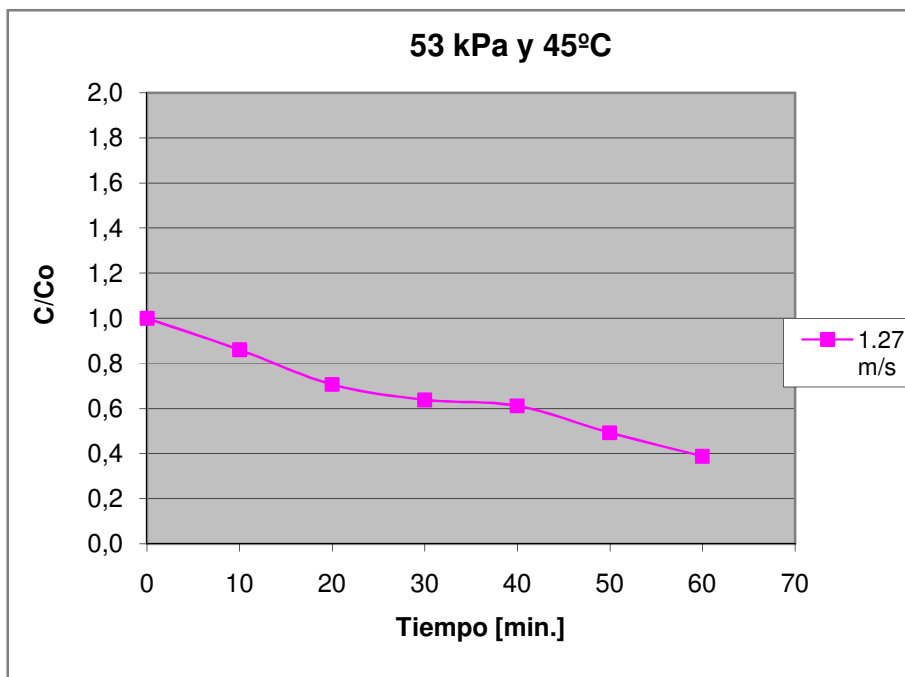
Figura D.16 Curva de secado de maíz crudo a 53 kPa y 45°C, 1.27 m/s
