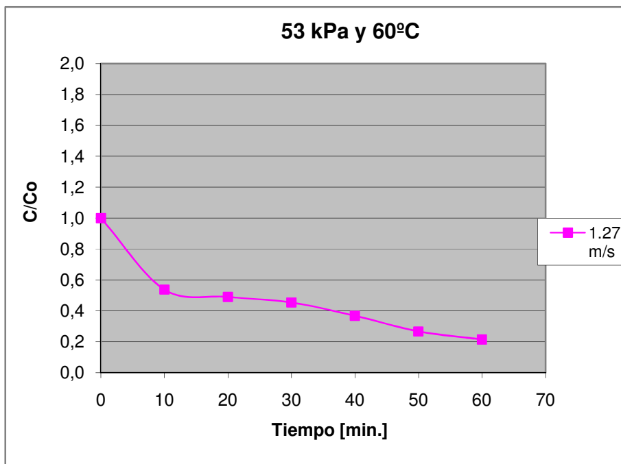
Figura D.18 Curva de secado de maíz crudo a 53 kPa y 60°C, 1.27 m/s
