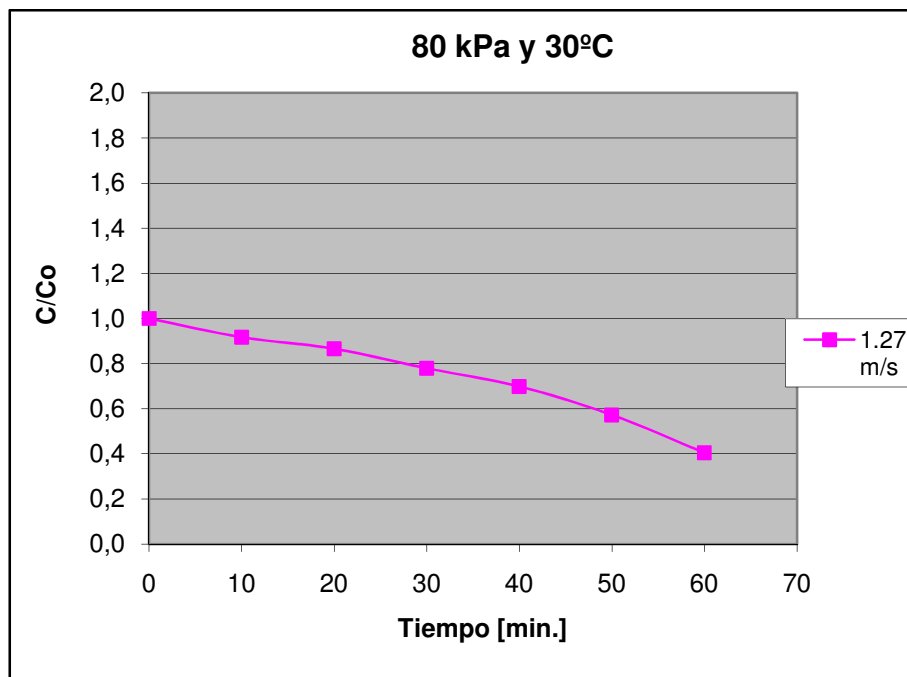
Figura D.2 Curva de secado de maíz crudo a 80 kPa y 30°C, 1.27 m/s
