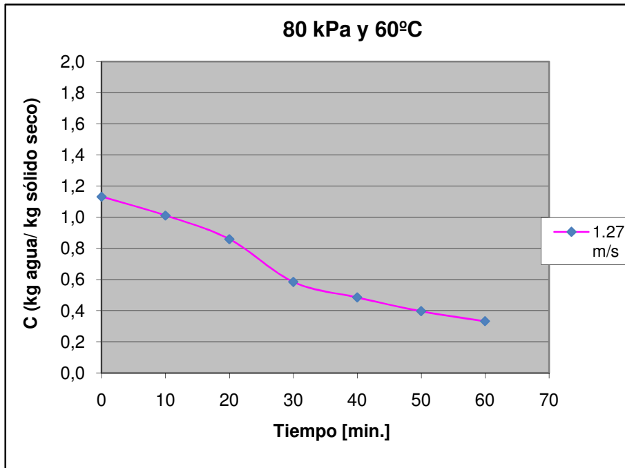
Figura D.5 Curva de secado de maíz crudo a 80 kPa y 60°C, 1.27 m/s
