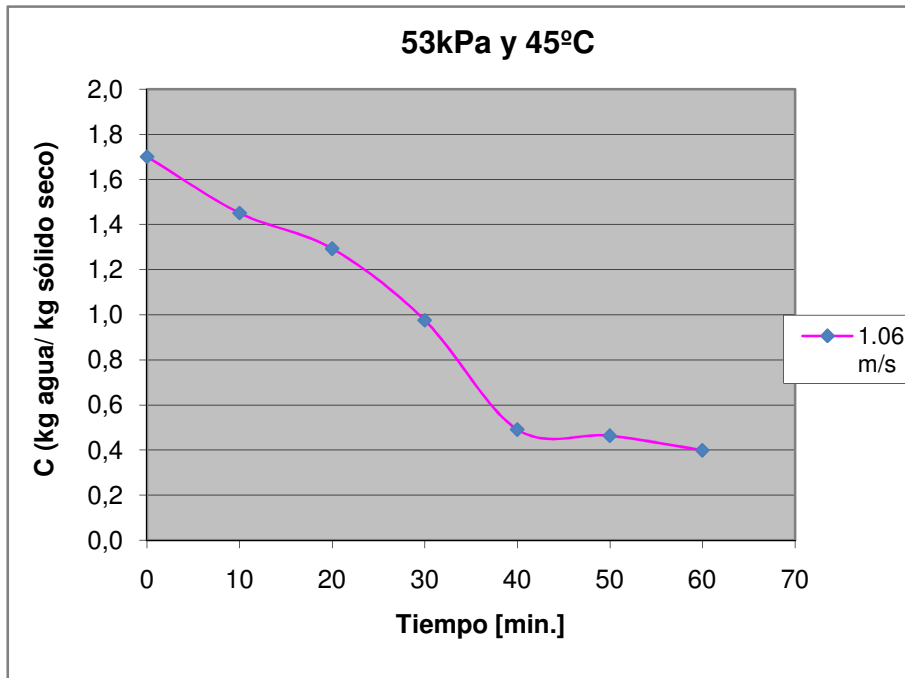
Figura D.33 Curva de secado de maíz crudo a 53 kPa y 45°C, 1.06 m/s
