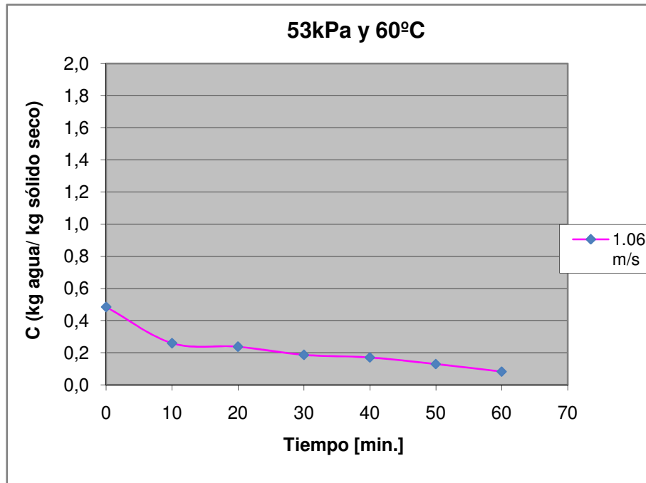
Figura D.35 Curva de secado de maíz crudo a 53 kPa y 60°C, 1.06 m/s
