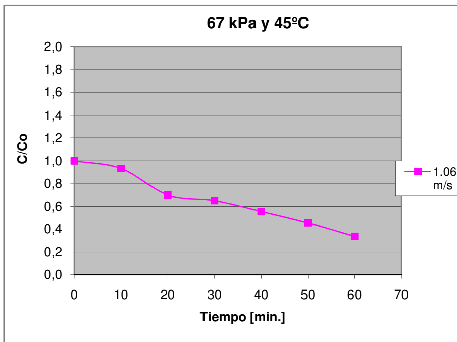
Figura D.28 Curva de secado de maíz crudo a 67 kPa y 45°C, 1.06 m/s
