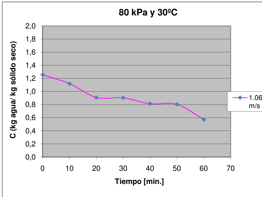
Figura D.19 Curva de secado de maíz crudo a 80 kPa y 30°C, 1.06 m/s
