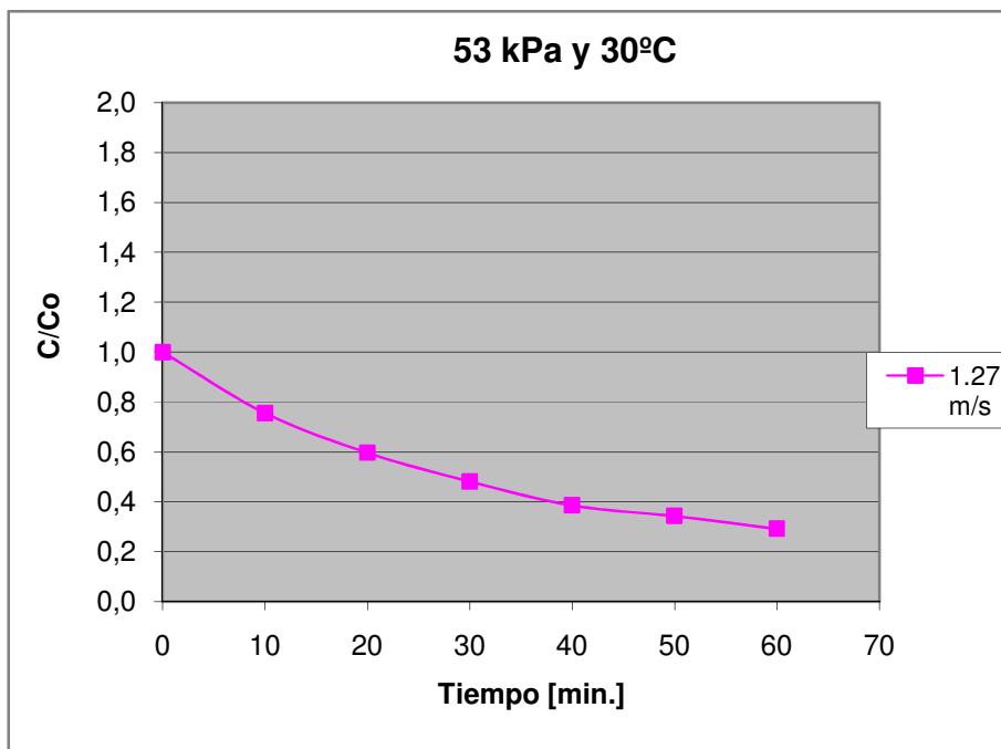
Figura D.14 Curva de secado de maíz crudo a 53 kPa y 30°C, 1.27 m/s
