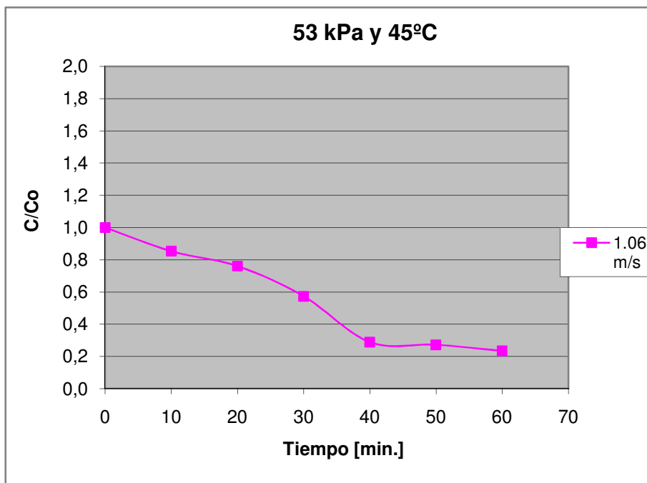
Figura D.34 Curva de secado de maíz crudo a 53 kPa y 45°C, 1.06 m/s
