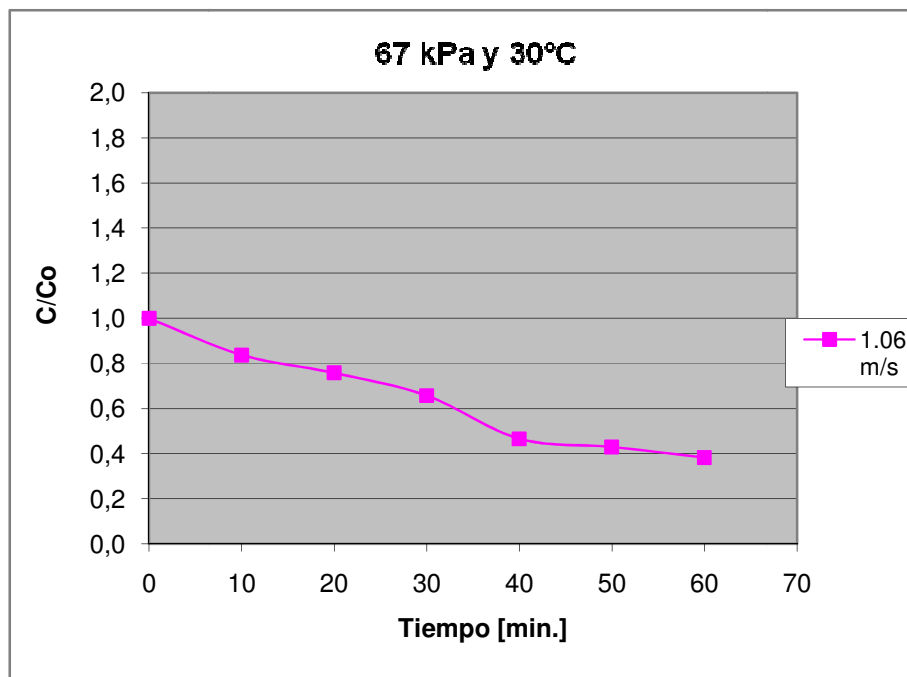
Figura D.26 Curva de secado de maíz crudo a 67 kPa y 30°C, 1.06 m/s
