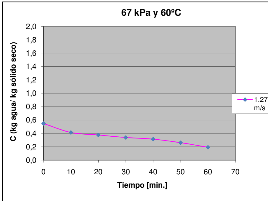
Figura D.11 Curva de secado de maíz crudo a 67kPa y 60°C, 1.27 m/s
