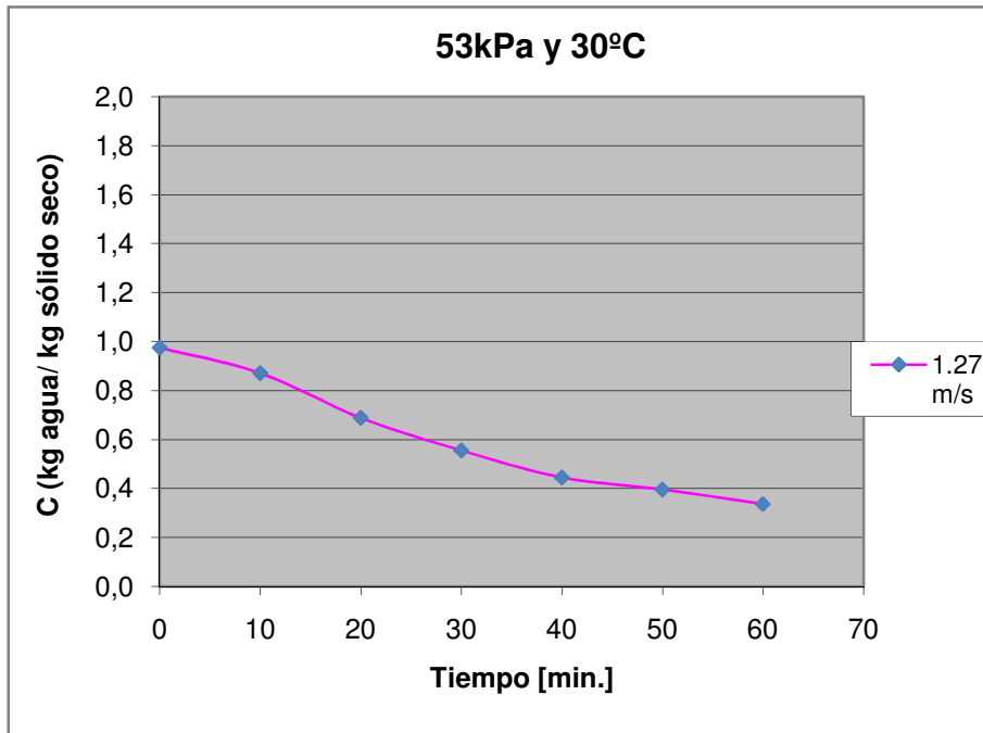
Figura D.13 Curva de secado de maíz crudo a 53 kPa y 30°C, 1.27 m/s
