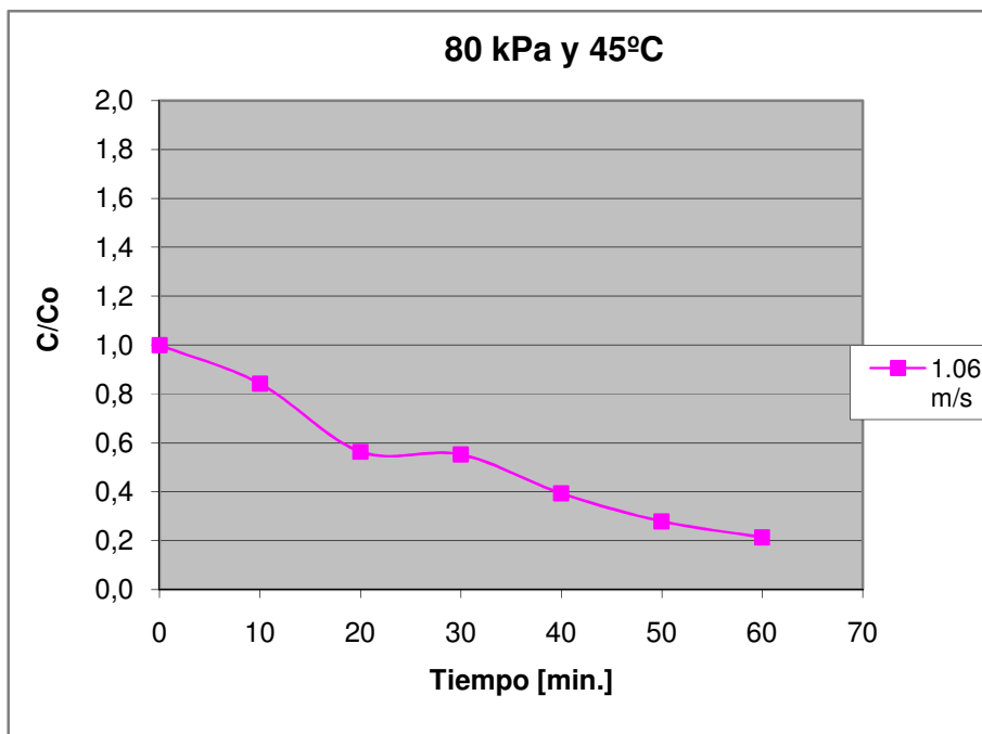
Figura D.22 Curva de secado de maíz crudo a 80 kPa y 45°C, 1.06 m/s
