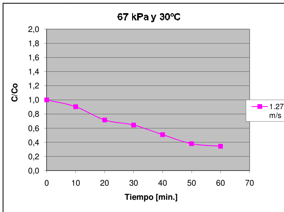
Figura D.8 Curva de secado de maíz crudo a 67 kPa y 30°C, 1.27 m/s
