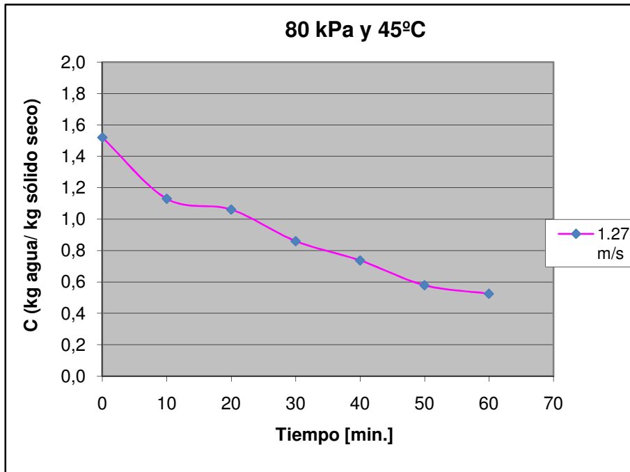
Figura D.3 Curva de secado de maíz crudo a 80 kPa y 45°C, 1.27 m/s
