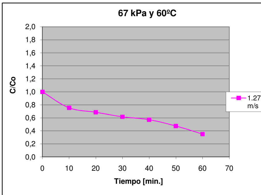
Figura D.12 Curva de secado de maíz crudo a 67 kPa y 60°C, 1.27 m/s
