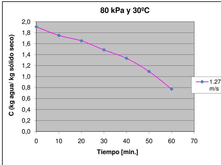
Figura D.1 Curva de secado de maíz crudo a 80 kPa y 30°C, 1.27 m/s
