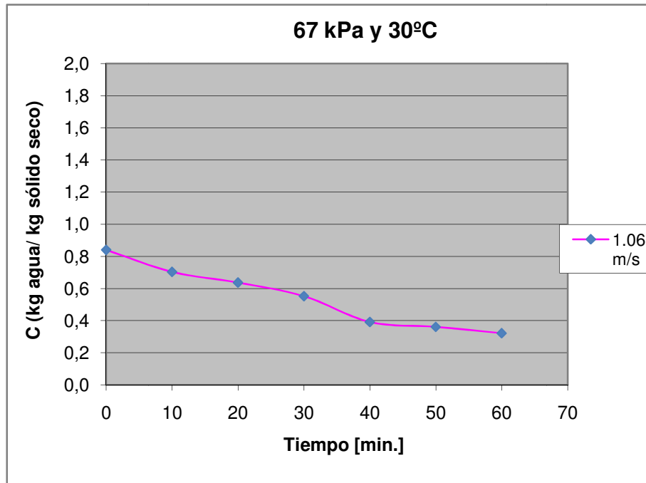
Figura D.25 Curva de secado de maíz crudo a 67 kPa y 30°C, 1.06 m/s
