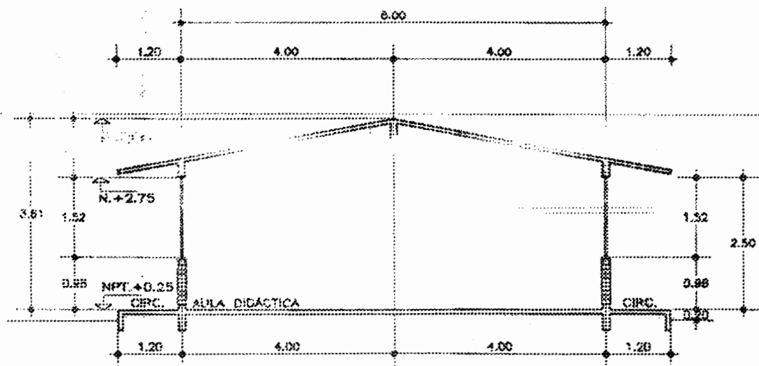
CORTE A-A'
