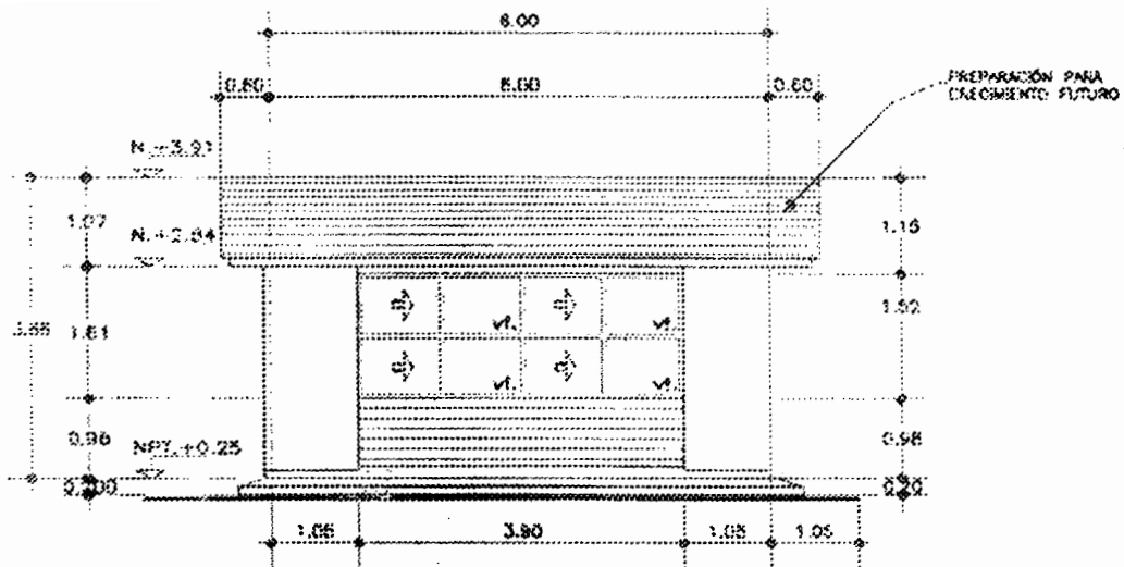
FACHADA POSTERIOR
