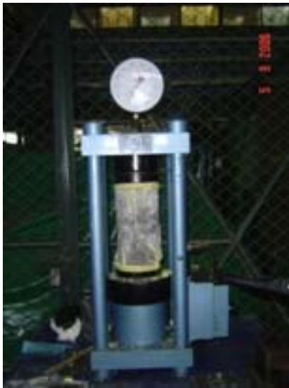
Figura J.7 Cilindro de madera a 28 días en prueba de compresión Elaboración propia
