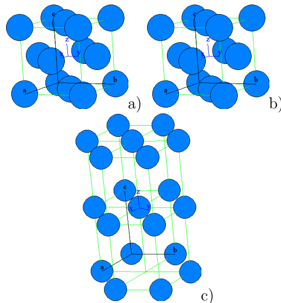
Figura B.1: Celda unitaria generadas con el programa Carine 3.1. a) Cúbica centrada en las caras del Cerio. b) Cúbica Centrada en el cuerpo del Europio. c) Hexagonal cerrada del Erblio.
