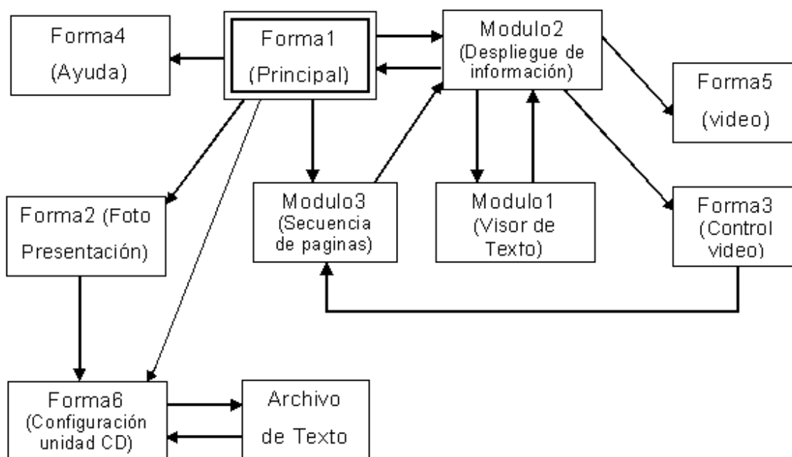
Figura B.1 Diagrama de flujo del programa.
