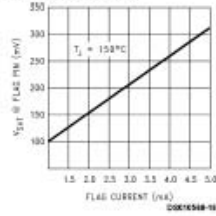
V DAT vs Flag Current
