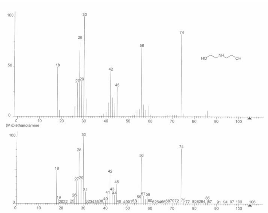
Figura J.5 Espectro característico de la DEA
