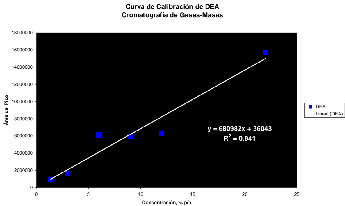
Figura J.11 Curva de Calibración de DEA (CG/M)
