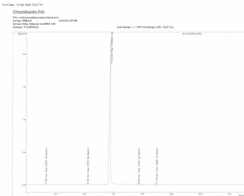
Figura J.7 Cromatograma de MDEA
