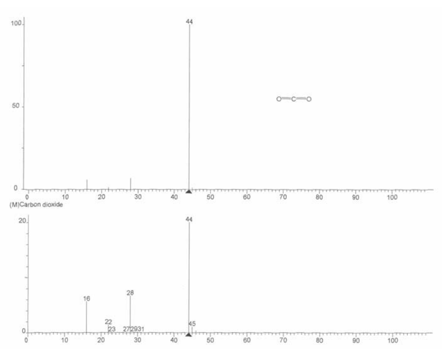
Figura J.6 Espectro característico del CO 2
