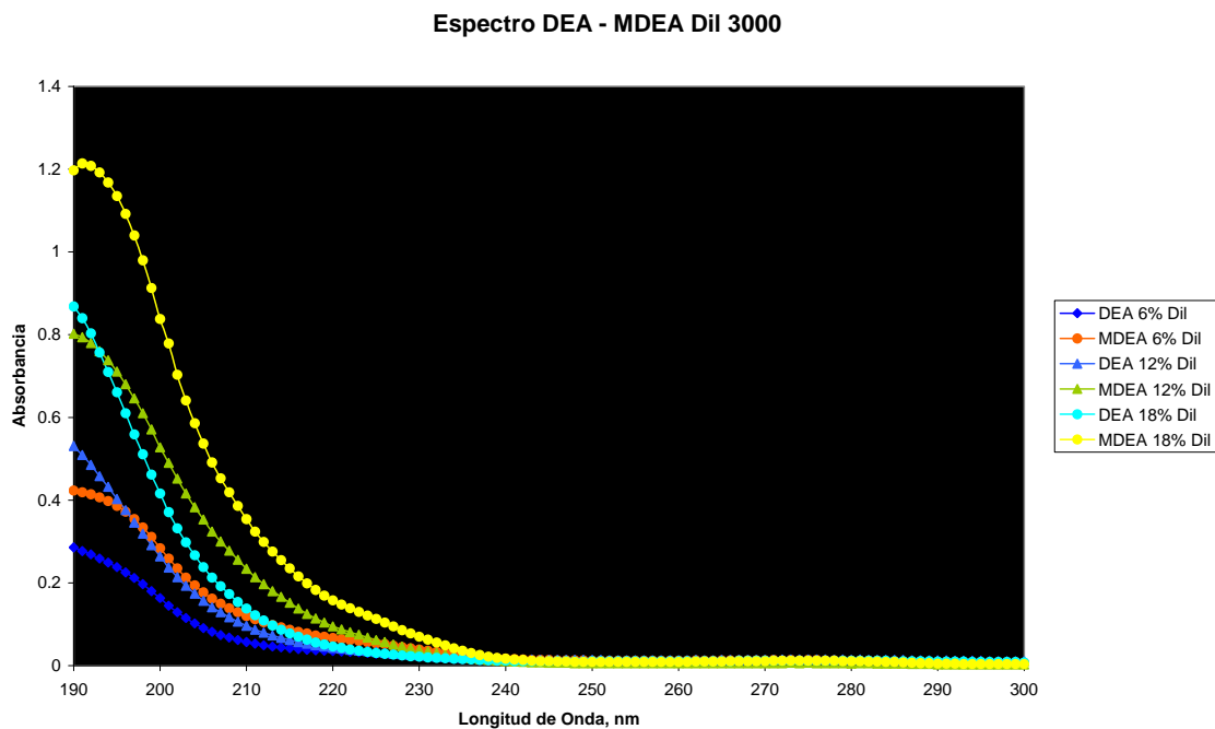
Figura H.4 Espectros DEA-MDEA diluidos
