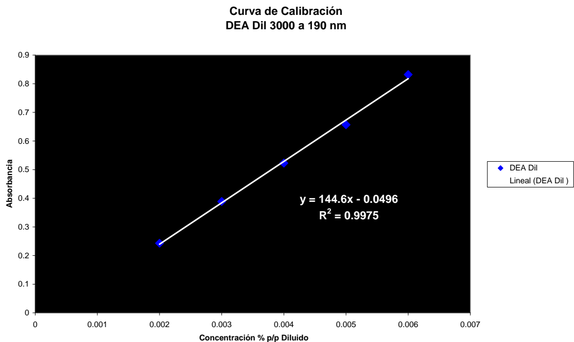
Figura H.5 Curva de calibración DEA (UV-Visible)
