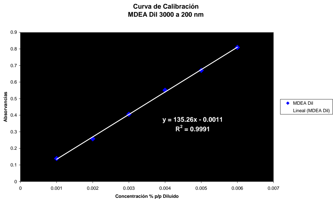
Figura H.6 Curva de calibración MDEA (UV-Visible)
