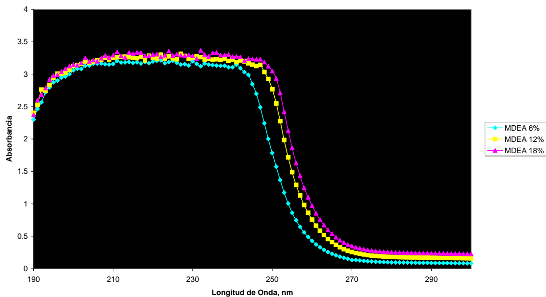
Espectros de MDEA
