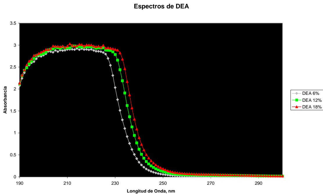
Figura H.3 Espectros de DEA
