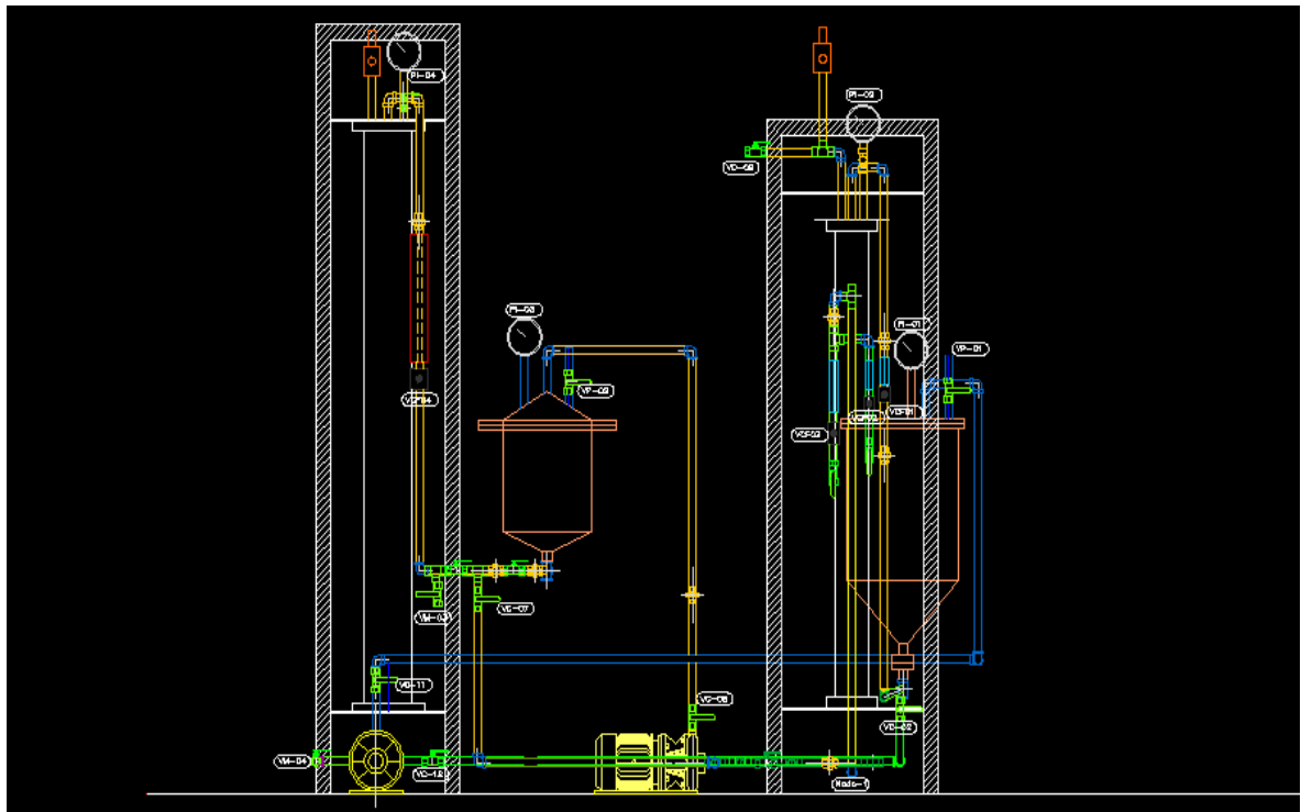
Figura A.1 Diagrama en AutoCad de la planta piloto
