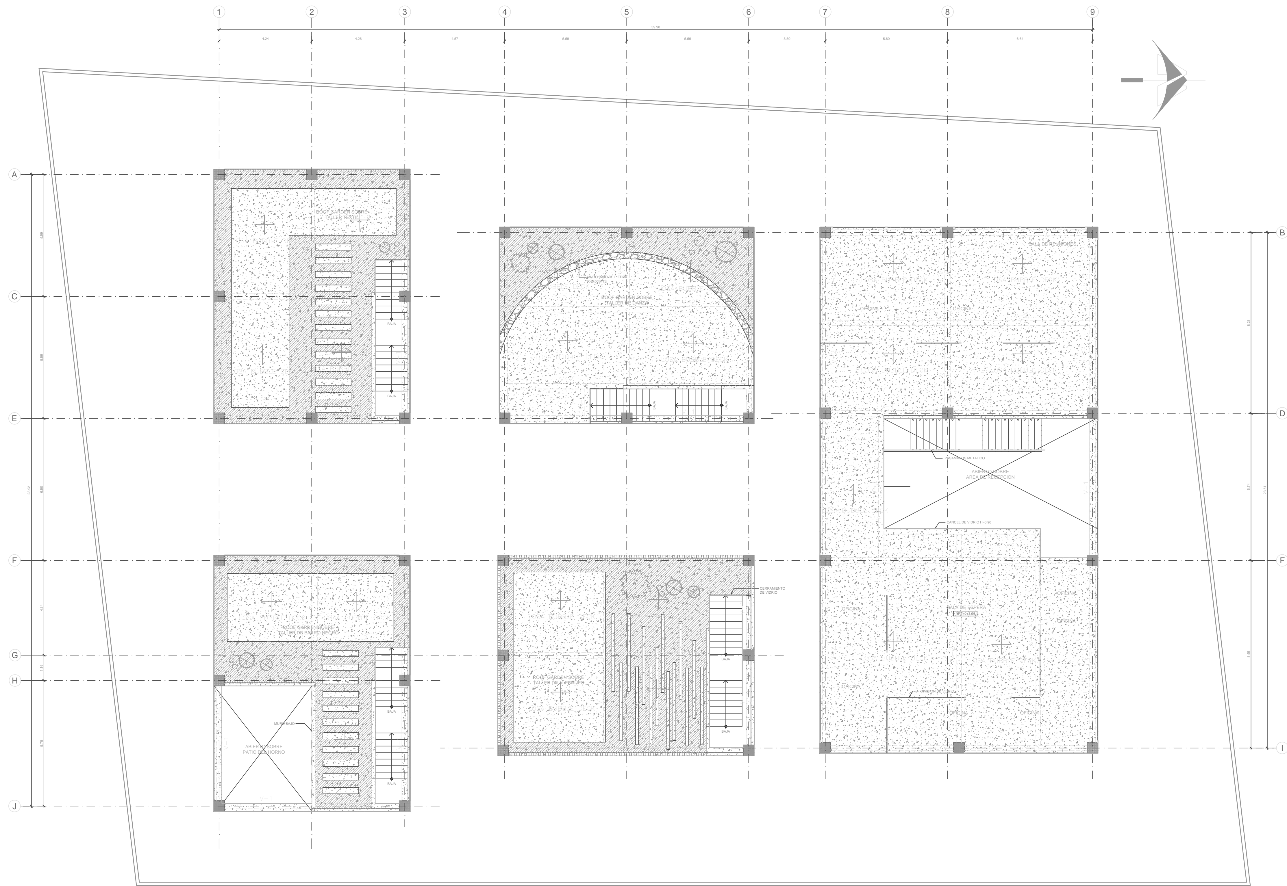
PLANTA ESTRUCTURAL NIVEL 2 (N=0+3.20)
