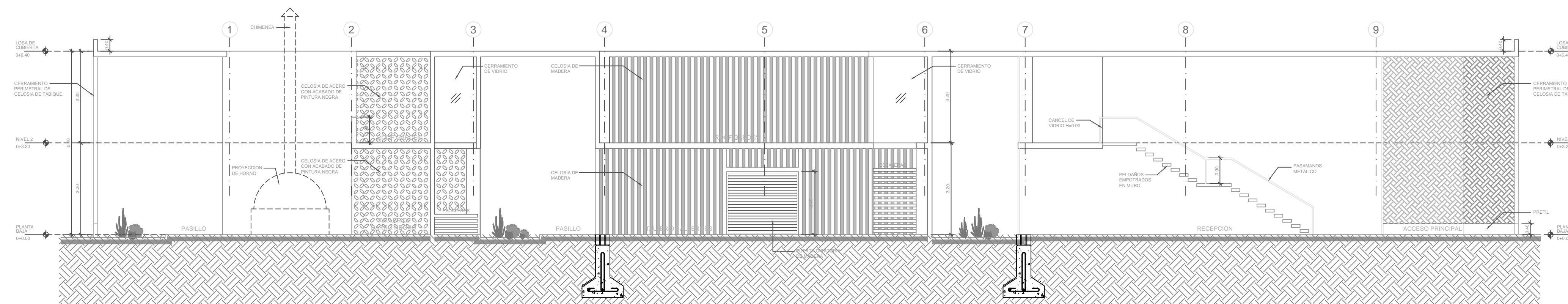
1 CORTE LONGITUDINAL
