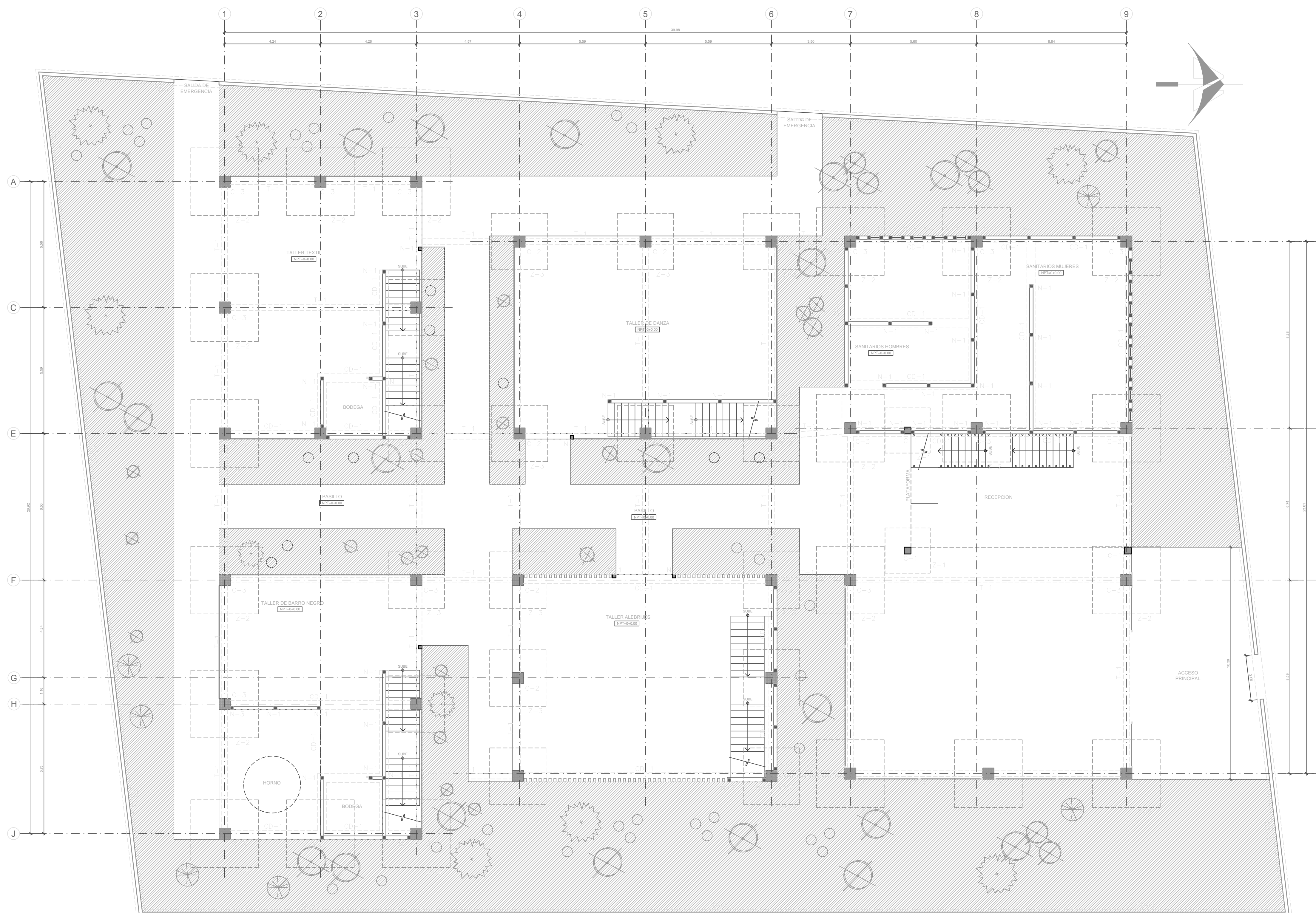
PLANTA ESTRUCTURAL DE FUNDACIONES (N=0+0.00) ESCALA 1: 100
